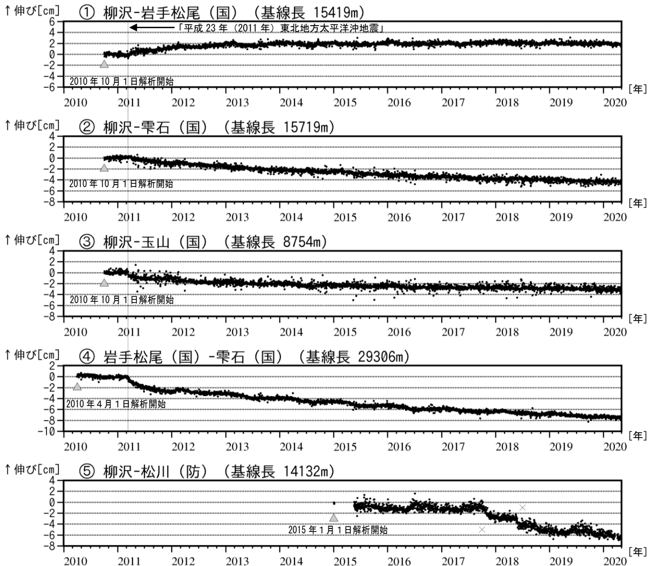
図5 岩手山 GNSS 基線長変化図（2010年4月～2020年4月）
