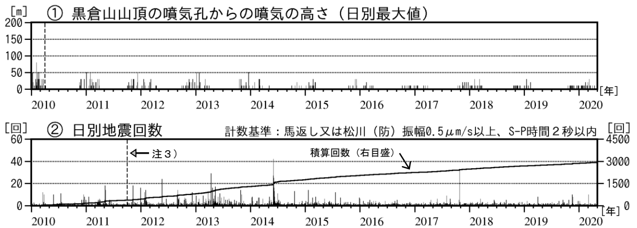
図4 岩手山 噴気の高さ及び日別地震回数（2010年1月～2020年4月）
