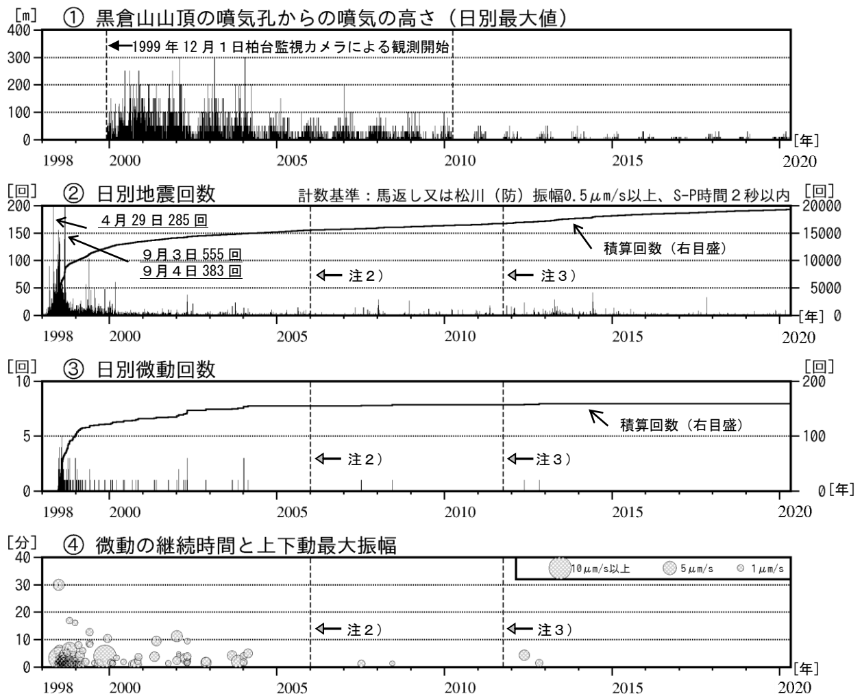
図3 岩手山 火山活動経過図（1998年1月～2020年4月）
