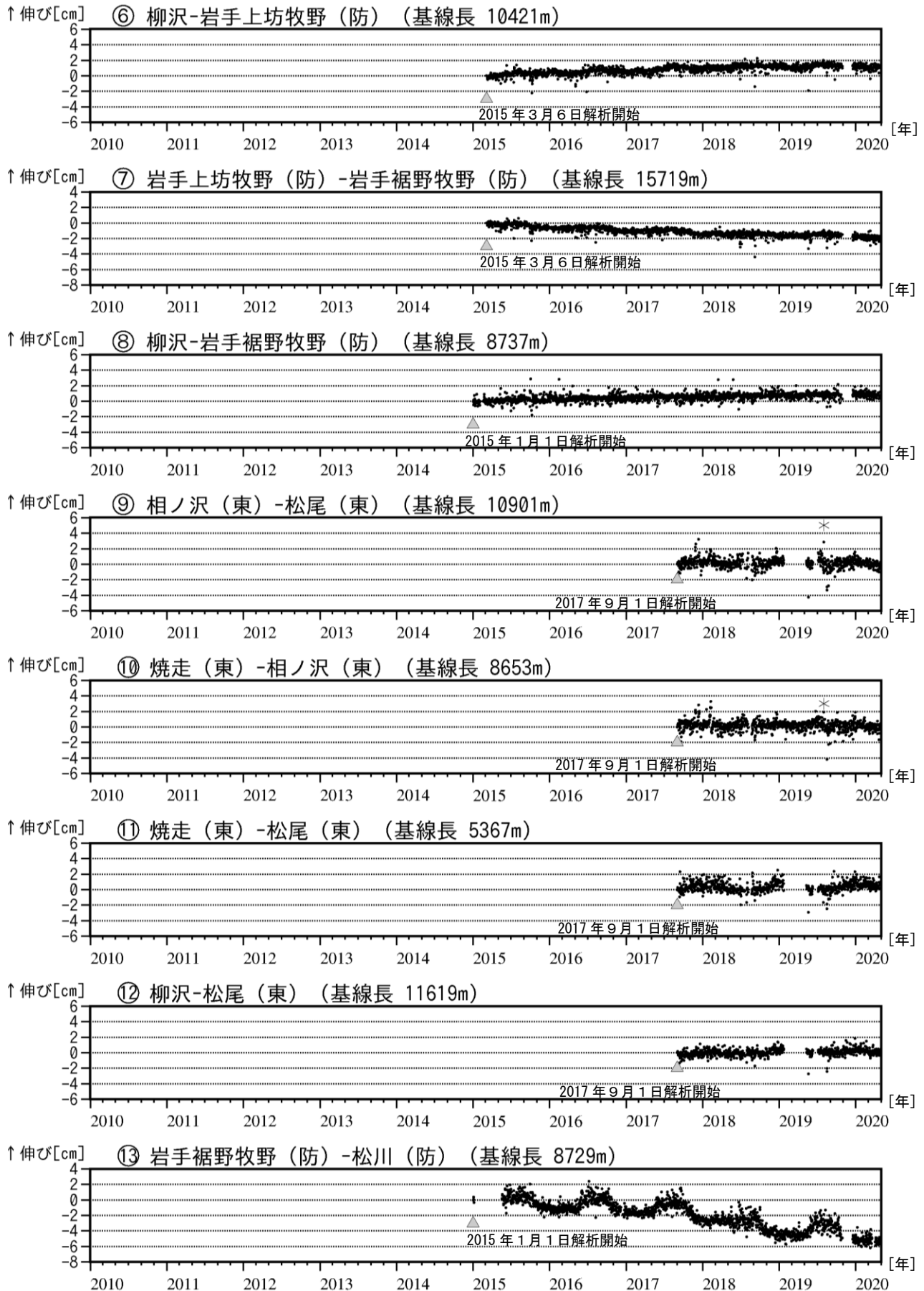
図6 岩手山 GNSS 基線長変化図（2015年1月～2020年4月）
