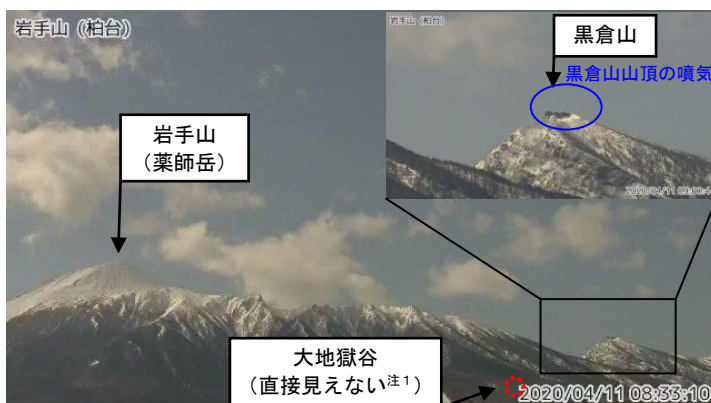
図1 岩手山 黒倉山の噴気の状況（4月11日）
