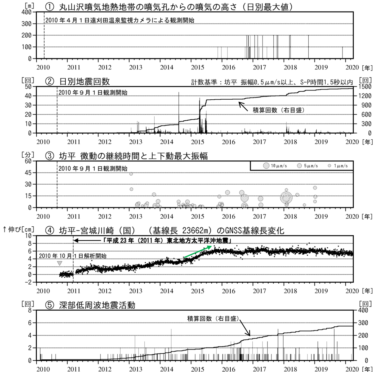
図2 蔵王山 火山活動経過図（2010年4月～2020年3月）
