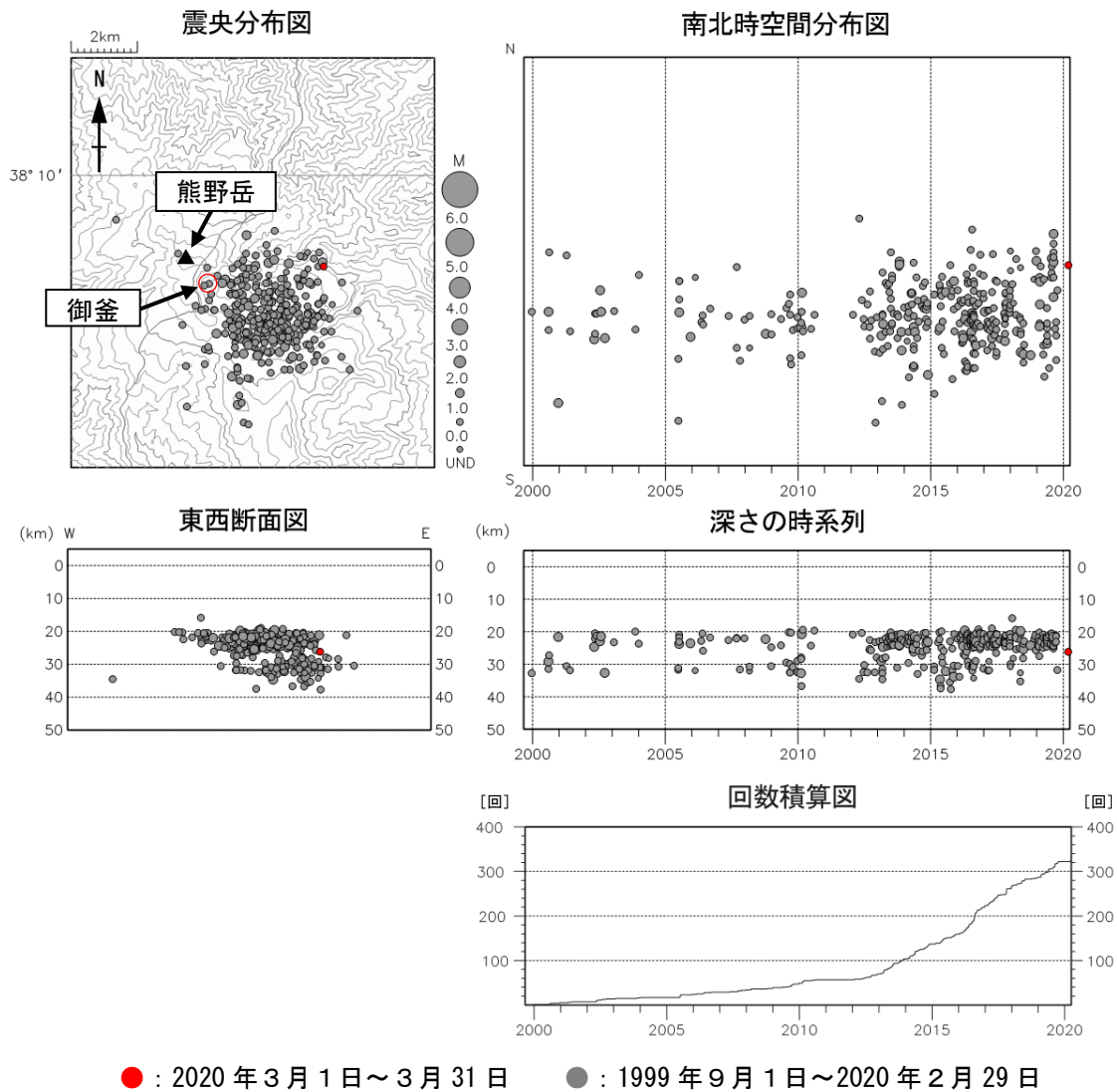
図3 蔵王山 広域地震観測網による深部低周波地震活動（1999年9月～2020年3月）
