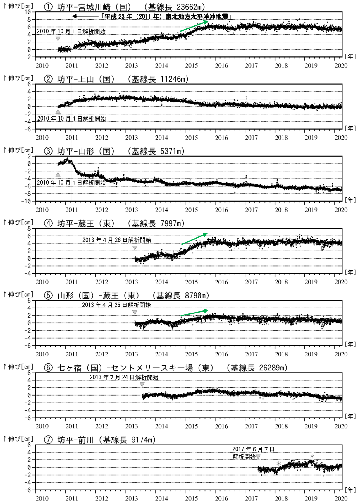
図4 蔵王山 GNSS 基線長変化図（2010年10月～2020年3月）
