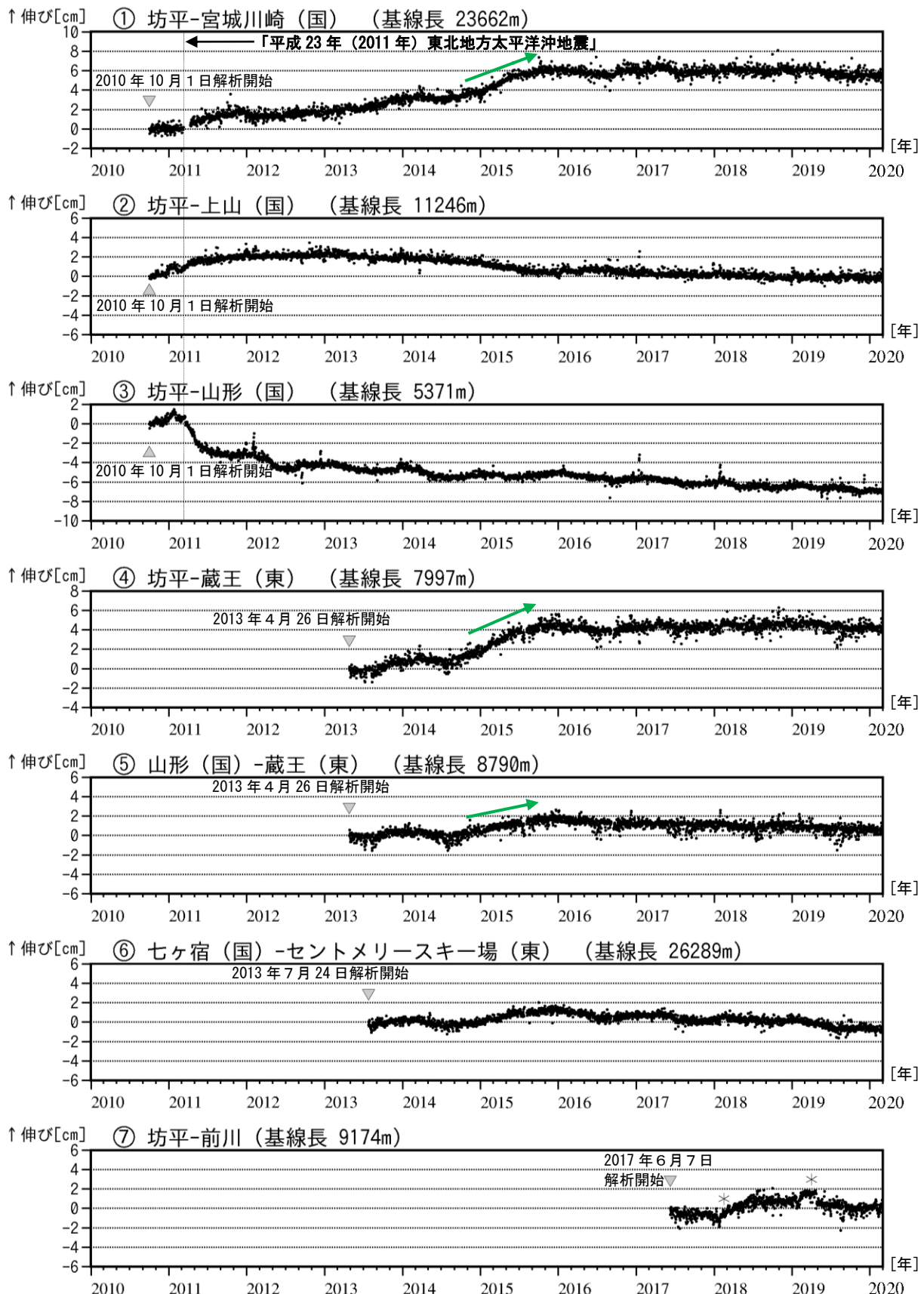
図7 蔵王山 GNSS 基線長変化図 (2010年10月～2020年2月)
