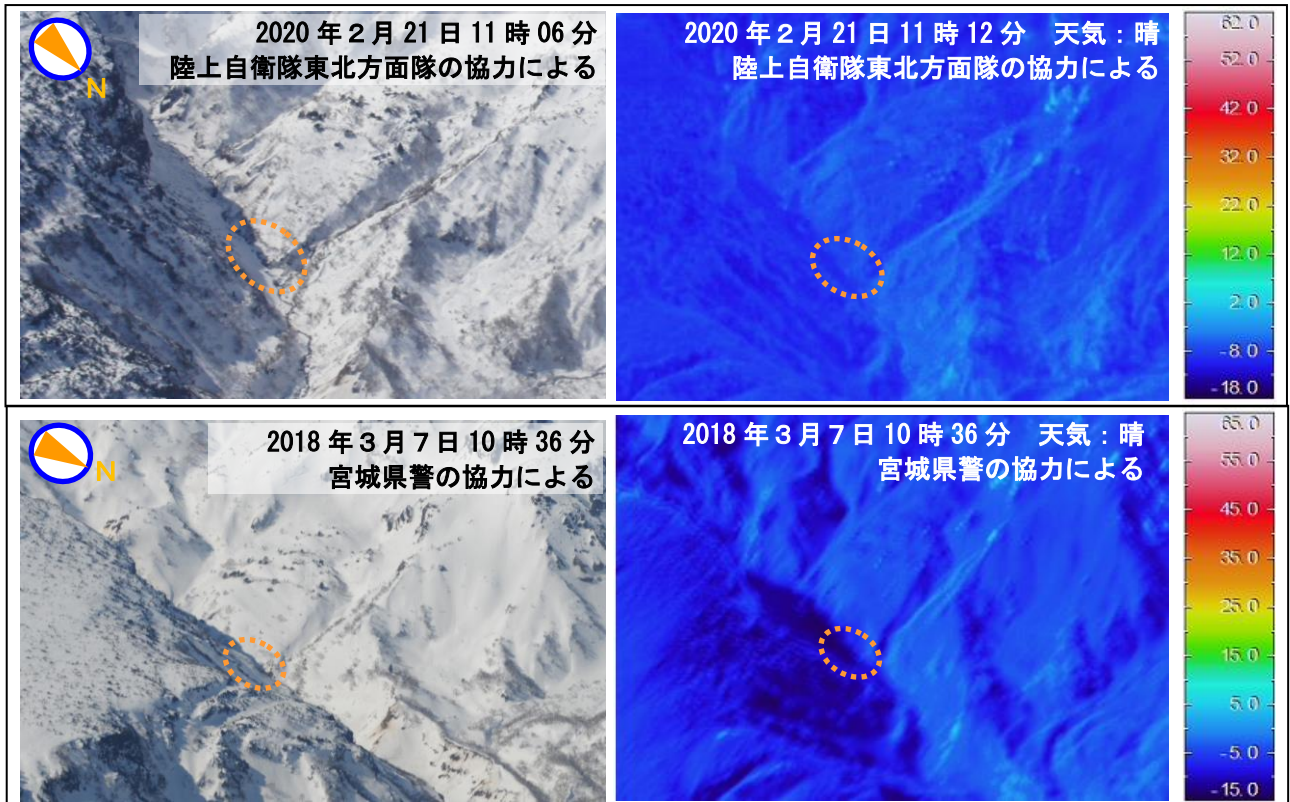
図4 蔵王山 上空から撮影した振子沢付近の状況と地表面温度分布
