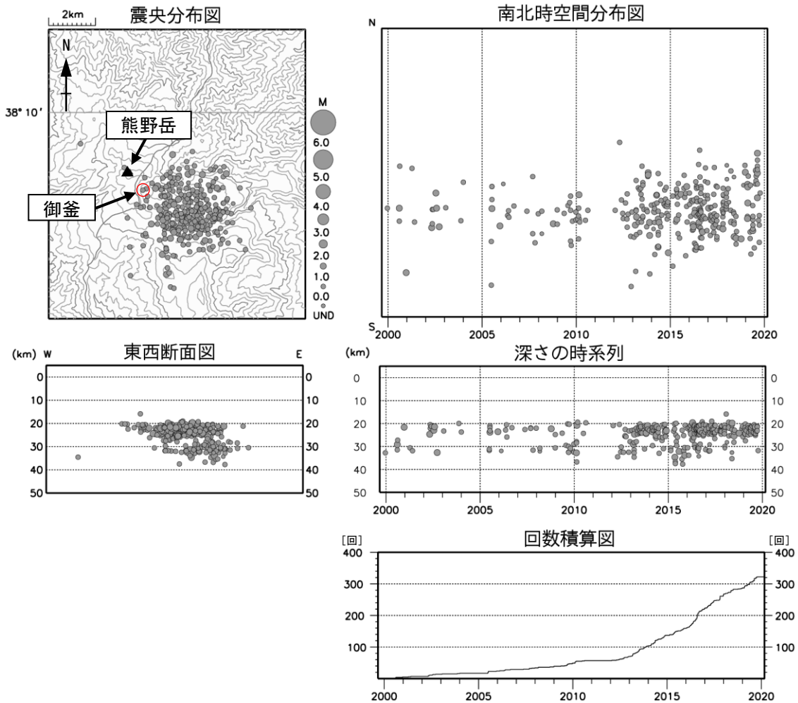
図 6 蔵王山 広域地震観測網による深部低周波地震活動（1999 年 9 月～2020 年 2 月）
