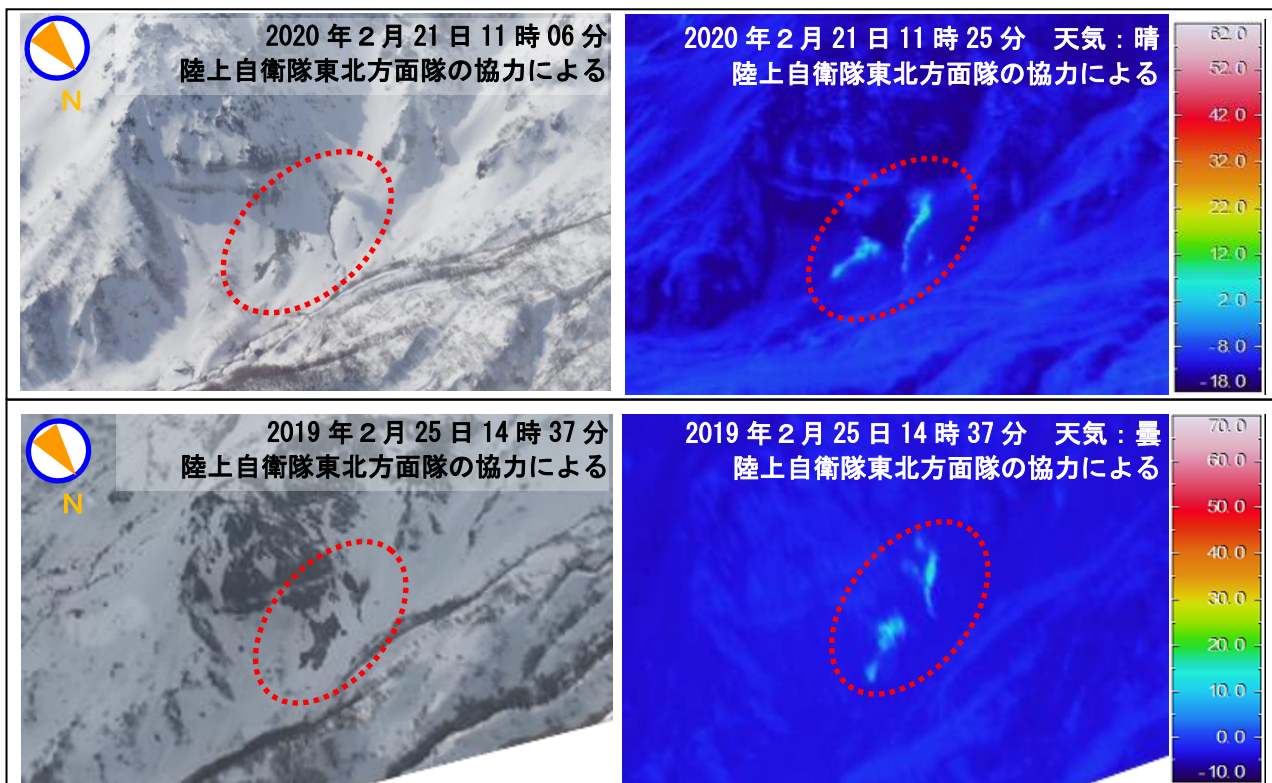
図3 蔵王山 上空から撮影した丸山沢噴気地熱地帯の状況と地表面温度分布
