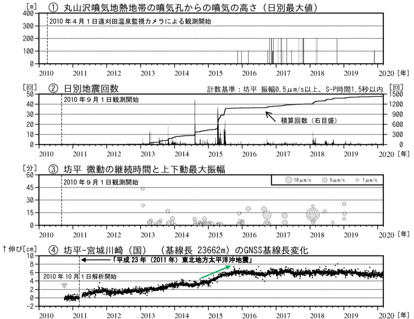
図5 蔵王山 火山活動経過図（2010年4月～2020年2月）
