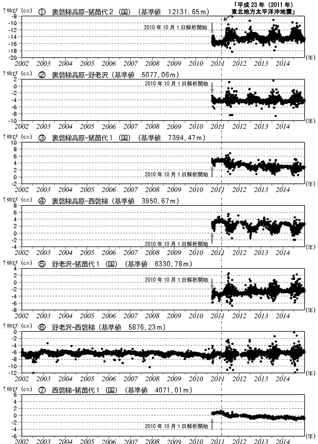
図 7 磐梯山 GNSS 2) 基線長変化図 (2002 年 1 月～2014 年 12 月)
