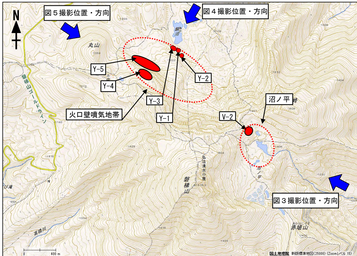
図 2 磐梯山 噴気と地熱域の分布及び上空からの写真と地表面温度分布 1) の撮影位置・方向
