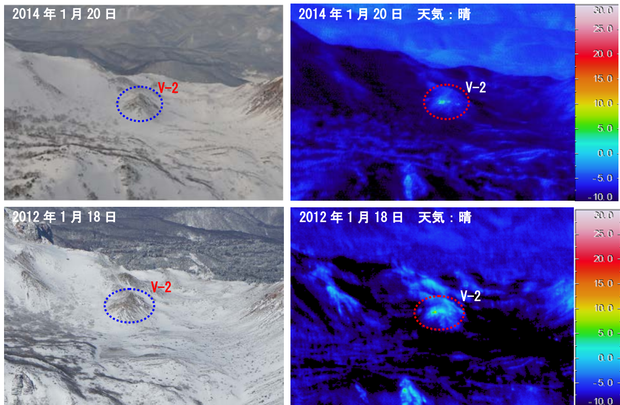
図 3 磐梯山 南東方向から撮影した沼ノ平 (V-2) の状況 (左) と地表面温度分布 (右) ・ 2012 年 1 月 18 日と比較して、地熱域に特段の変化は認められませんでした。
