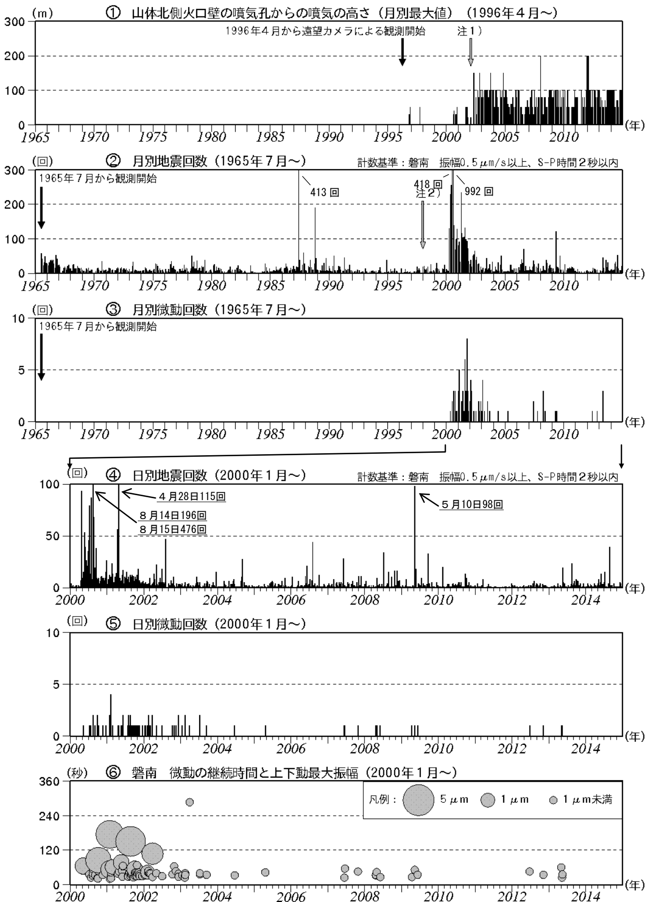
図6 磐梯山 火山活動経過図（1965年7月～2014年12月）
