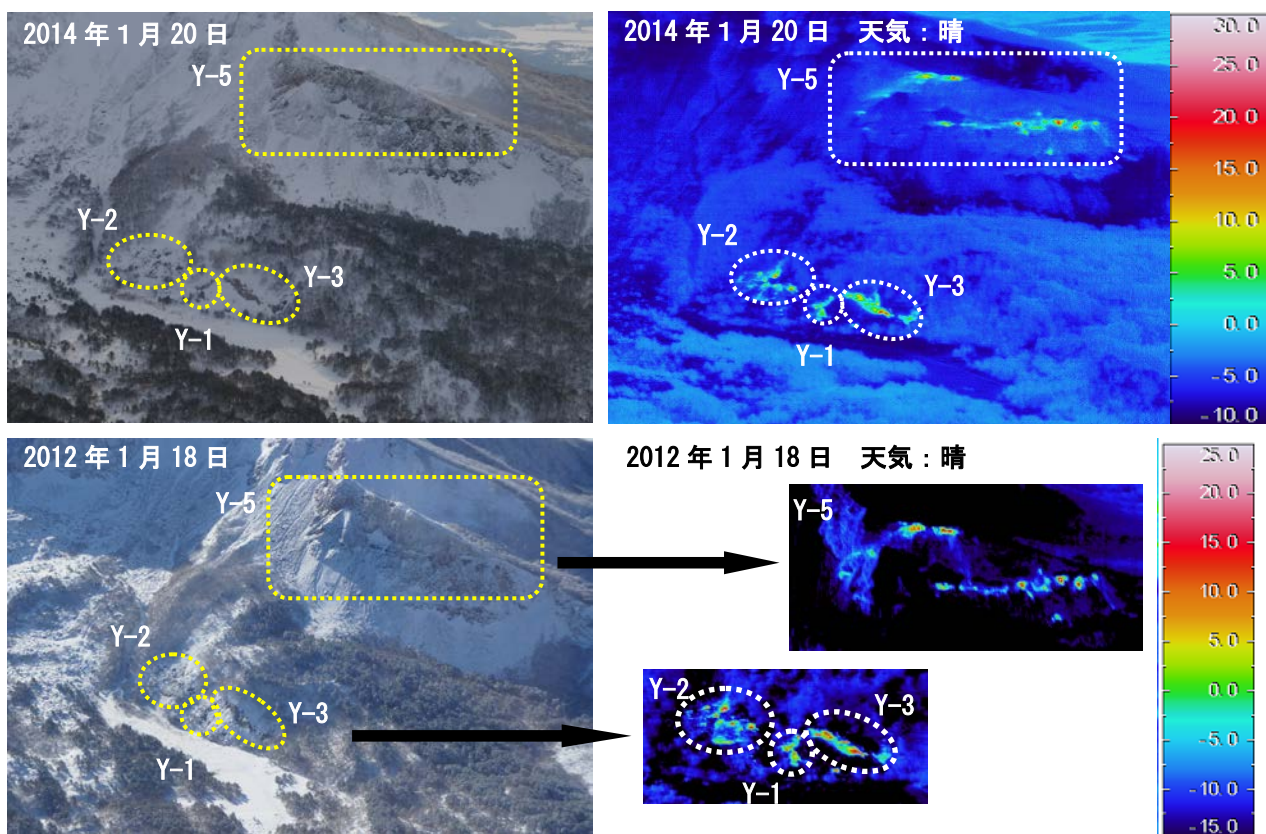
図 4 磐梯山 北東方向から撮影した火口壁噴気地帯（Y-1、2、3、5）の状況（左）と地表面温度分布（右）
