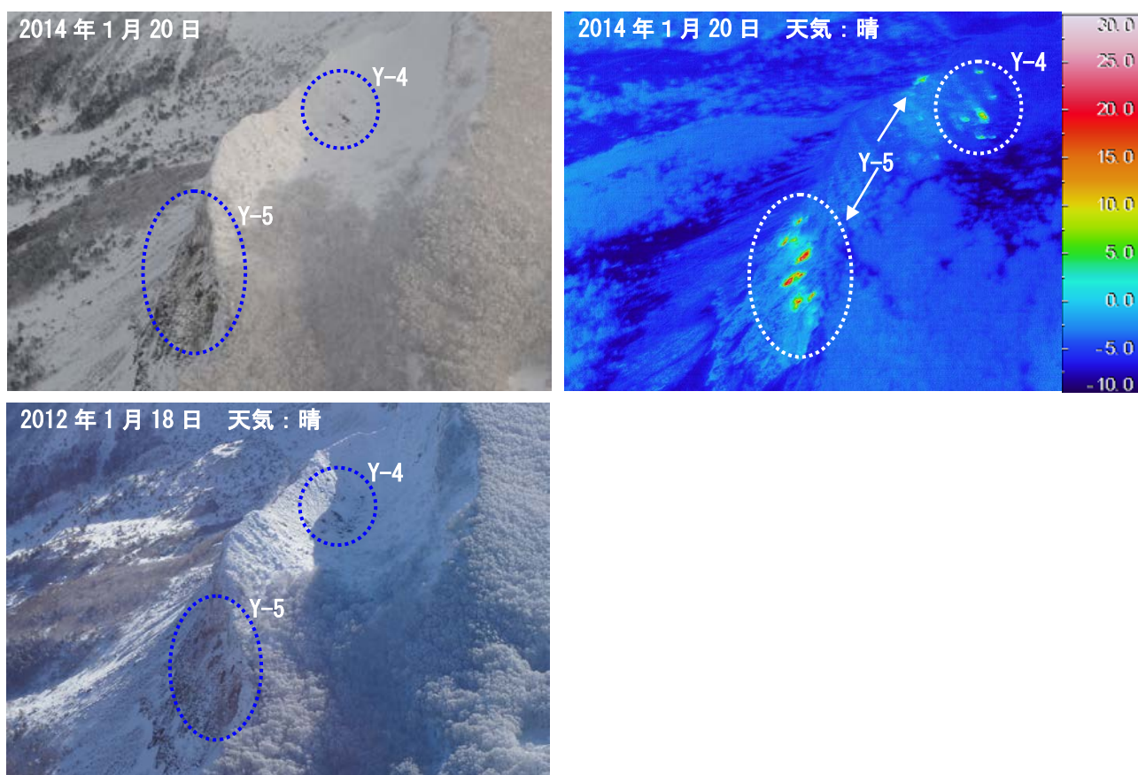
図 5 磐梯山 北西方向から撮影した火口壁噴気地帯（Y-4、5）の状況（左）と地表面温度分布（右）
