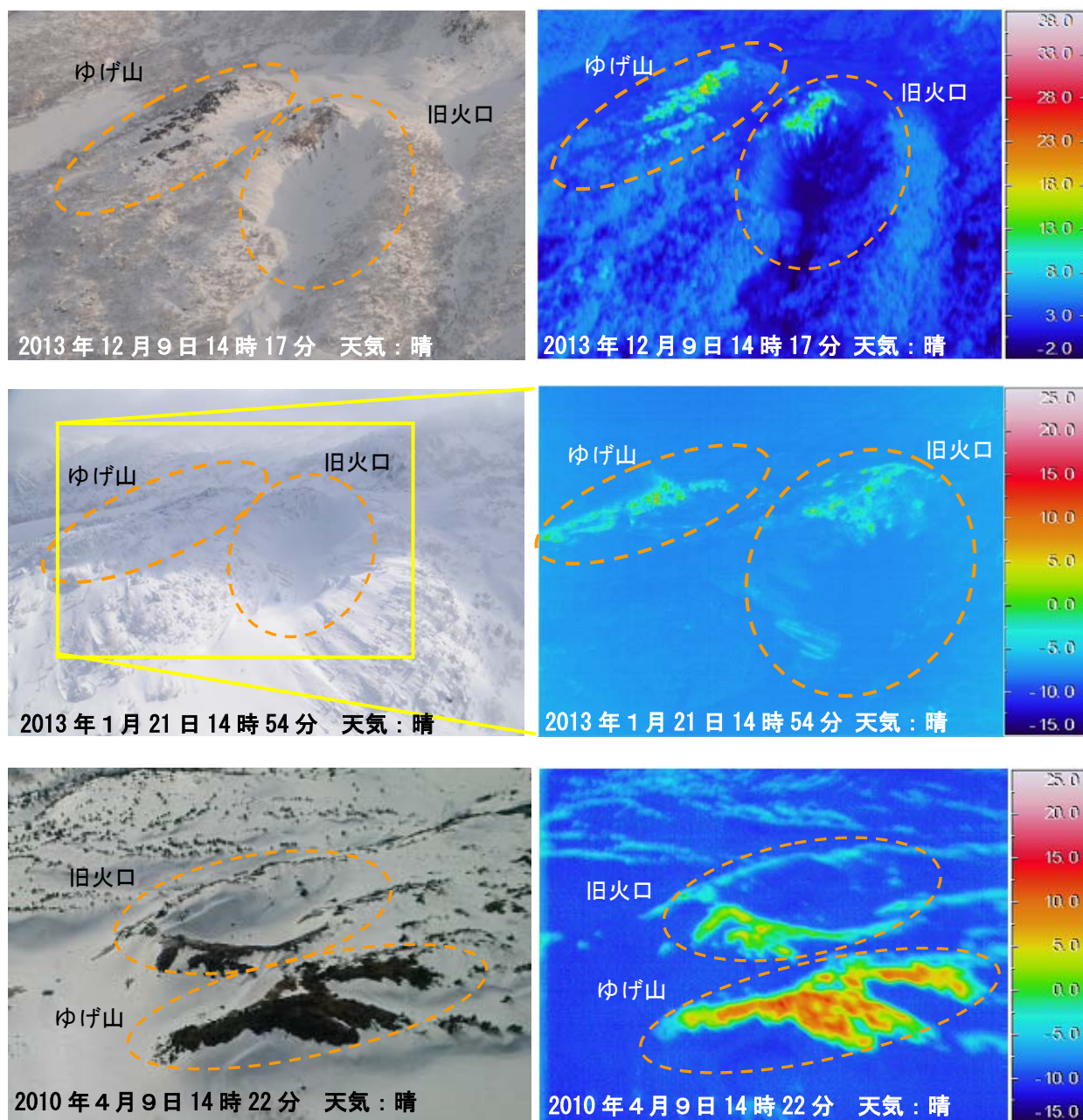
図5 栗駒山 ゆげ山、旧火口付近の可視画像（左）と地表面温度分布 1) （右）
