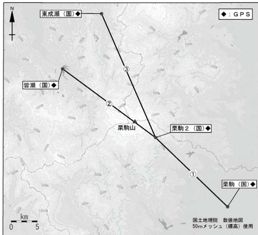
図 9 栗駒山 GPS 観測点配置図
