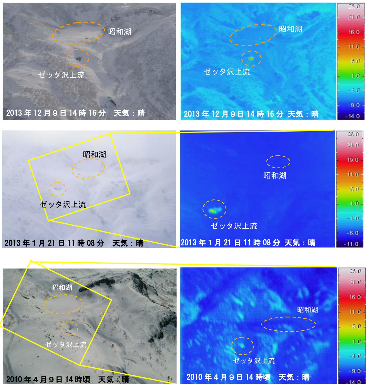
図6 栗駒山 ゼッタ沢上流、昭和湖付近の可視画像（左）と地表面温度分布 1) （右）
