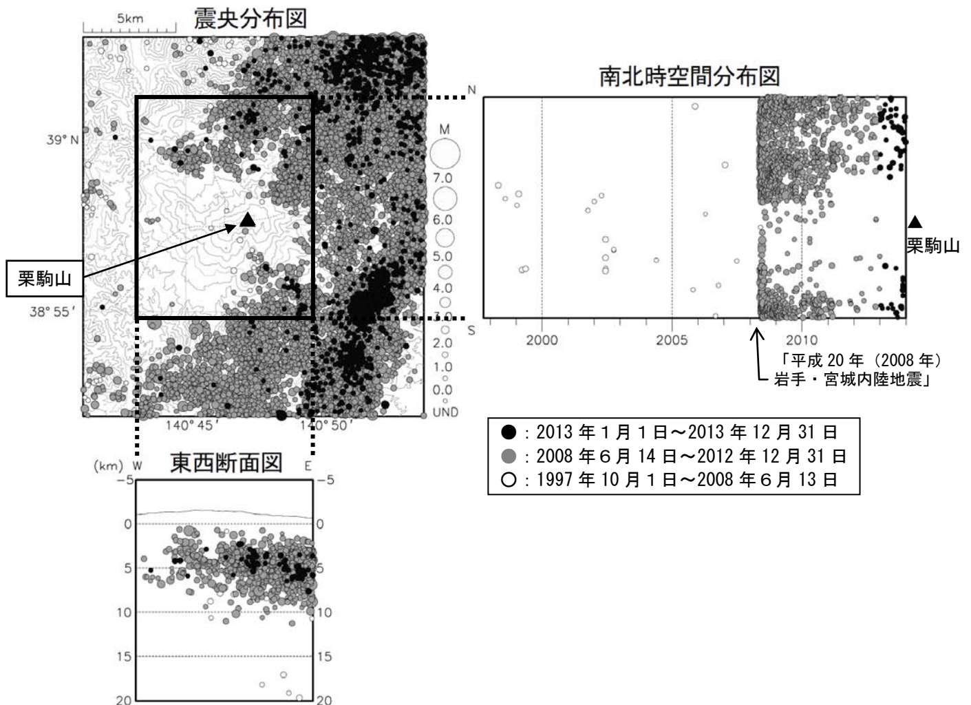
図8 栗駒山 広域地震観測網による栗駒山周辺の地震活動（1997年10月～2013年12月）
