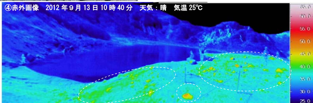
図 4 栗駒山 昭和湖の可視画像と地表面温度分布 1)
