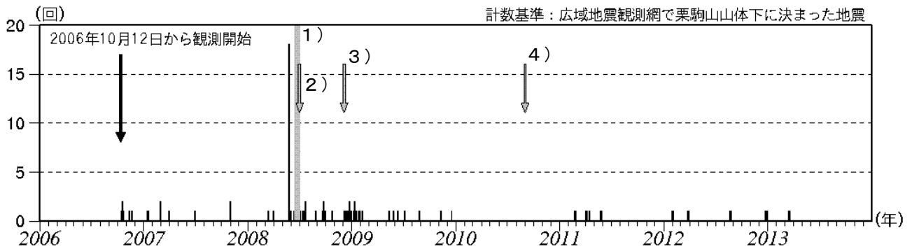
図7 栗駒山 日別地震回数（2006年10月～2013年12月）
