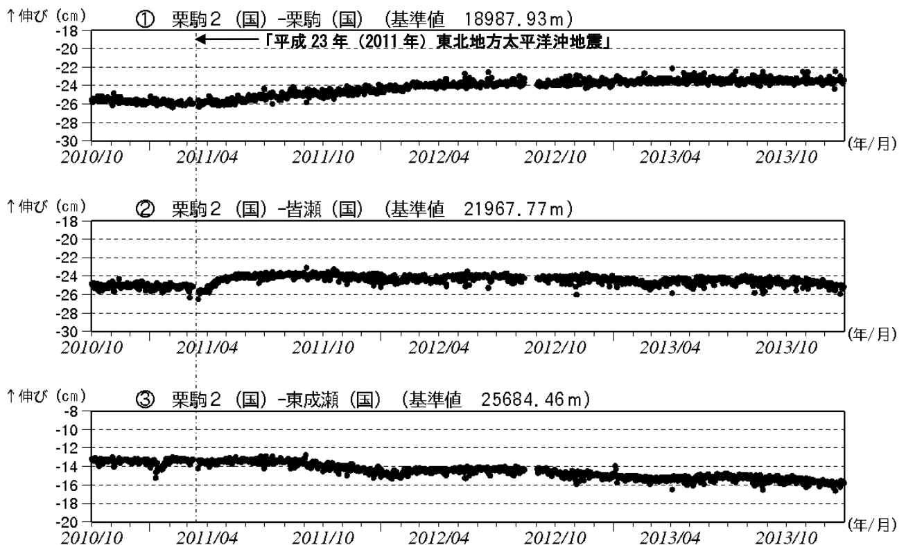
図 10 栗駒山 GPS 基線長変化図 (2010 年 10 月～2013 年 12 月)
