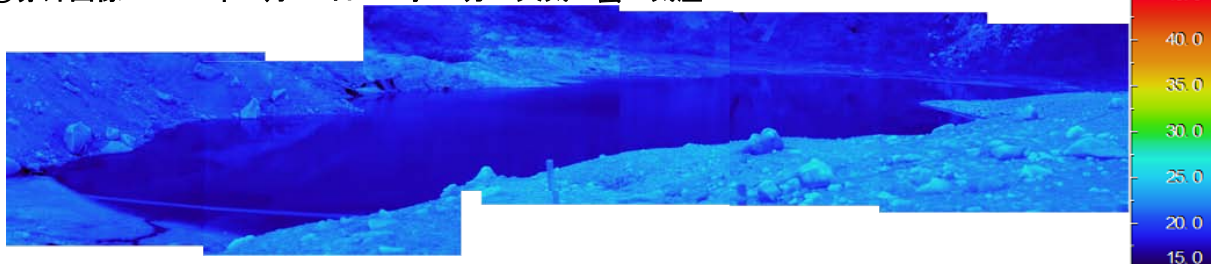
②赤外画像 2013 年 9 月 12 日 09 時 47 分 天気：曇 気温 21℃
