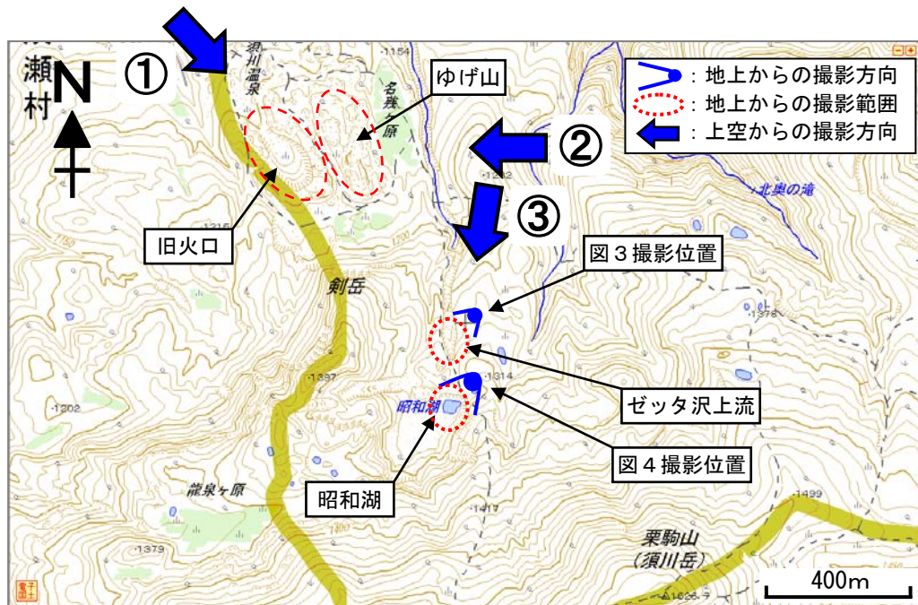
図2 栗駒山 可視画像と地表面温度分布 1) 撮影位置と撮影ポイント
