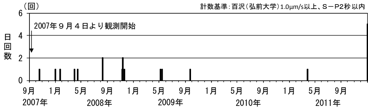
図 2※ 岩木山 日別地震回数 (2007 年 9 月～2011 年 12 月) 弘前大学からのデータ提供により、2007 年 9 月 4 日から観測を開始しています。
