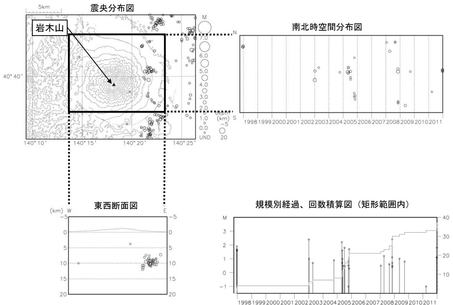
図 3※ 広域地震観測網による岩木山周辺の地震活動 (1997 年 10 月～2011 年 12 月)
