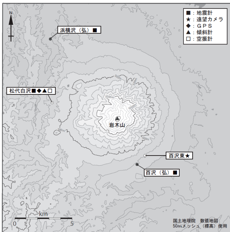
図 4 岩木山 観測点配置図
