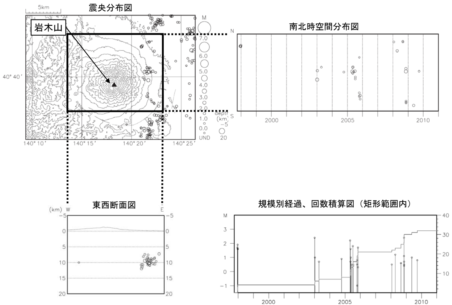
図 3※ 岩木山周辺の地震活動 (1997 年 10 月～2010 年 12 月)
