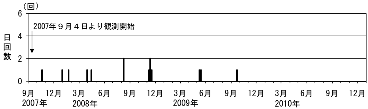
図 2※ 岩木山 日別地震回数 (2007 年 9 月～2010 年 12 月)
