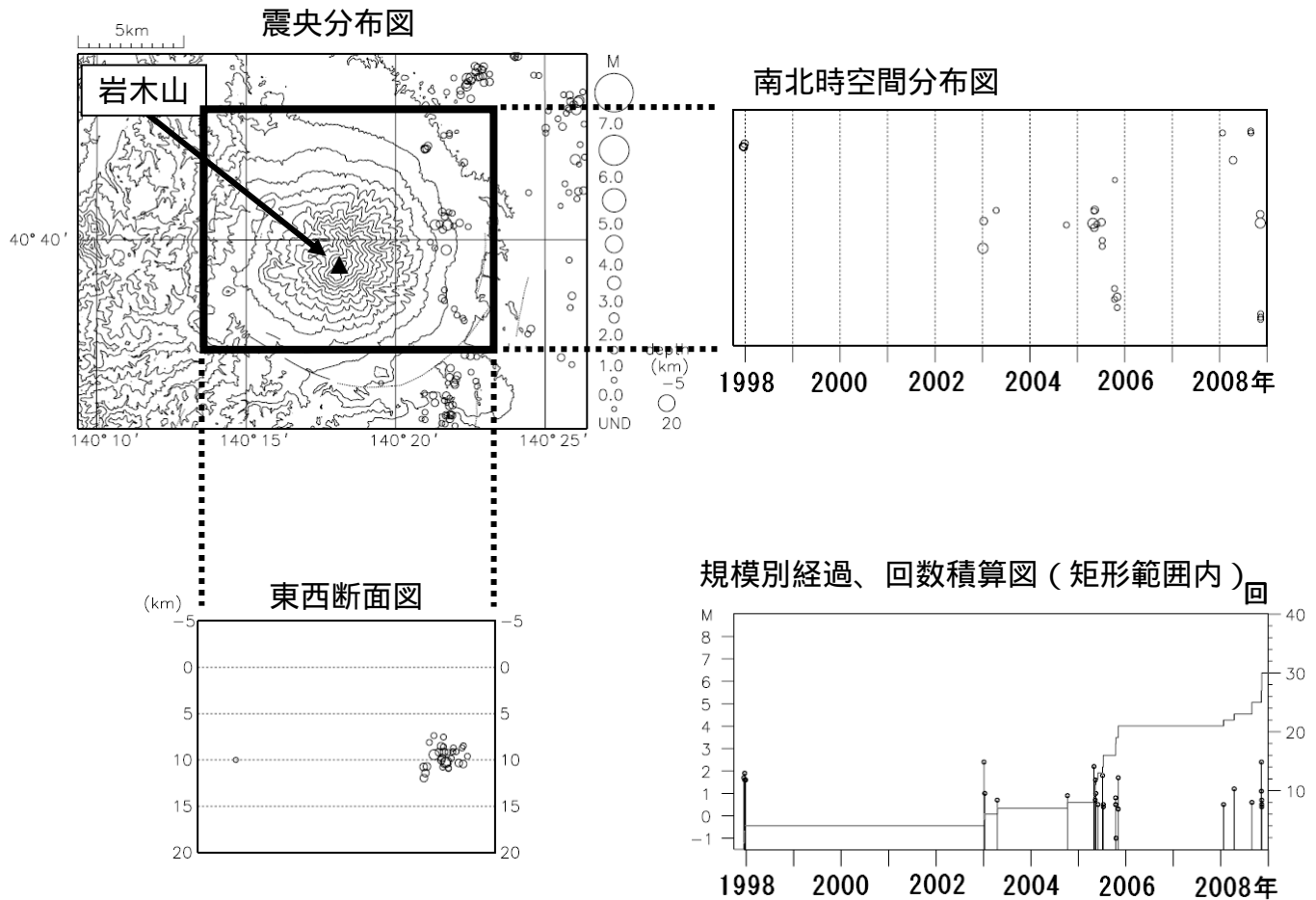
図 2 岩木山周辺の地震活動（1997 年 10 月～2008 年 12 月）
