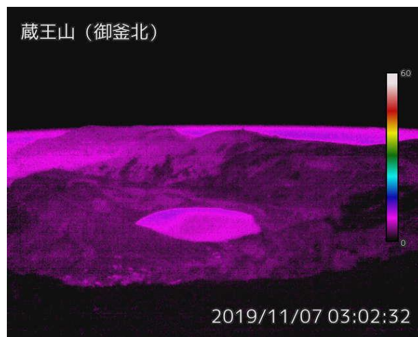
図 2 蔵王山 山頂部の地表面温度分布（11 月 7 日）
