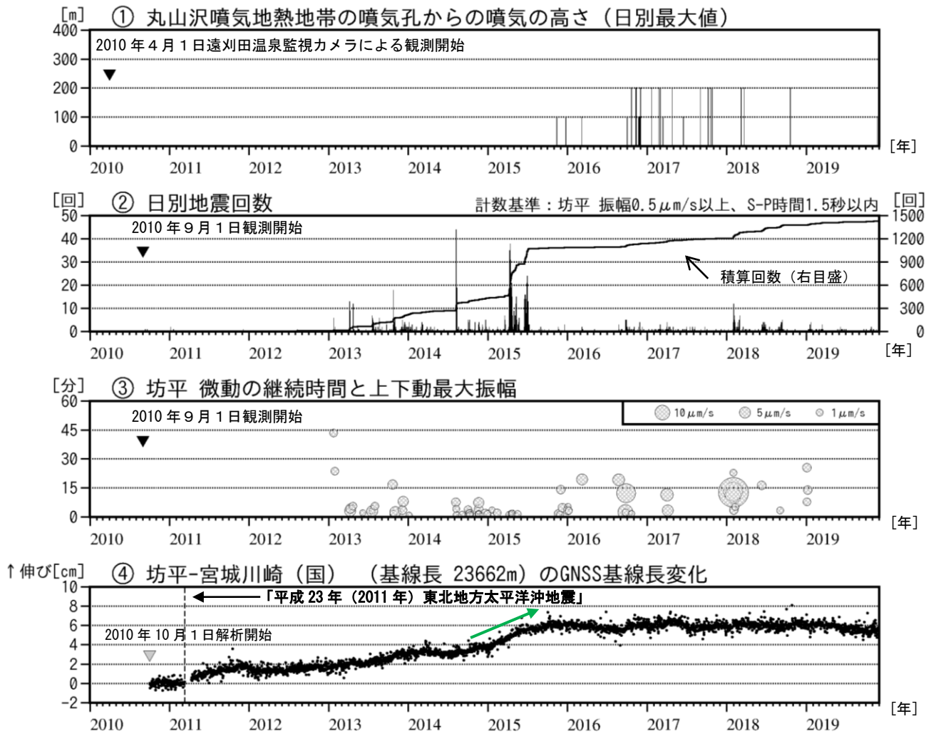
図3 蔵王山 火山活動経過図（2010年4月～2019年11月）
