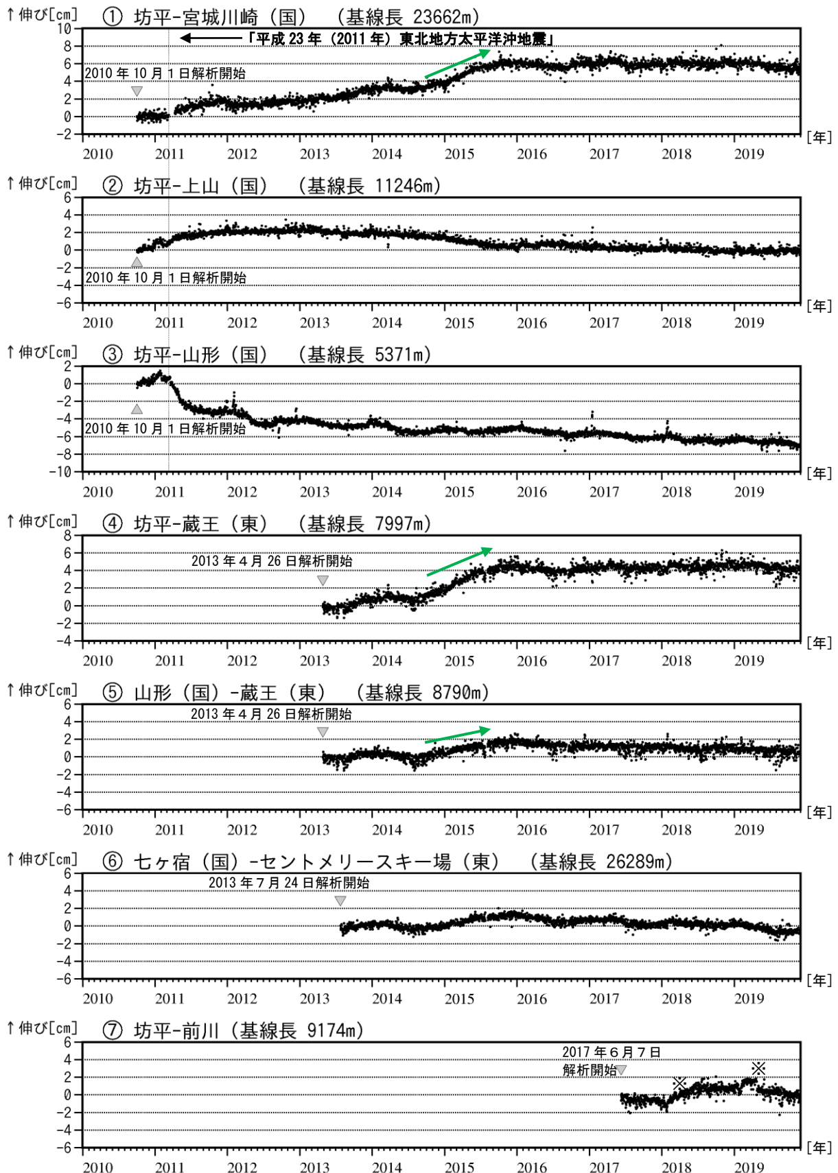
図5 蔵王山 GNSS 基線長変化図 (2010 年 10 月～2019 年 11 月)
