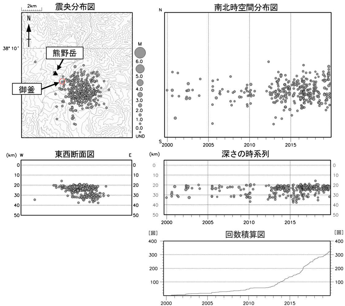
図 4 蔵王山 広域地震観測網による深部低周波地震活動（1999 年 9 月～2019 年 11 月）
