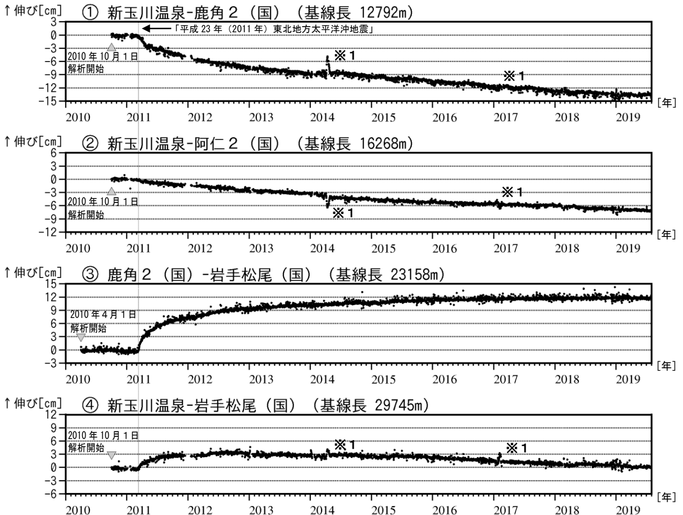
図3 秋田焼山 GNSS 基線長変化図（2010年4月～2019年7月）
