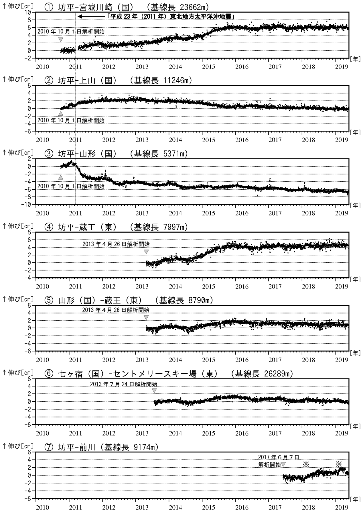
図4 蔵王山 GNSS 基線長変化図 (2010年10月～2019年5月)
