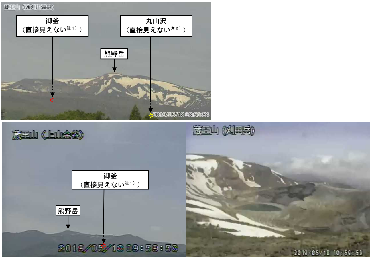
図1 蔵王山 山頂部の状況（5月18日）
