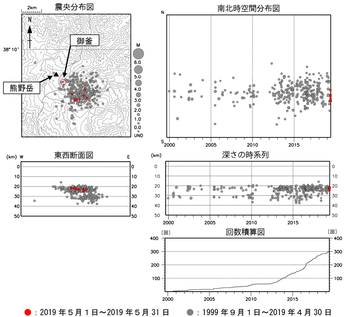
図3 蔵王山 広域地震観測網による深部低周波地震活動（1999 年 9 月～2019 年 5 月）
