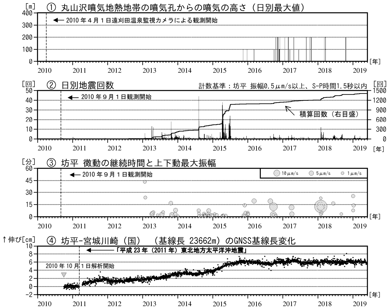
図2 蔵王山 火山活動経過図（2010年4月～2019年5月）
