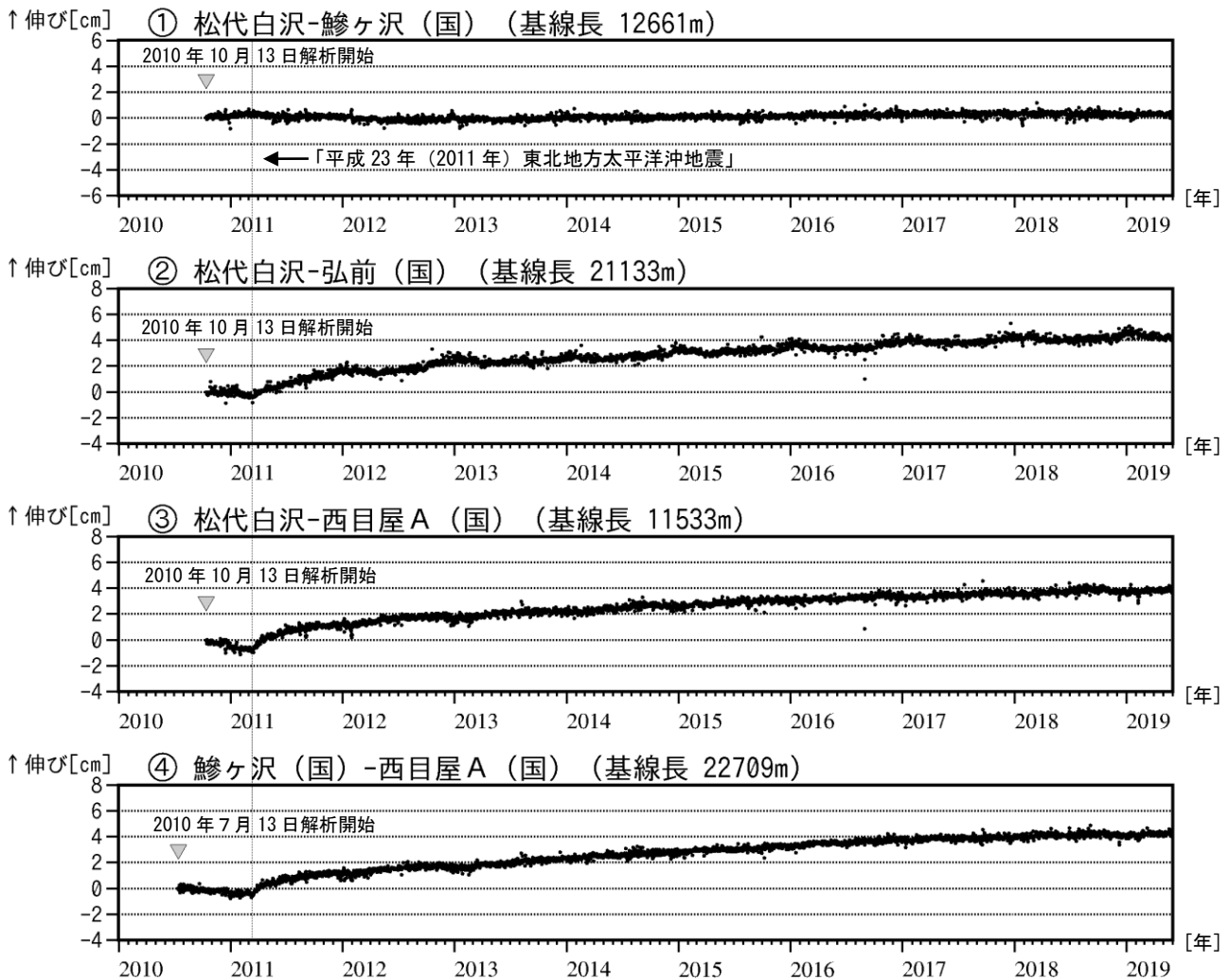
図3 岩木山 GNSS 基線長変化図（2010年7月～2019年5月）
