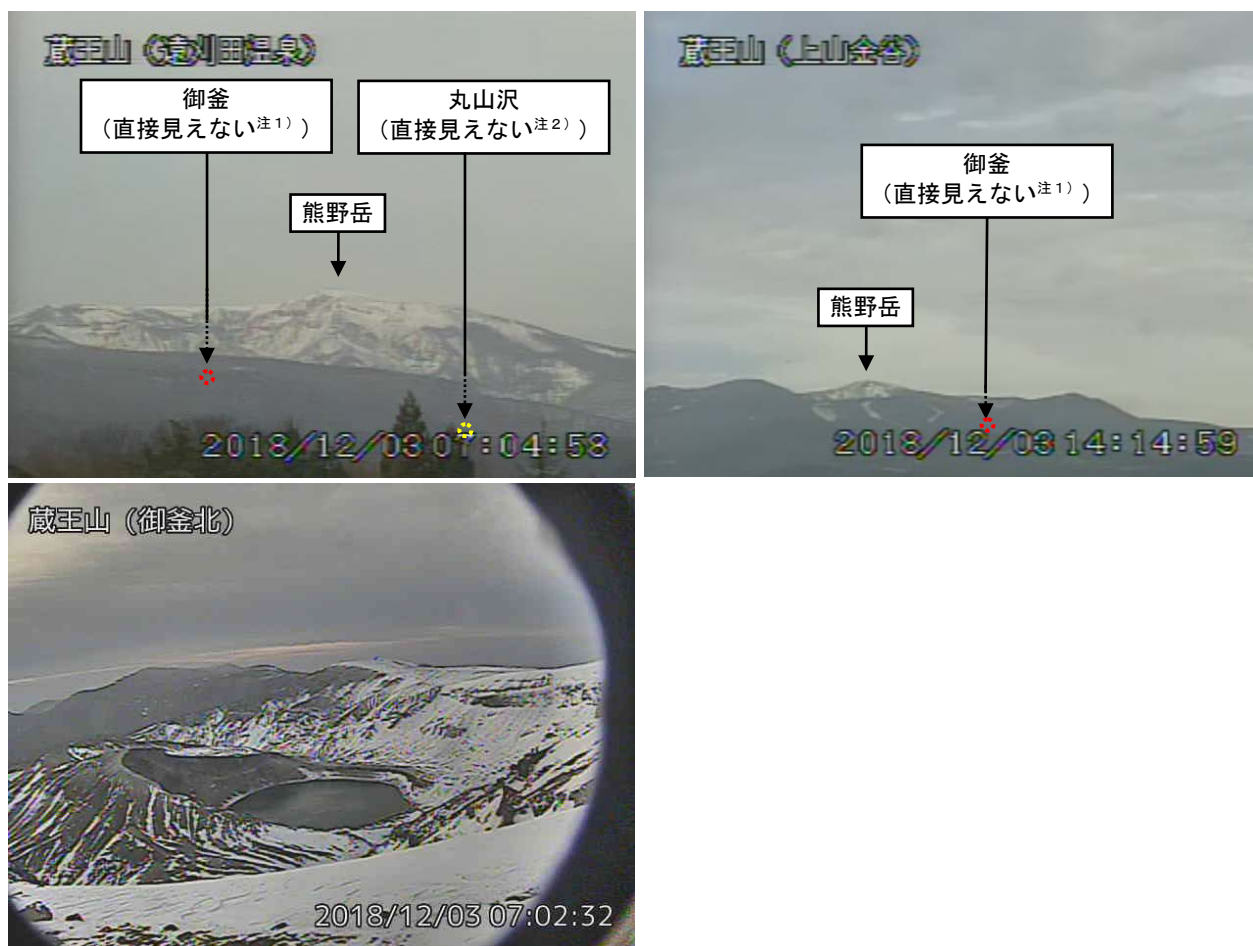
図1 蔵王山 山頂部の状況（12月3日）
