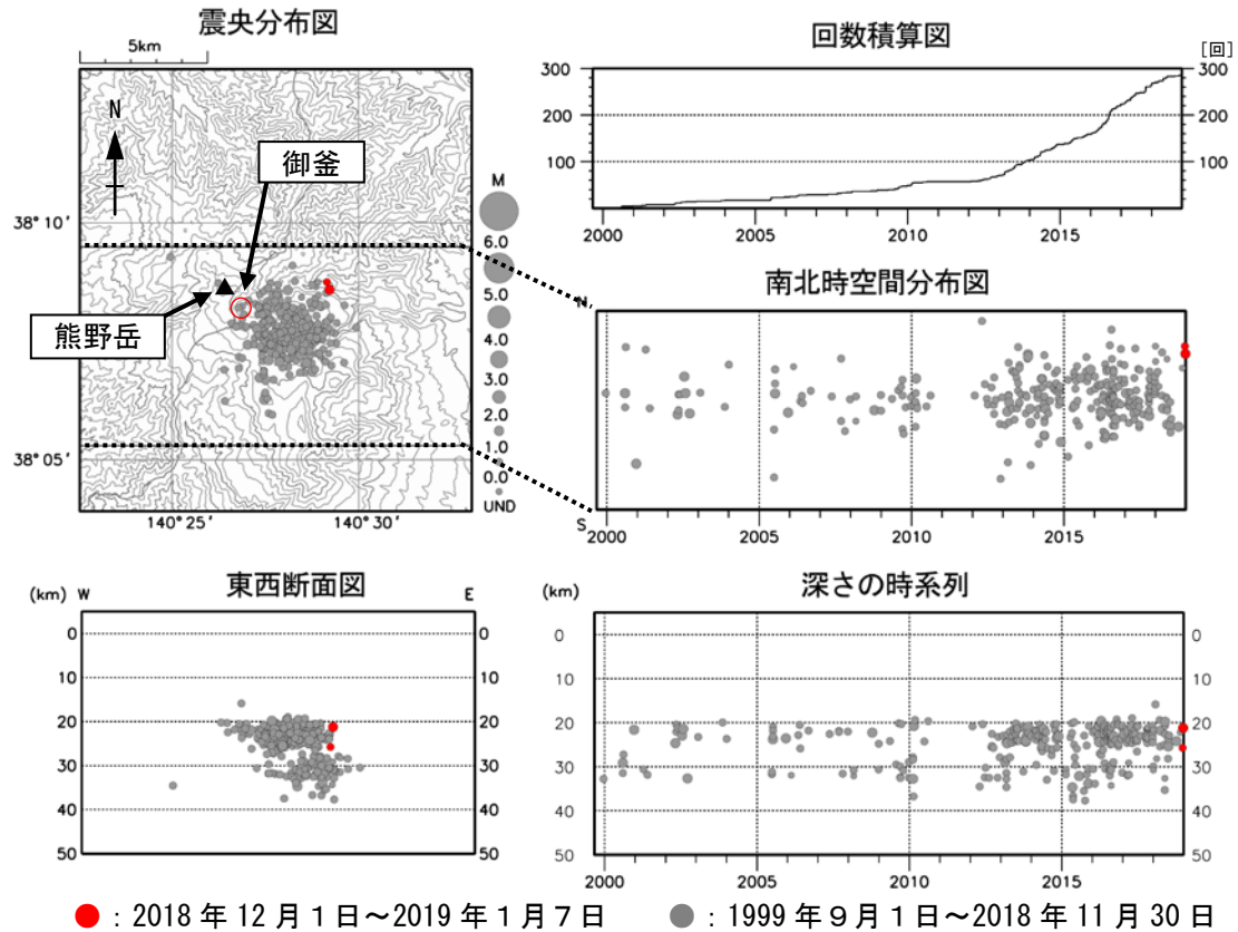
図 6 蔵王山 広域地震観測網による深部低周波地震活動（1999 年 9 月～2019 年 1 月 7 日）
