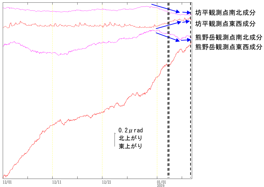
図 7 蔵王山 坊平観測点及び熊野岳観測点での傾斜変動
