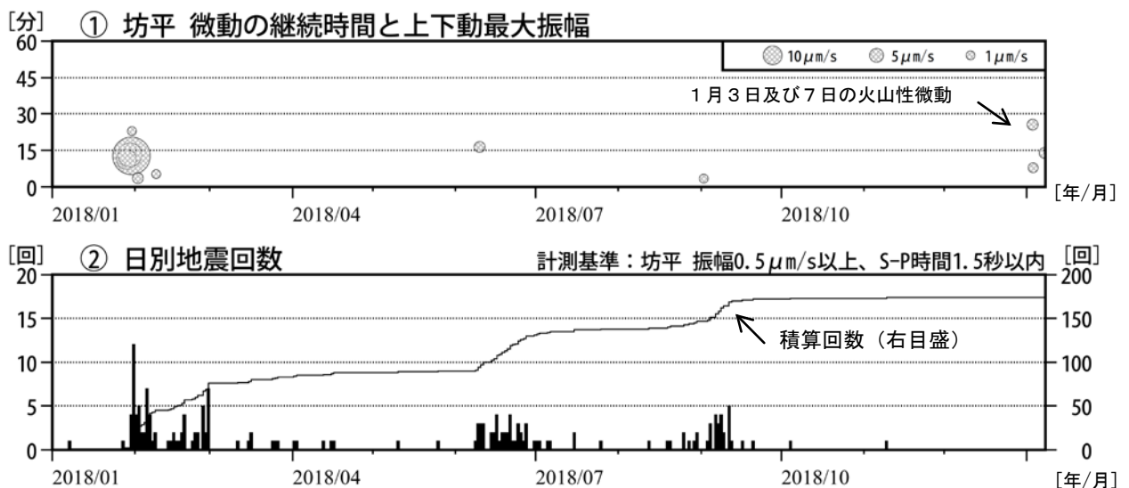
図 3 蔵王山 微動の発生状況及び日別地震回数（2018 年 1 月～2019 年 1 月 7 日）
