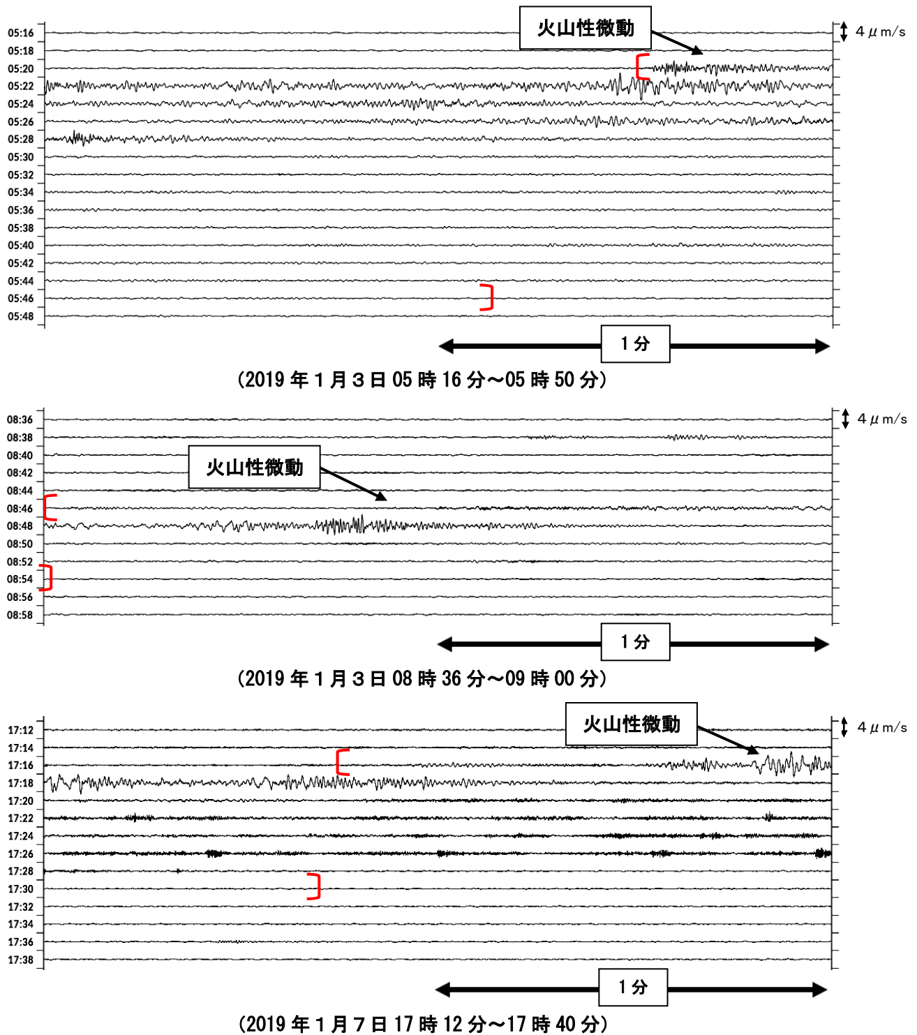
図 4 蔵王山 坊平観測点（上下成分）での火山性微動の発生状況
