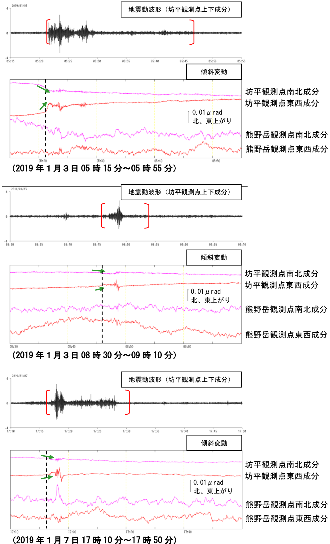
図 5 蔵王山 火山性微動波形及び傾斜変動
