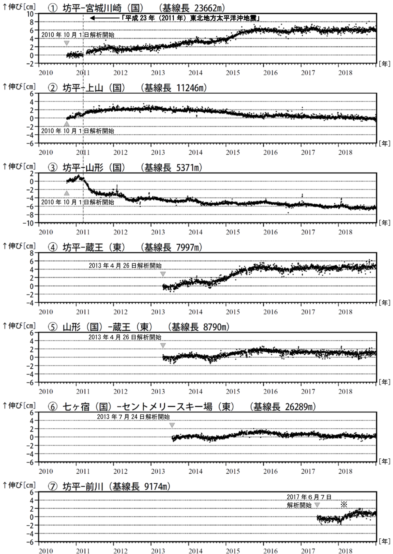
図 8 蔵王山 GNSS 基線長変化図 (2010 年 10 月～2019 年 1 月 7 日)
