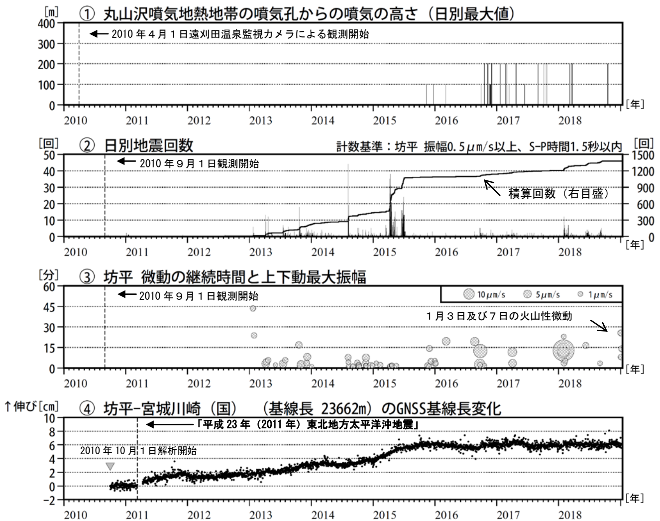
図 2 蔵王山 火山活動経過図（2010年 4 月～2019年 1 月 7 日）
