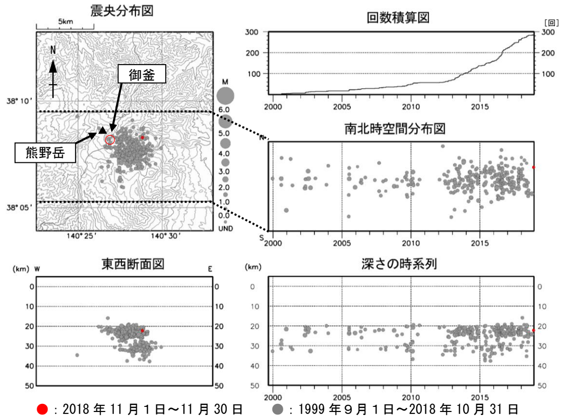
図3 蔵王山 広域地震観測網による深部低周波地震活動（1999 年 9 月～2018 年 11 月）
