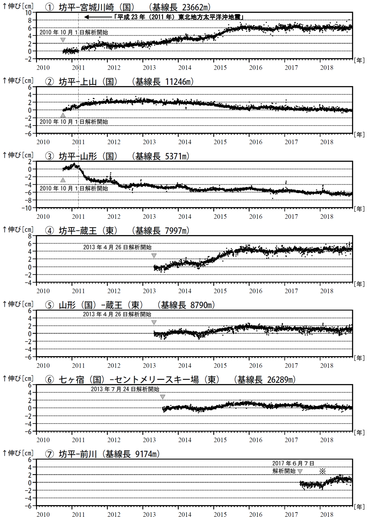
図 4 蔵王山 GNSS 基線長変化図 (2010 年 10 月～2018 年 11 月)
