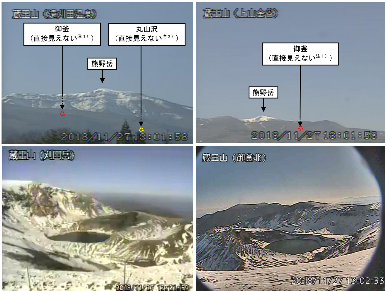
図1 蔵王山 山頂部の状況（11月27日）
