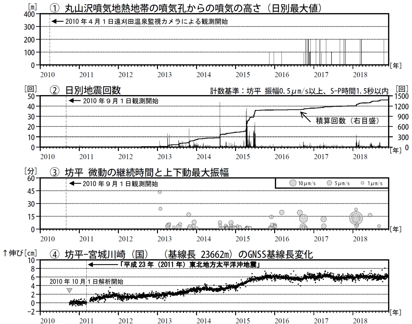
図 2 蔵王山 火山活動経過図（2010年4月～2018年11月）
