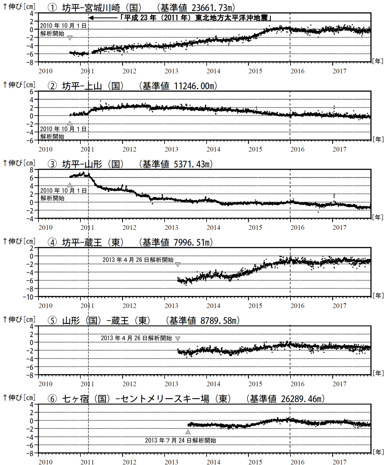
図 4 蔵王山 GNSS 基線長変化図 (2010 年 10 月～2017 年 11 月)
