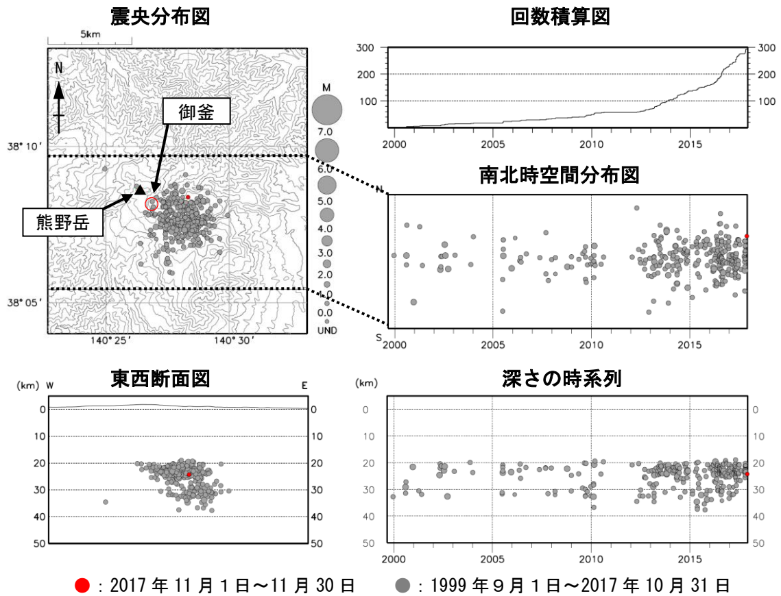
図3 蔵王山 広域地震観測網による深部低周波地震活動（1999 年 9 月～2017 年 11 月）
