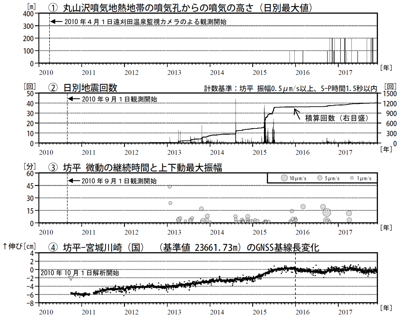
図2 蔵王山 火山活動経過図（2010年4月～2017年11月）
