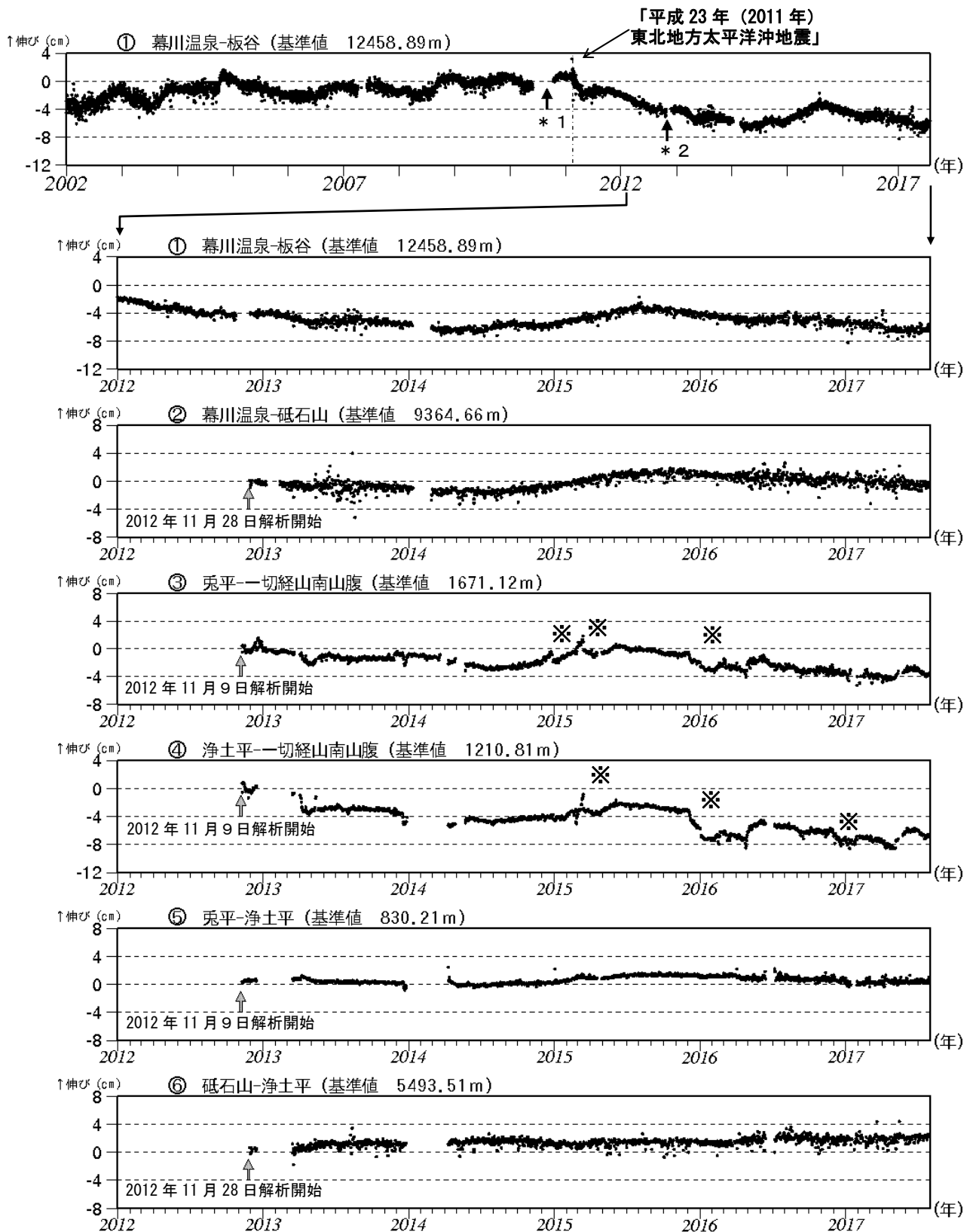
図 3 吾妻山 GNSS 1) 基線長変化図 (2002 年 1 月～2017 年 7 月)
