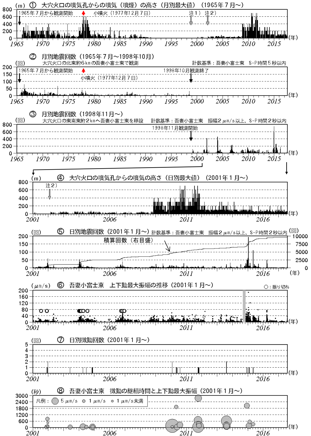
図2 吾妻山 火山活動経過図 (1965年7月～2017年7月)
