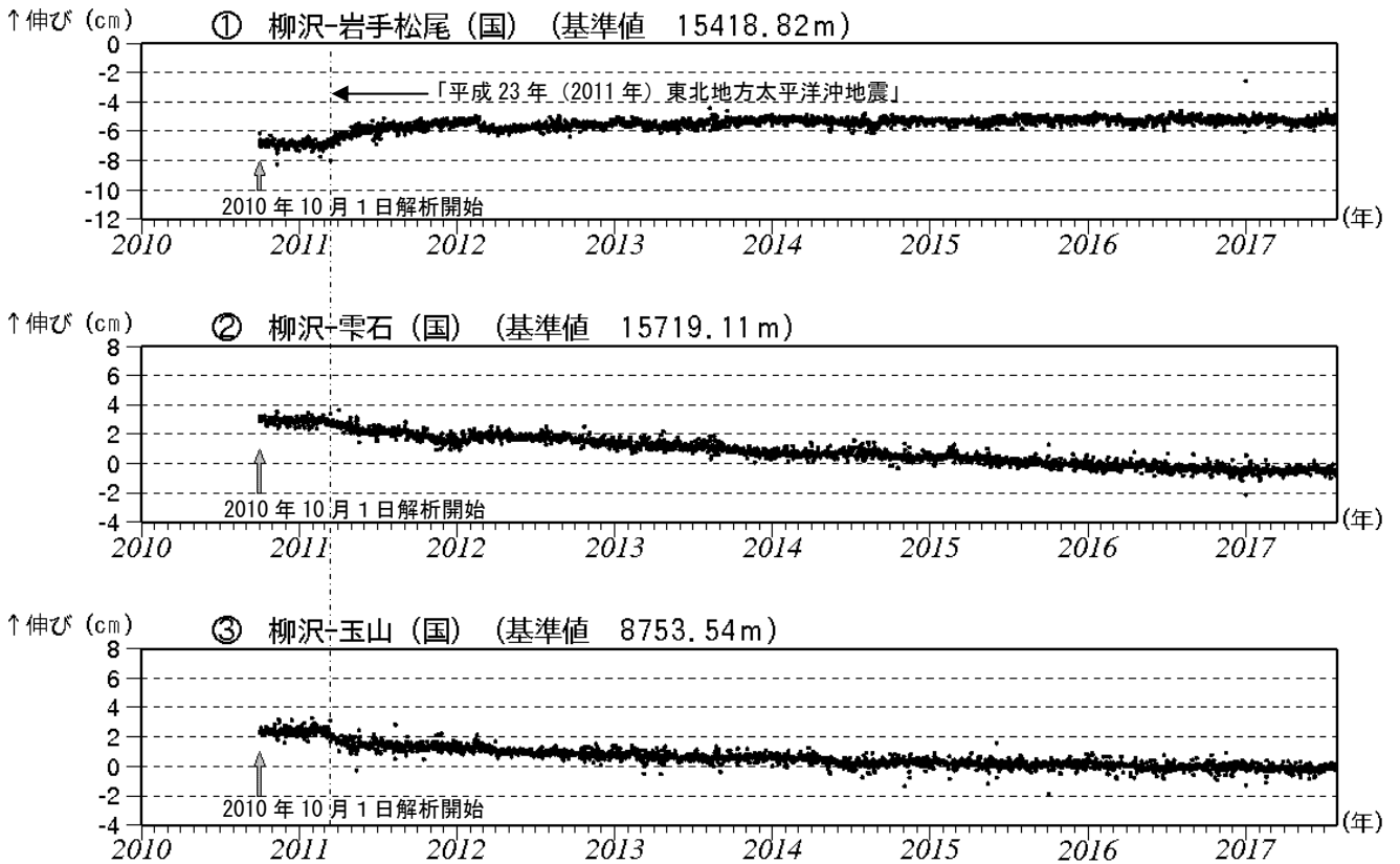
図 5 岩手山 GNSS 1) 基線長変化図（2010 年 10 月～2017 年 7 月）
