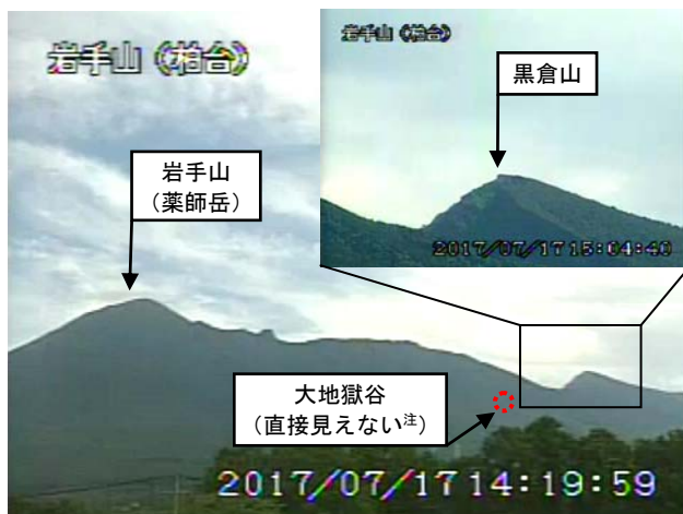
図 1 岩手山 黒倉山の噴気の状況 （7 月 17 日）
