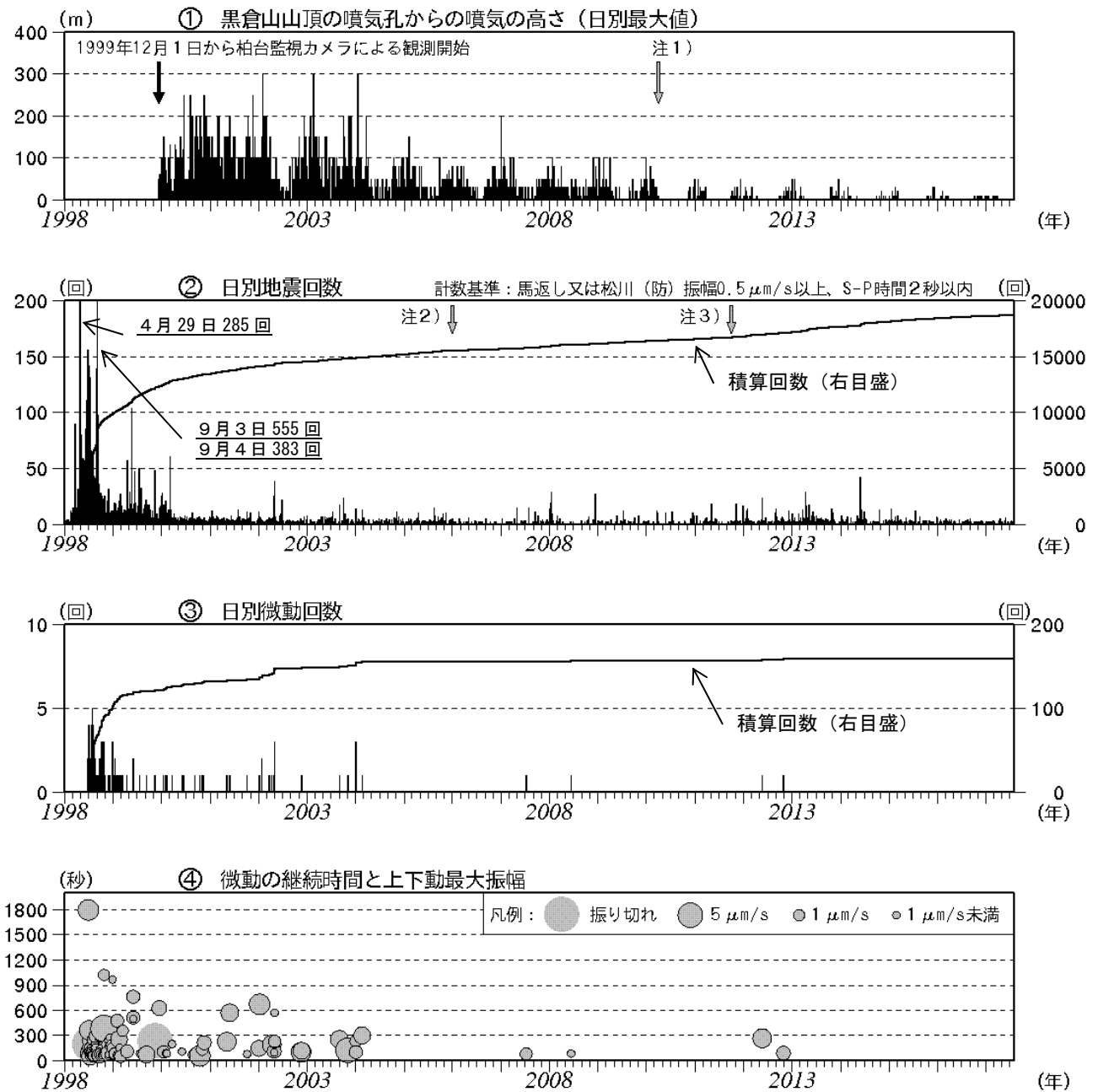
図3 岩手山 火山活動経過図（1998年1月～2017年7月）
