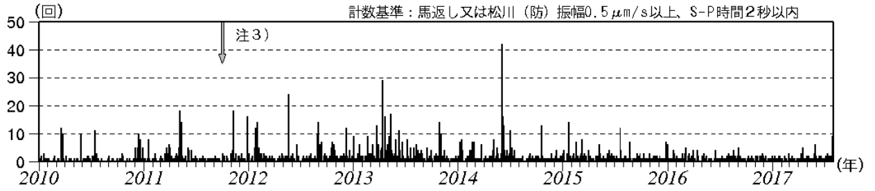
図 4 岩手山 日別地震回数（2010 年 1 月～2017 年 7 月）
