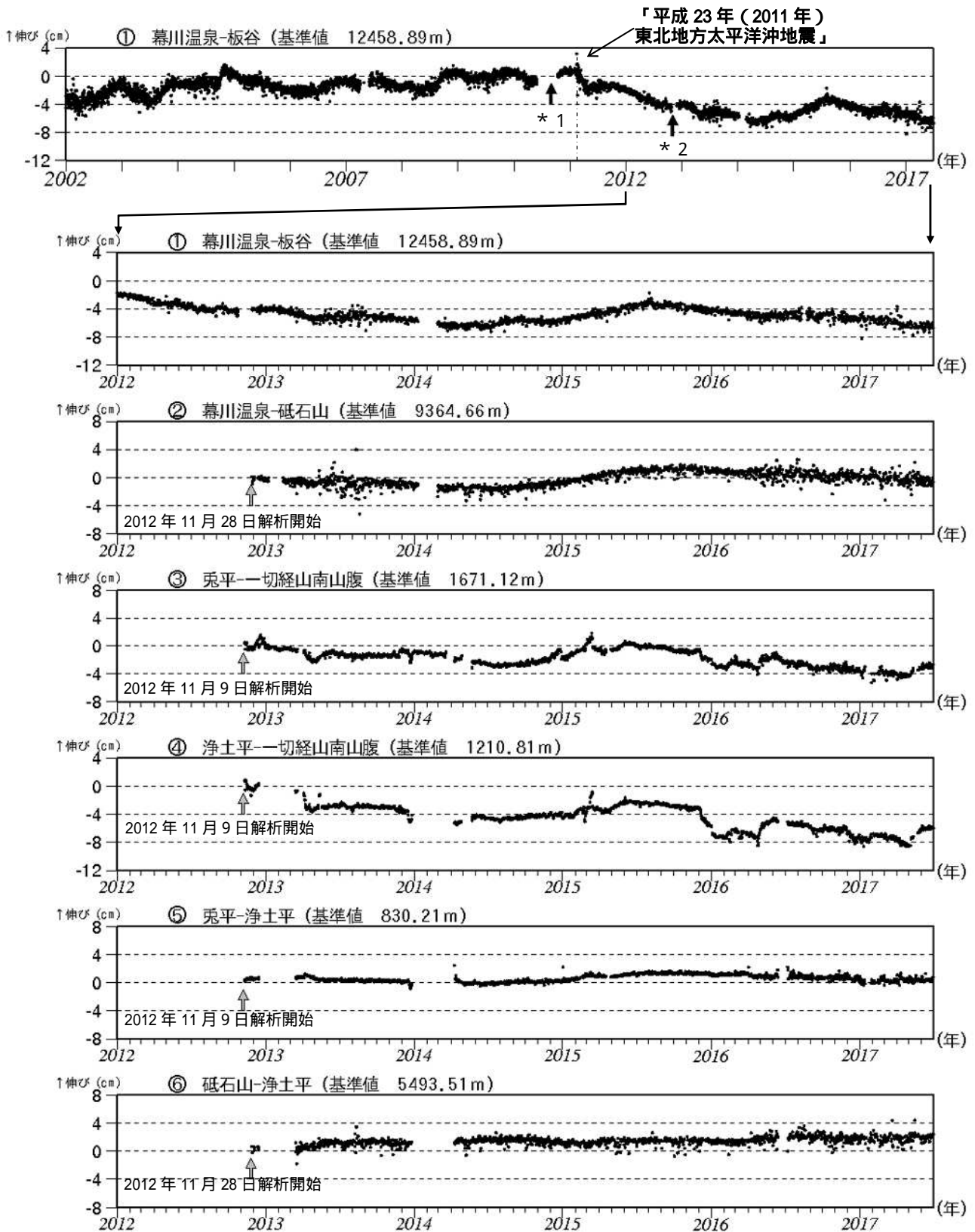
図 3 吾妻山 GNSS 1) 基線長変化図 (2002 年 1 月 ~ 2017 年 6 月)
