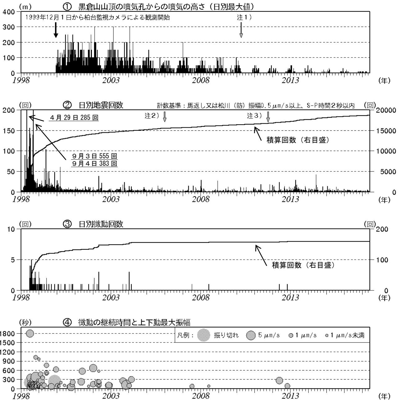
図3 岩手山 火山活動経過図（1998年1月～2017年5月）
