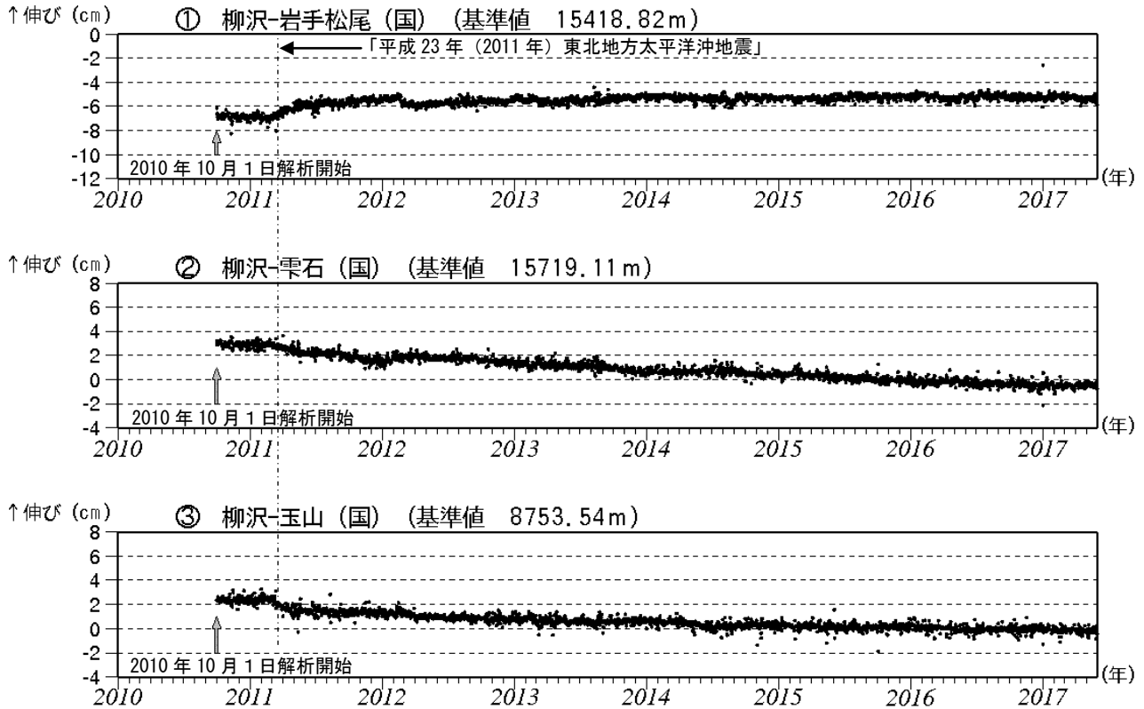
図5 岩手山 GNSS 1) 基線長変化図（2010年10月～2017年5月）
