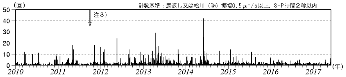
図4 岩手山 日別地震回数（2010年1月～2017年5月）
