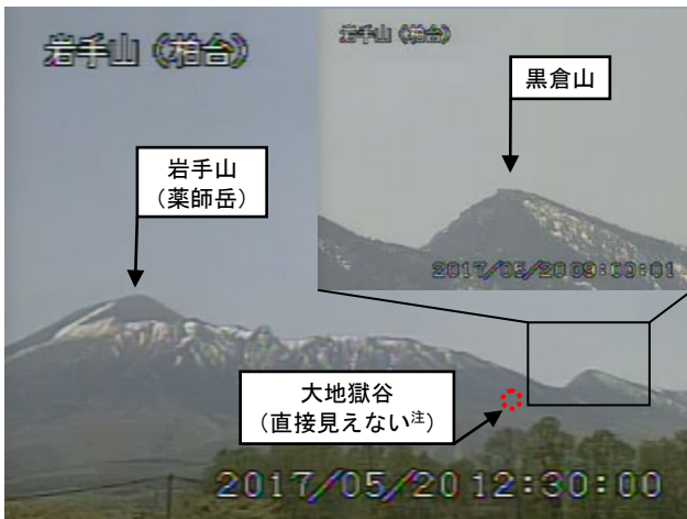
図 1 岩手山 黒倉山の噴気の状況 （5月20日）
