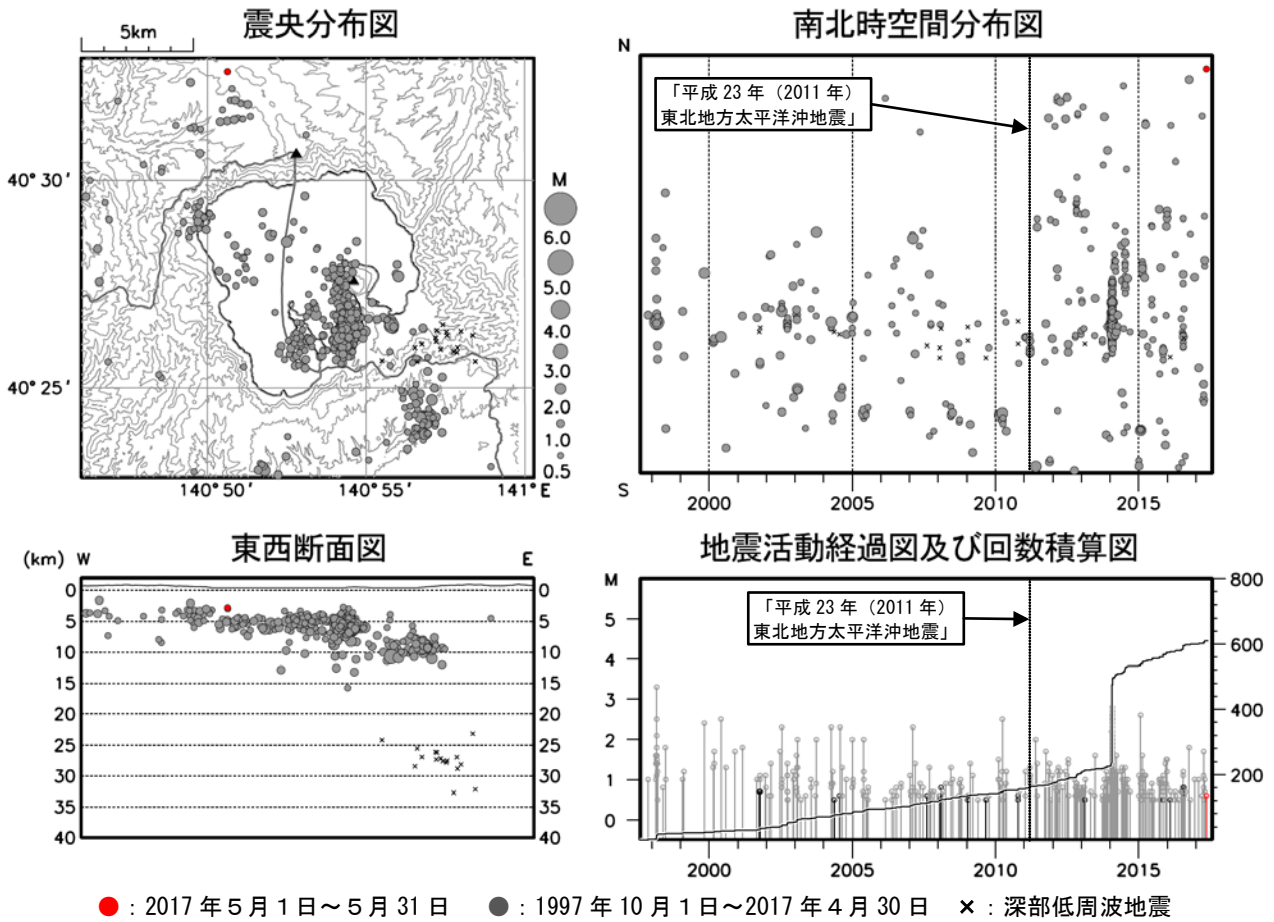
図3 十和田 広域地震観測網による十和田周辺の地震活動図（1997年10月～2017年5月）
