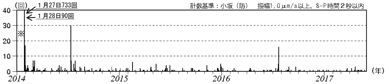
図2 十和田 日別地震回数（2014年1月～2017年5月）
