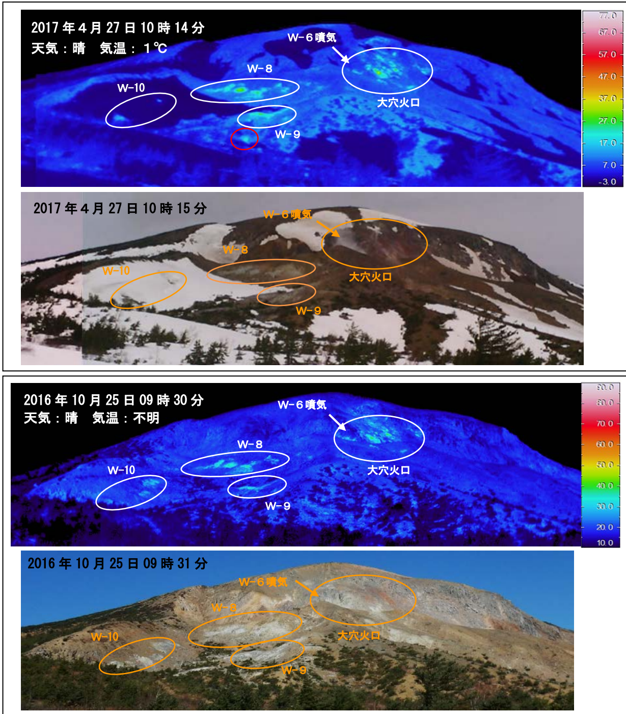
図3 吾妻山 大穴火口及び八幡焼の状況と地表面温度分布
