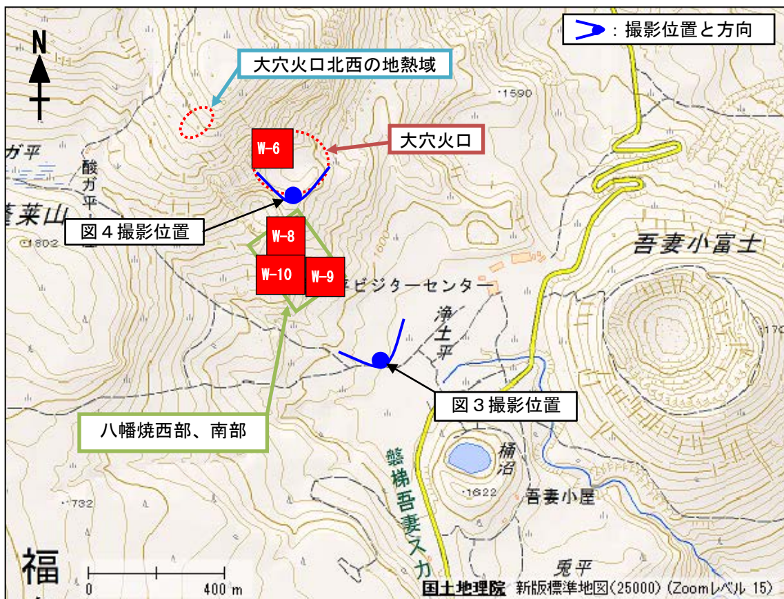
図2 吾妻山 大穴火口付近の地熱域の分布及び写真と地表面温度分布 1) 撮影位置
