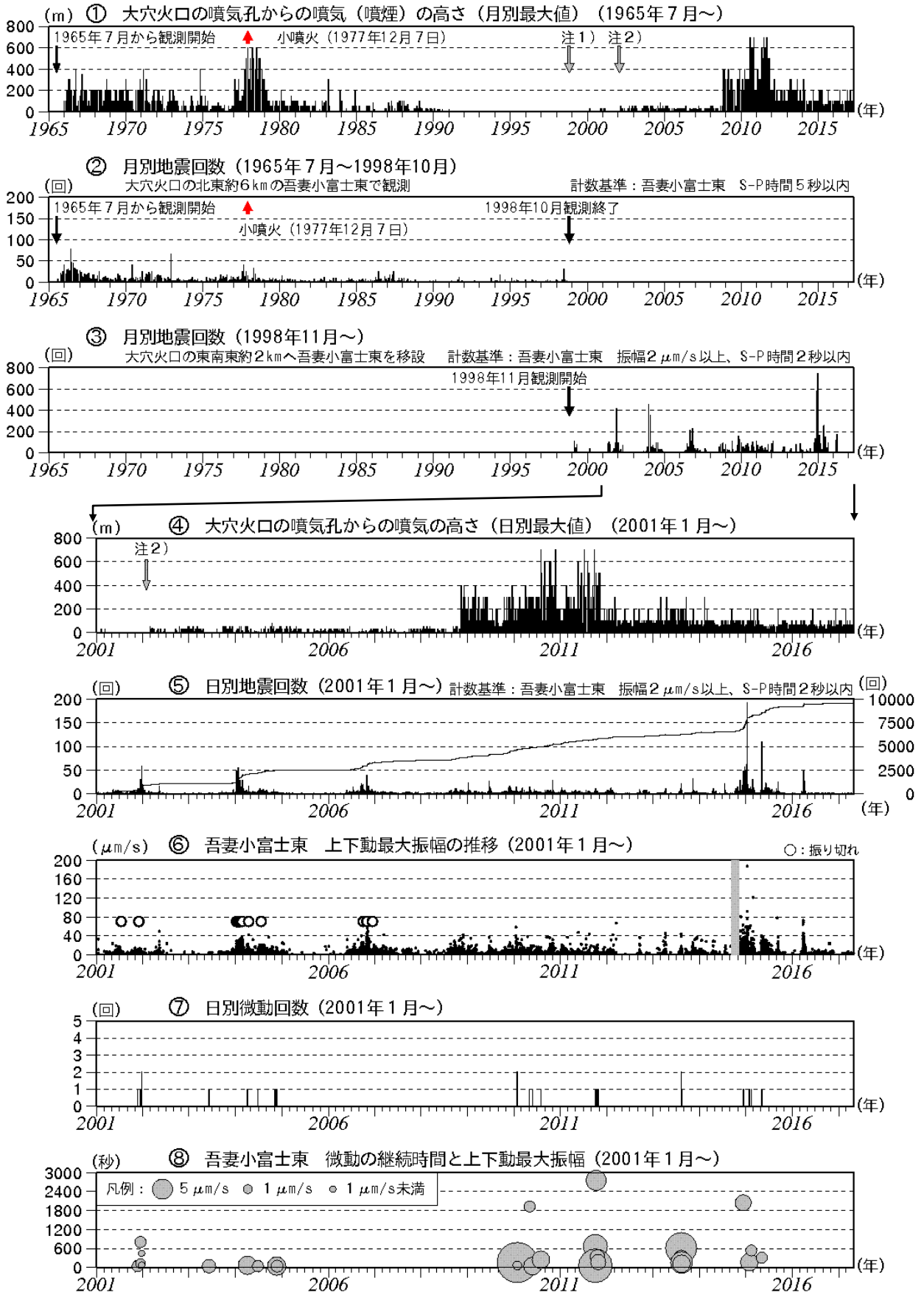
図5 吾妻山 火山活動経過図(1965年7月~2017年4月)
