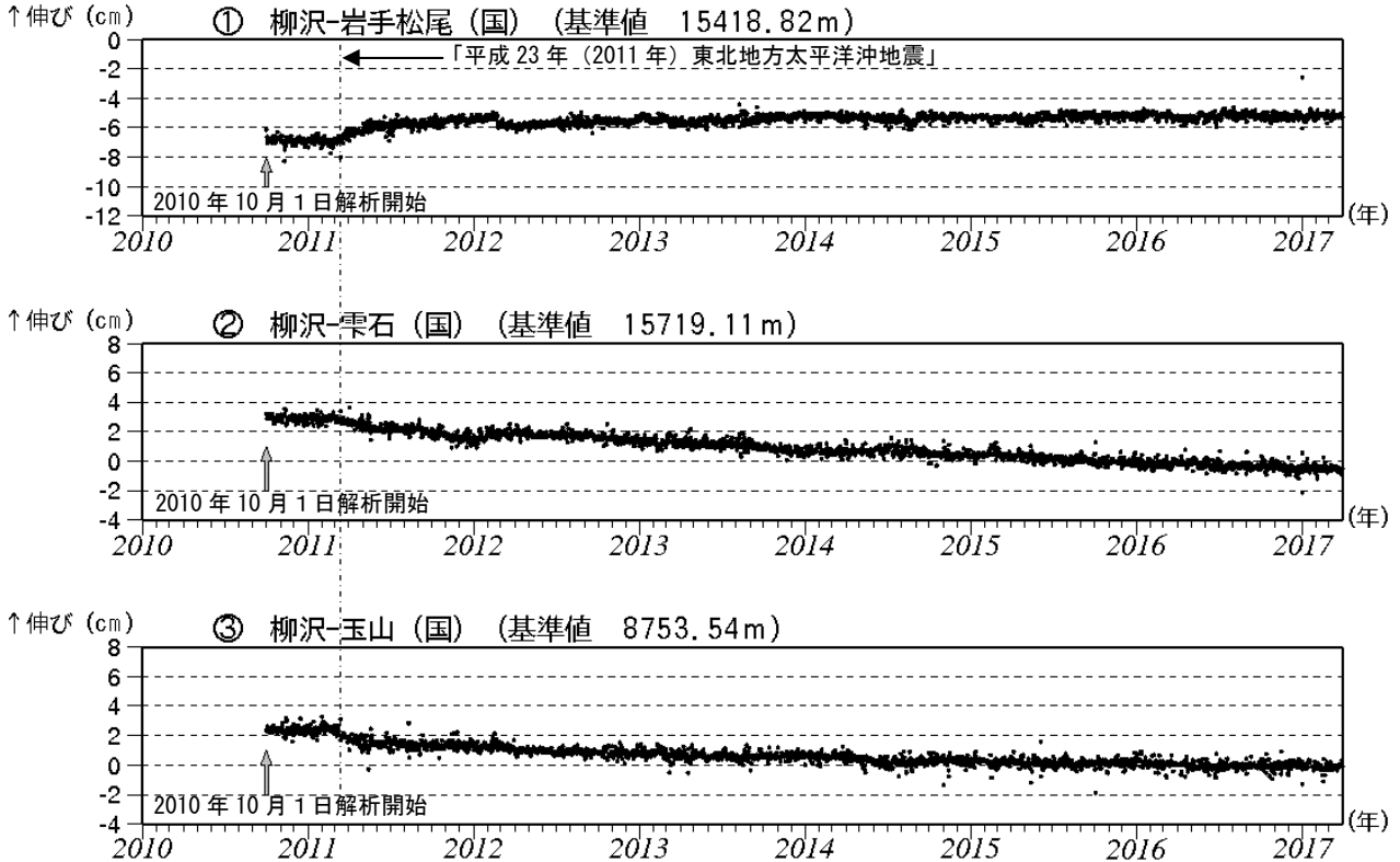
図5 岩手山 GNSS 1) 基線長変化図（2010年10月～2017年3月）
