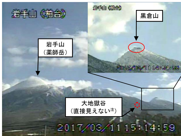
図 1 岩手山 黒倉山の噴気の状況 （3月11日）
