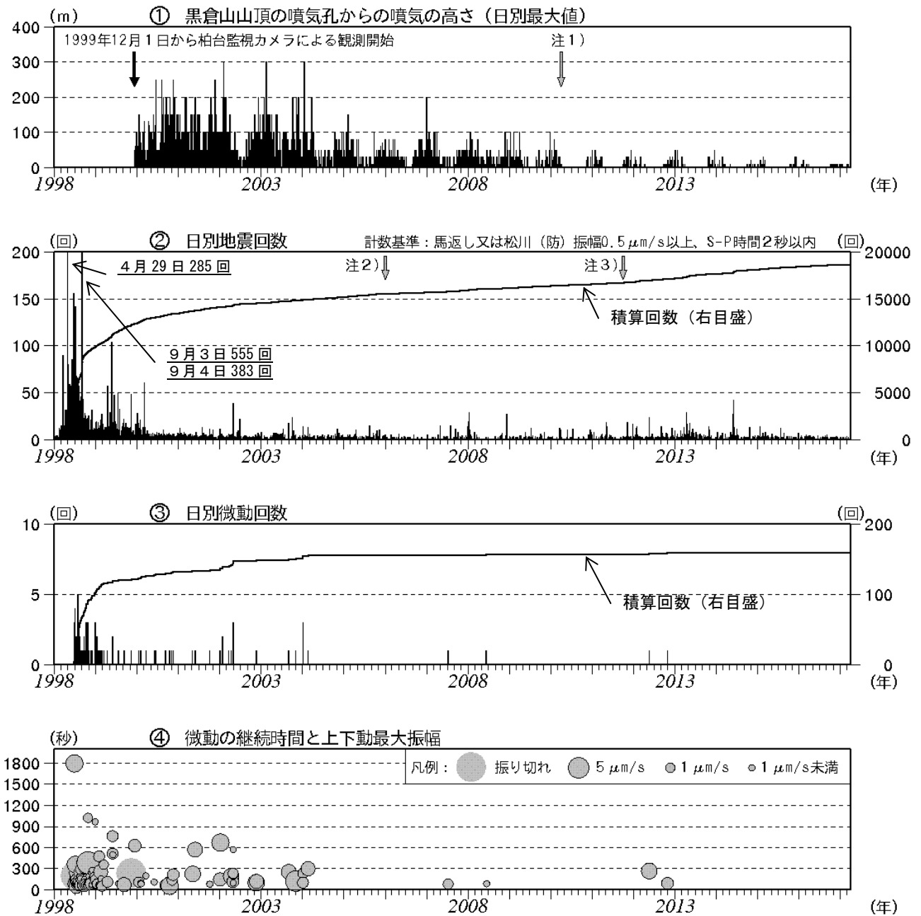
図3 岩手山 火山活動経過図（1998年1月～2017年3月）
