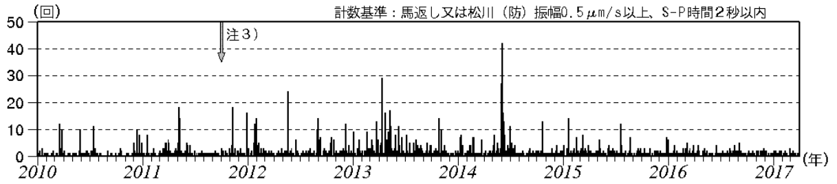
図4 岩手山 日別地震回数（2010年1月～2017年3月）
