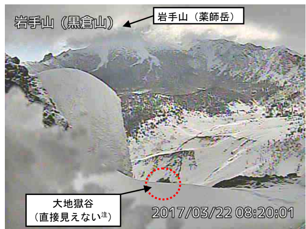
図 2 岩手山 黒倉山監視カメラからの状況 （3月22日）
