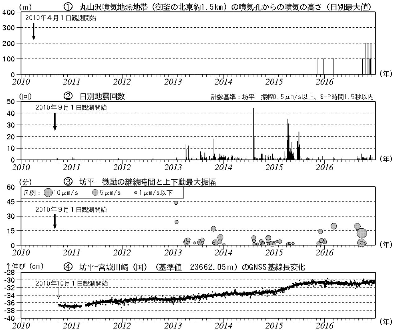
図2 蔵王山 火山活動経過図 (2010年4月~2016年12月)
