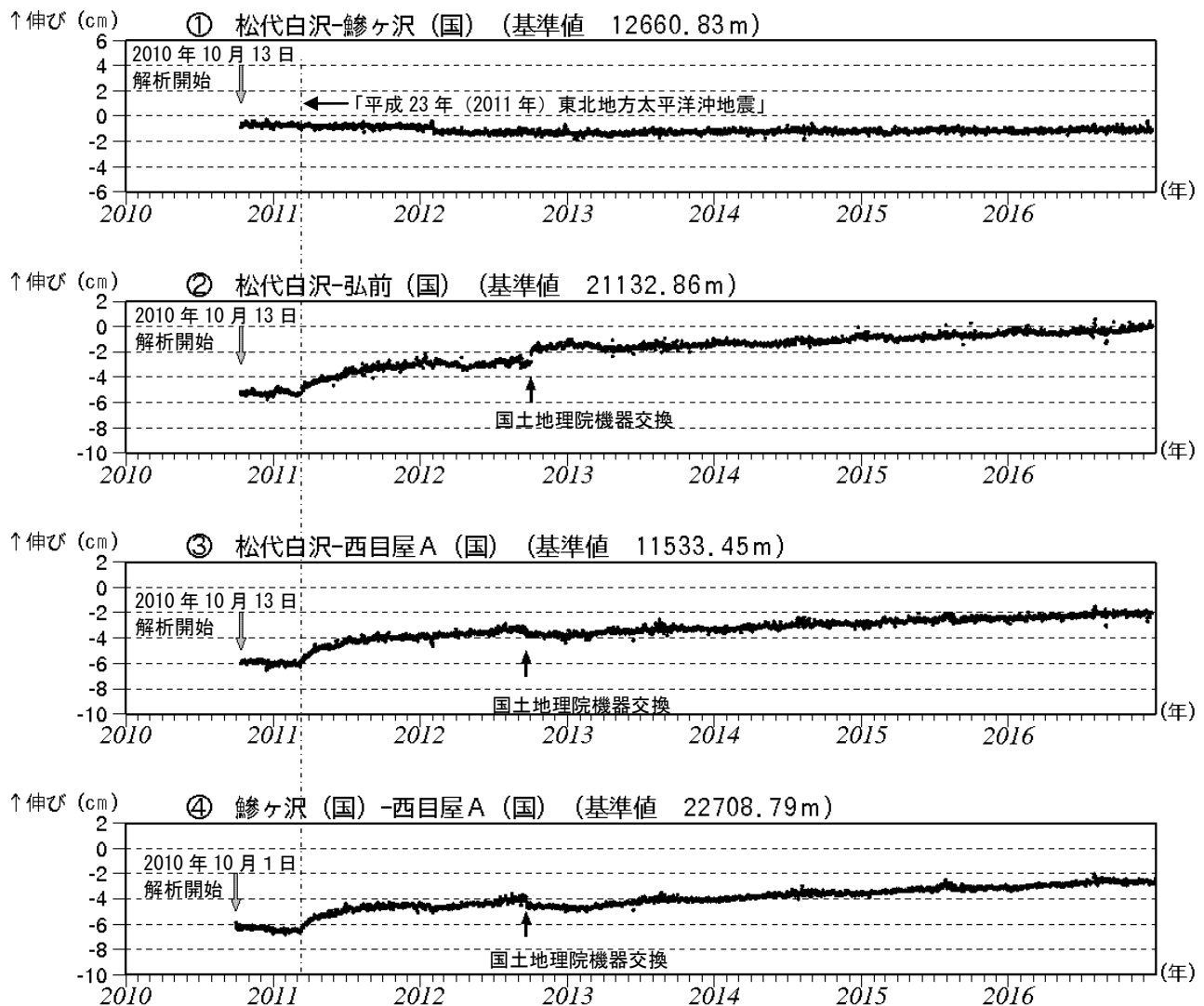
図3 岩木山 GNSS 1) 基線長変化図（2010年10月～2016年12月）
