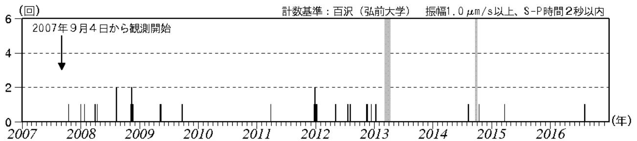
図2 岩木山 日別地震回数（2007年9月～2016年12月）
