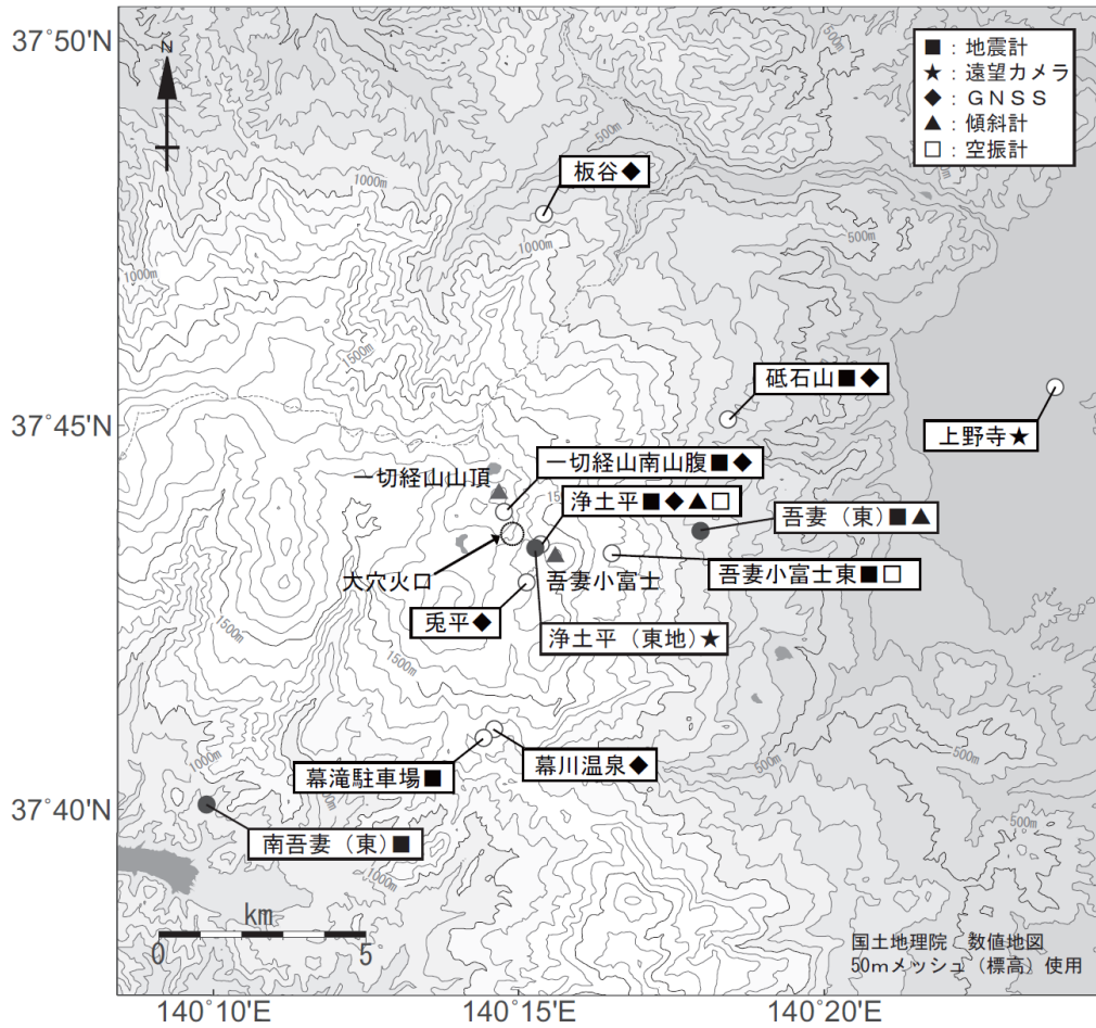
図7 吾妻山 観測点配置図
