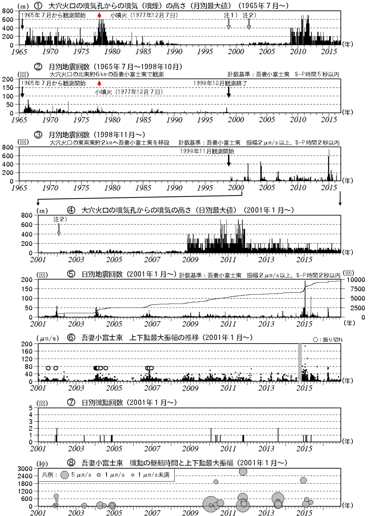
図2 吾妻山 火山活動経過図(1965年7月~2016年11月)
