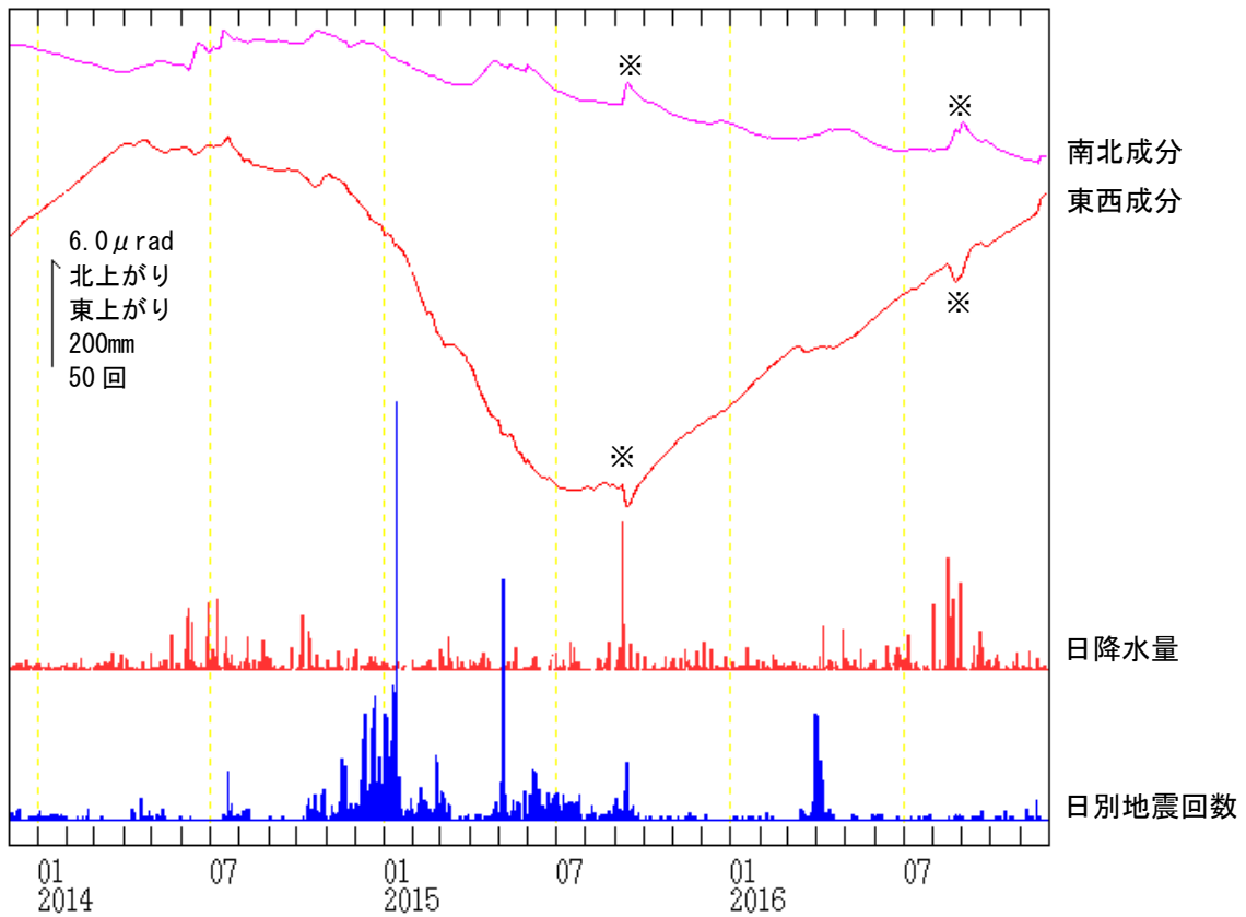
図 4 吾妻山 浄土平観測点での傾斜変動
