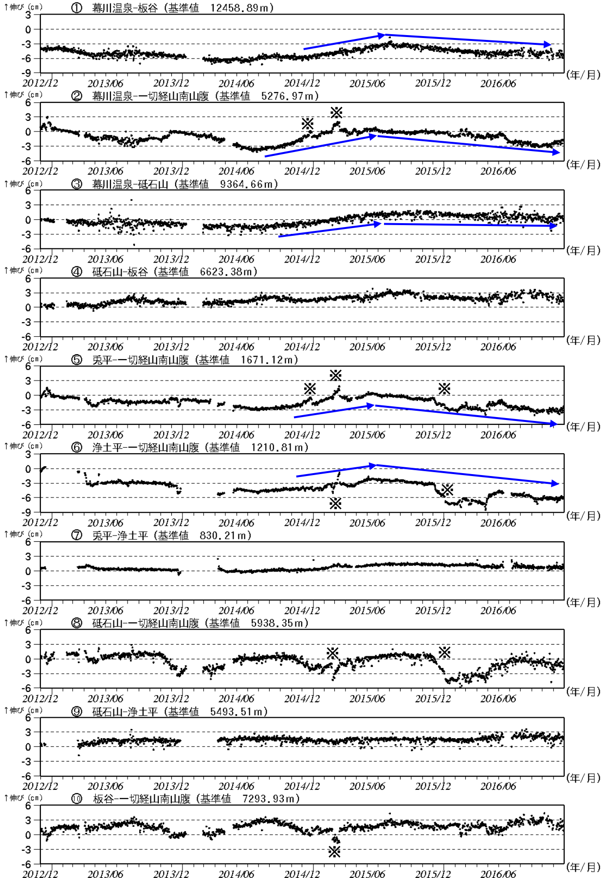
図 6-2 吾妻山 GNSS 基線長変化図 (2012 年 12 月～2016 年 11 月)
