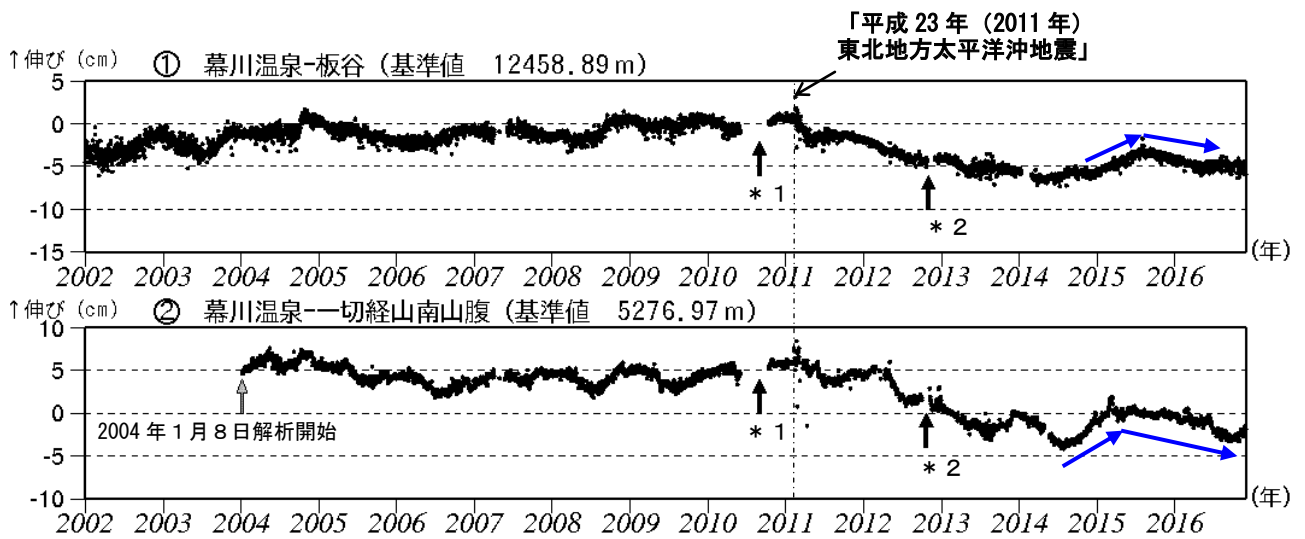
図6-1 吾妻山 GNSS 基線長変化図 (2002 年 1 月～2016 年 11 月)
