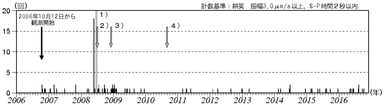
図2 栗駒山 日別地震回数（2006年10月～2016年11月）
