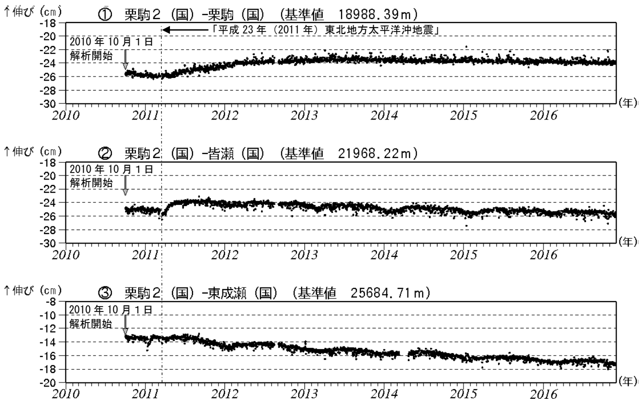
図3 栗駒山 GNSS 1) 基線長変化図（2010年10月～2016年11月）
