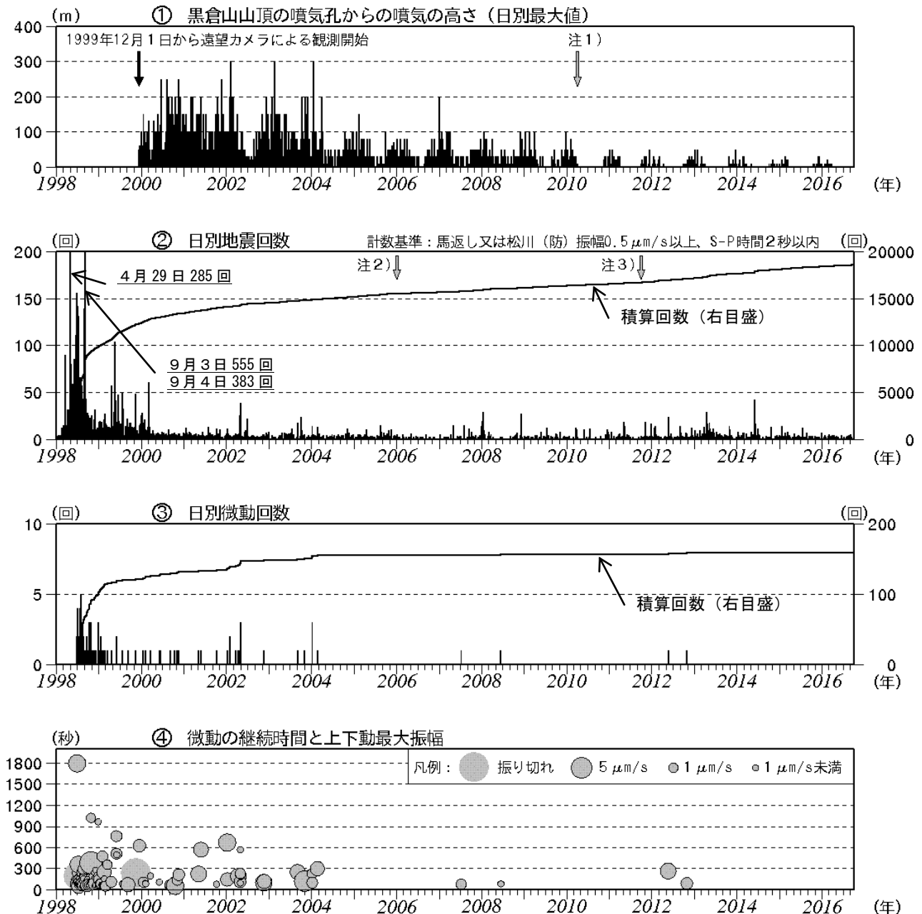
図2 岩手山 火山活動経過図（1998年1月～2016年9月）
