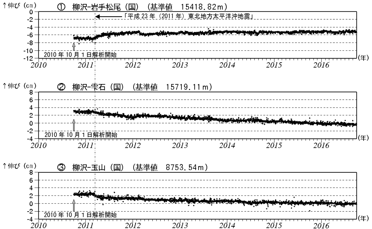
図4 岩手山 GNSS 2) 基線長変化図（2010年10月～2016年9月）
