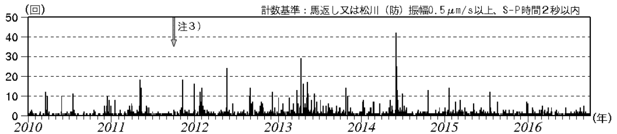
図3 岩手山 日別地震回数（2010年1月～2016年9月）
