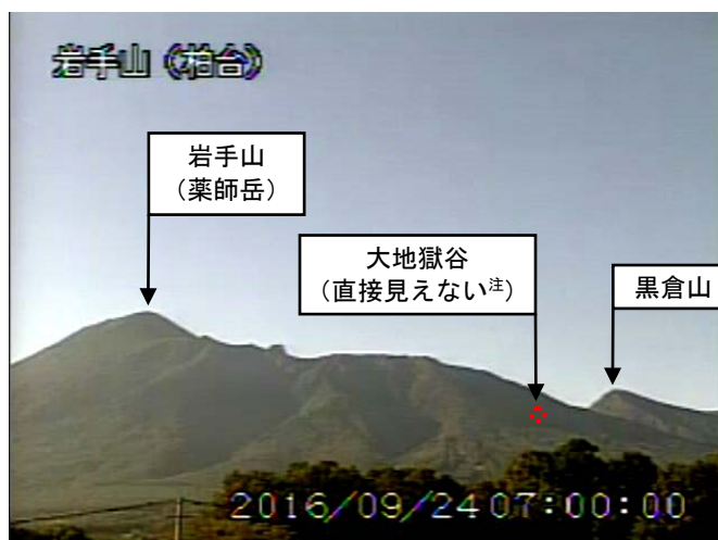
図 1 岩手山 黒倉山の噴気の状況（9 月 24 日）
