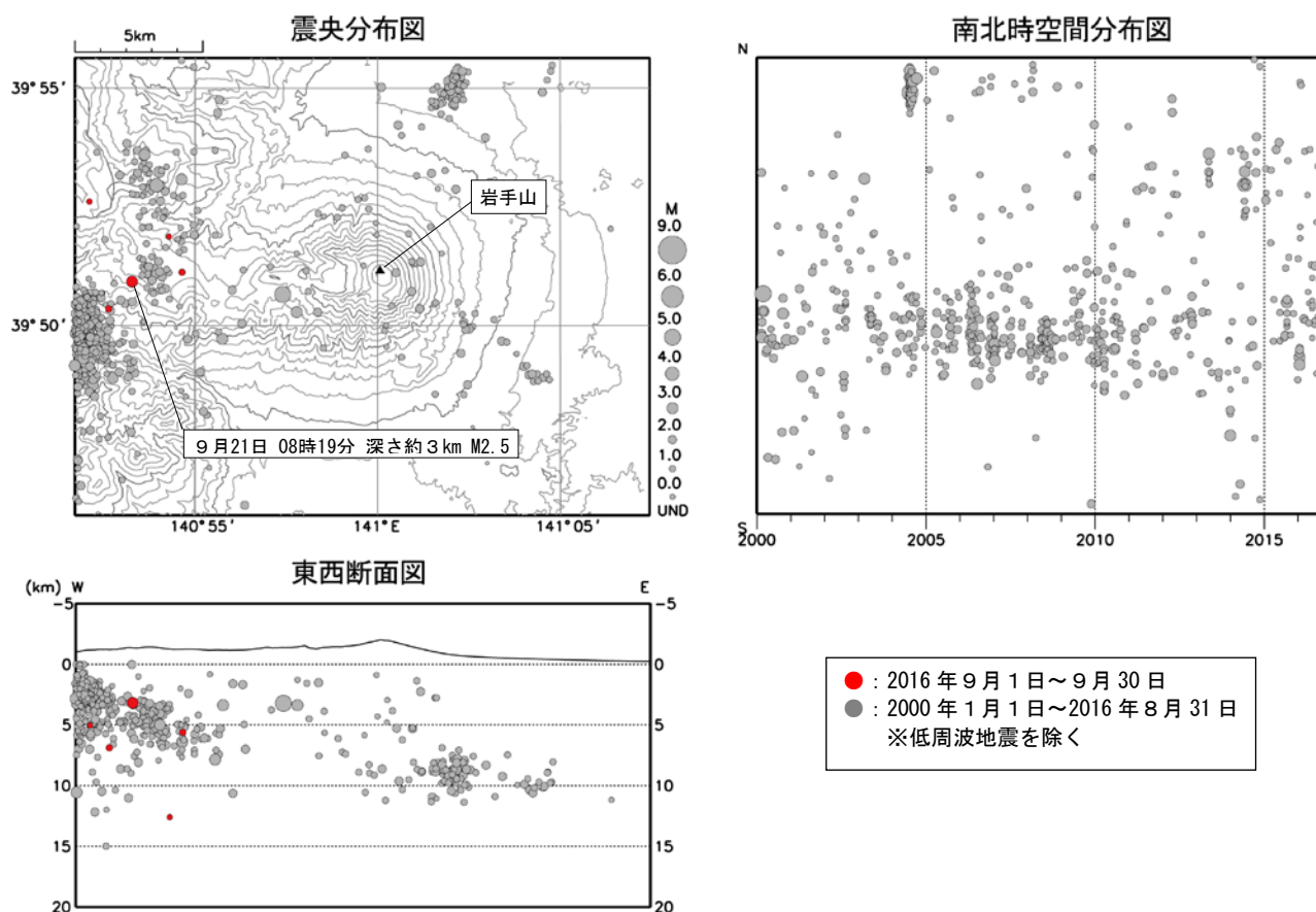
図5 岩手山 広域地震観測網による岩手山周辺の地震活動（2000 年 1 月～2016 年 9 月）
