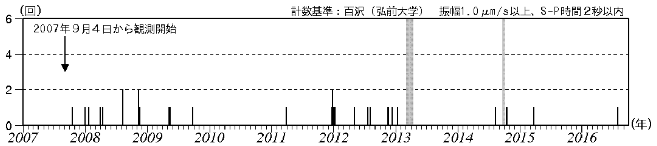
図2 岩木山 日別地震回数（2007年9月～2016年9月）
