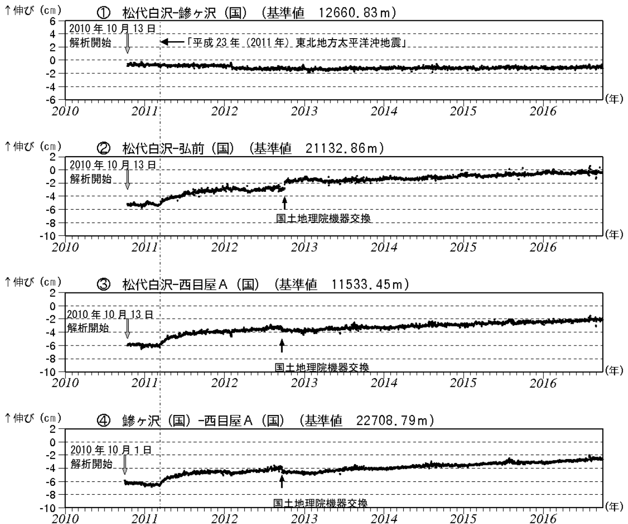
図3 岩木山 GNSS 1) 基線長変化図（2010年10月～2016年9月）
