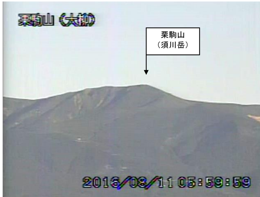
図 1 栗駒山 山頂周辺の状況（8 月 11 日） ・大柳（山頂の南東約 20km）に設置している遠望カメラの映像です。
