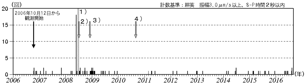
図5 栗駒山 日別地震回数（2006年10月～2016年8月）
