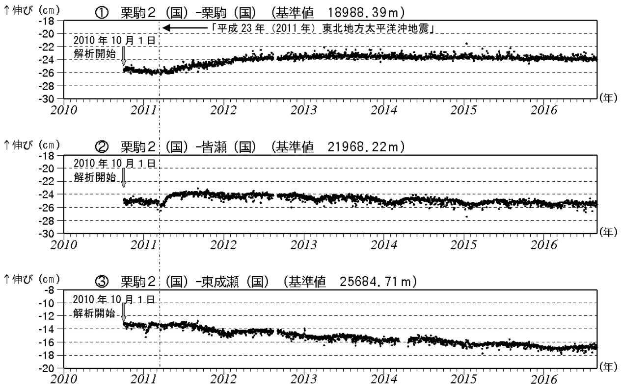
図6 栗駒山 GNSS 2) 基線長変化図（2010年10月～2016年8月）
