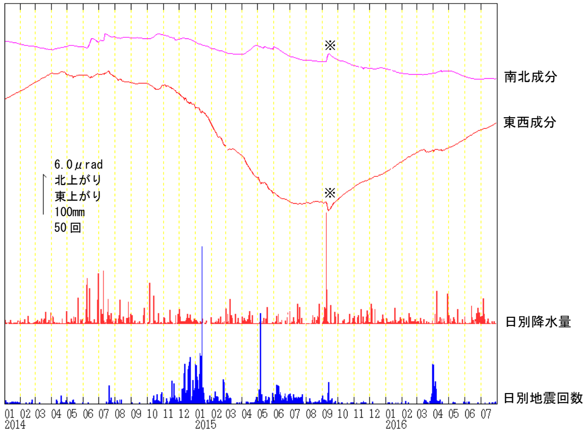
図 9 吾妻山 浄土平観測点での傾斜変動（2014 年 1 月～2016 年 7 月、時間値、潮汐補正あり） ・ 1 \mu rad（マイクロラジアン）は、1 km 先が 1 mm 上下するような変化量です。 ・ 2015 年 6 月頃までみられていた西南西側（火口方向側）上がりの変動は、2015 年 7 月頃から停滞していましたが、2015 年 9 月頃から西側下がり傾向となっています。 ・ 日別降水量は鷲倉地域気象観測所で観測された値です。 ※ 「平成 27 年 9 月関東・東北豪雨」による変動です。
