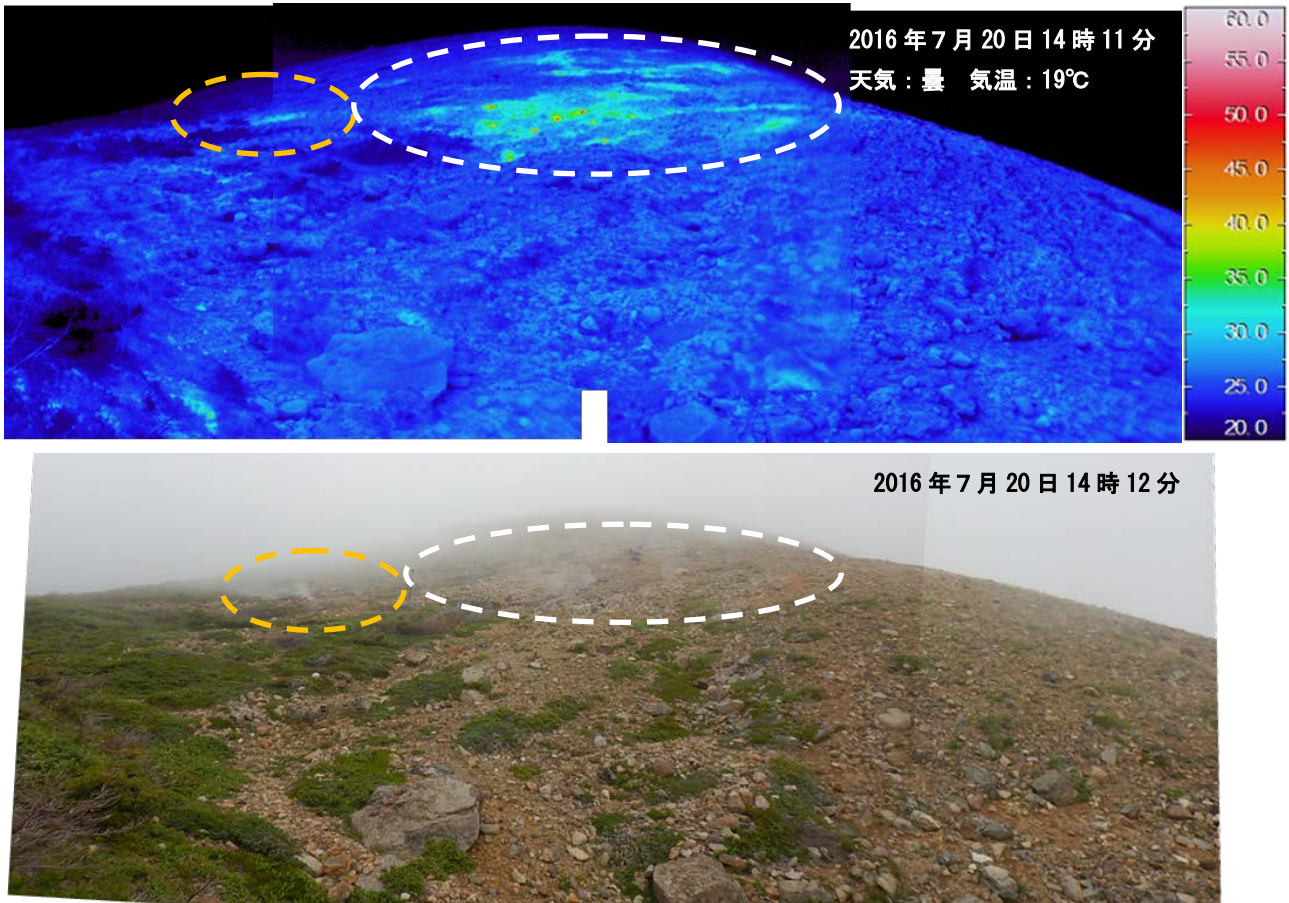
図5 吾妻山 大穴火口北西の状況と地表面温度分布
