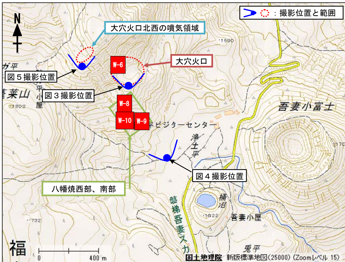
図2 吾妻山 噴気や地熱域の分布図及び写真と地表面温度分布 3) 撮影位置
