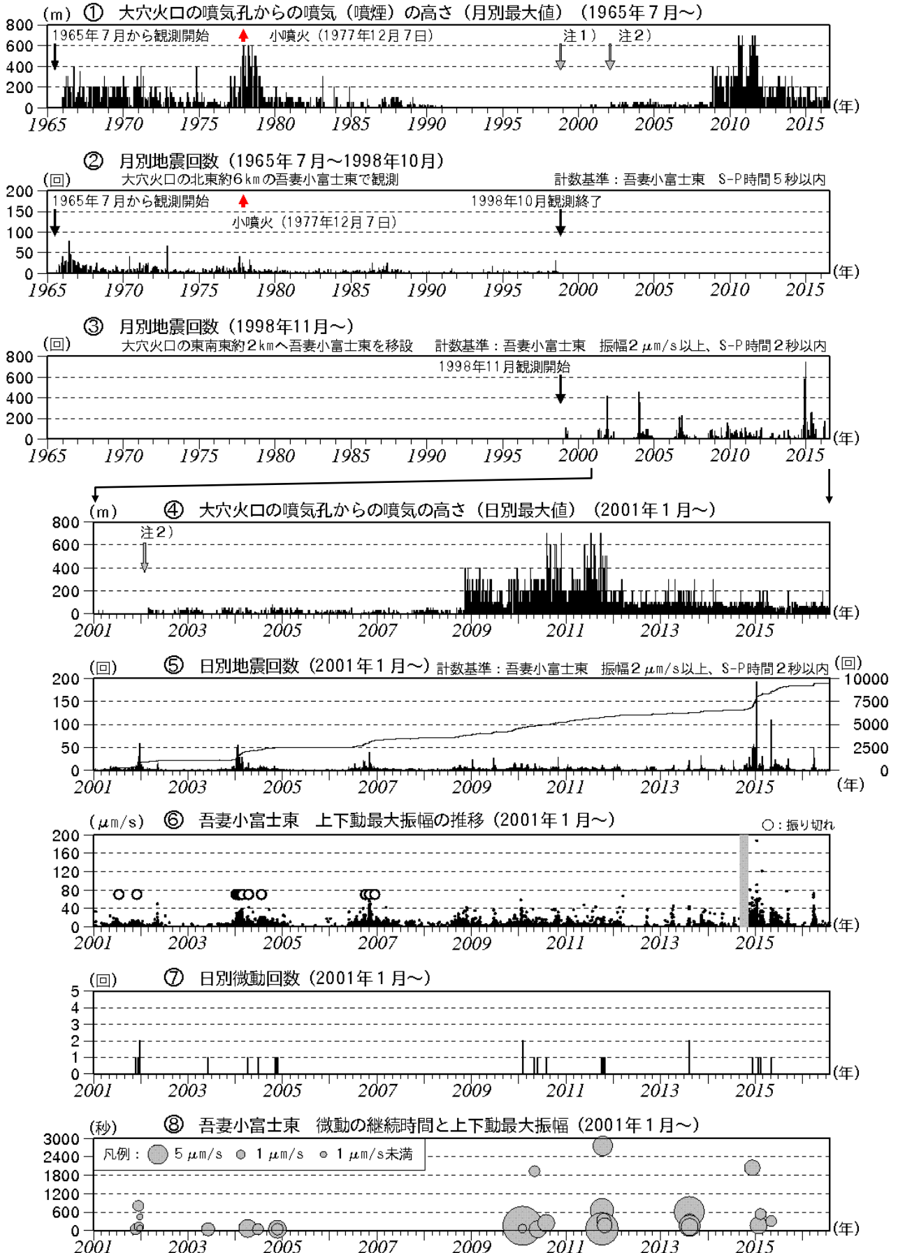
図7 吾妻山 火山活動経過図 (1965年7月~2016年7月)
