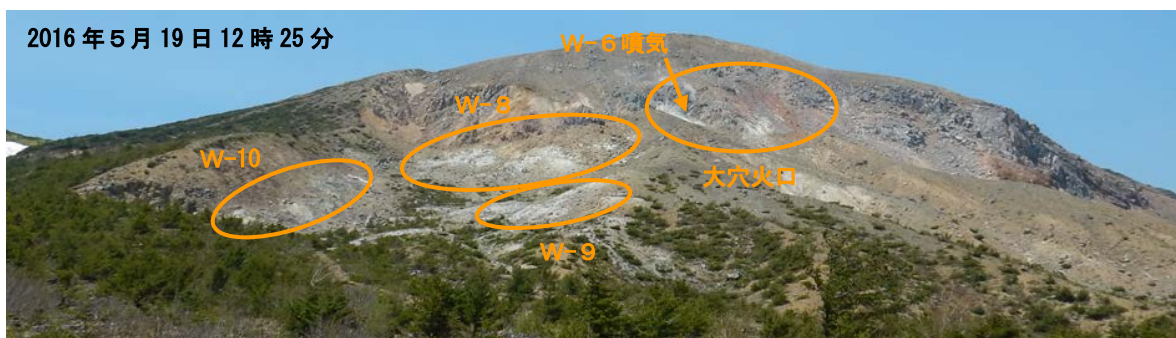
図4 吾妻山 大穴火口の状況と地表面温度分布
