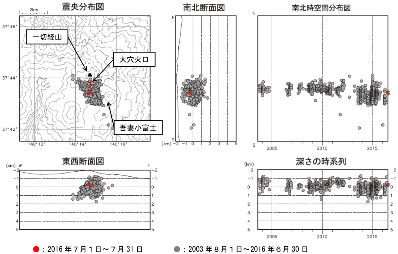
● : 2016 年 7 月 1 日～7 月 31 日 ● : 2003 年 8 月 1 日～2016 年 6 月 30 日 図 8 吾妻山 地震活動（2003 年 8 月～2016 年 7 月） ・ 2012 年 12 月 1 日以降、観測点の移設更新の影響により、震源がやや南側に分布する傾向がみられます。
