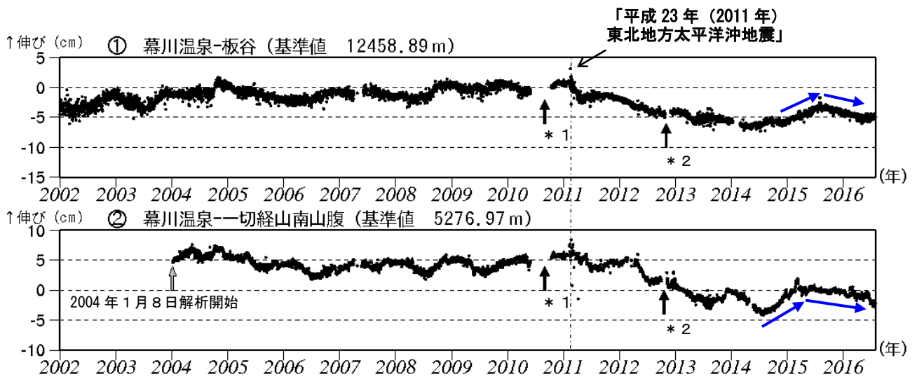
図 11-1 吾妻山 GNSS 基線長変化図 (2002 年 1 月～2016 年 7 月)
