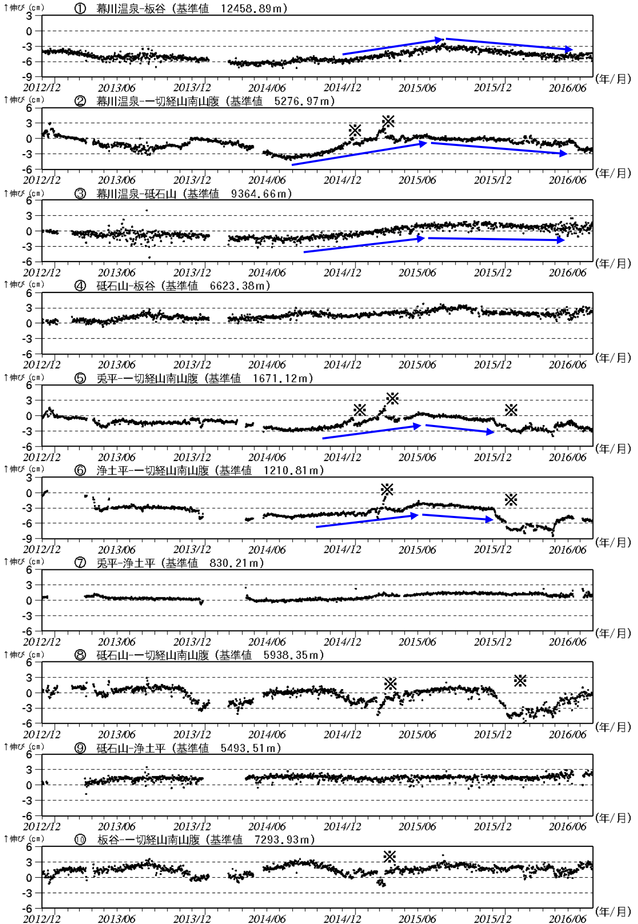
図 11-2 吾妻山 GNSS 基線長変化図 (2012 年 12 月～2016 年 7 月)
