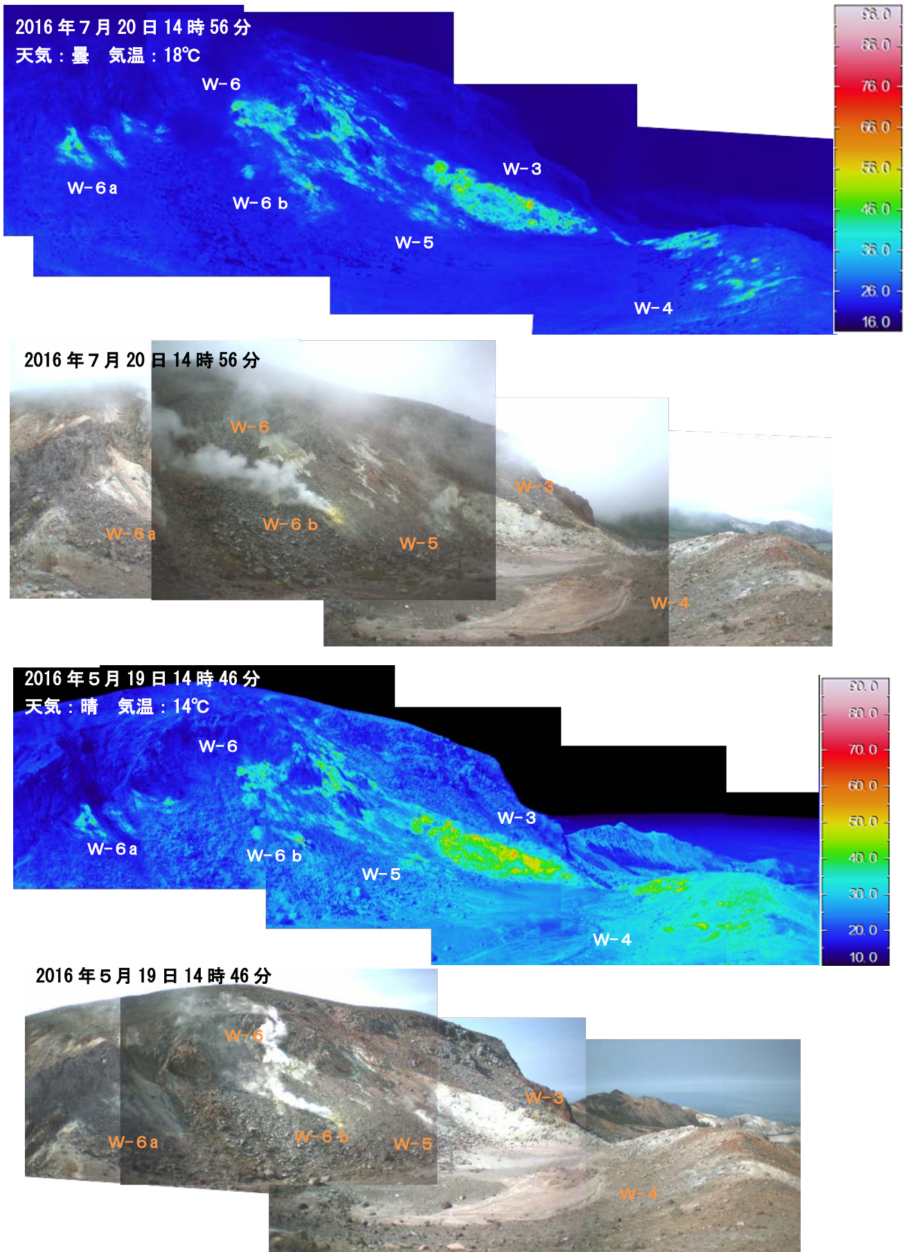
図3 吾妻山 大穴火口の状況と地表面温度分布
