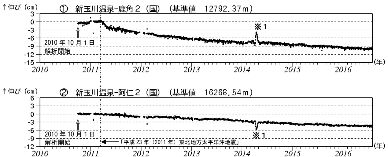
図4 秋田焼山 GNSS 1) 基線長変化図（2010年10月～2016年7月）
