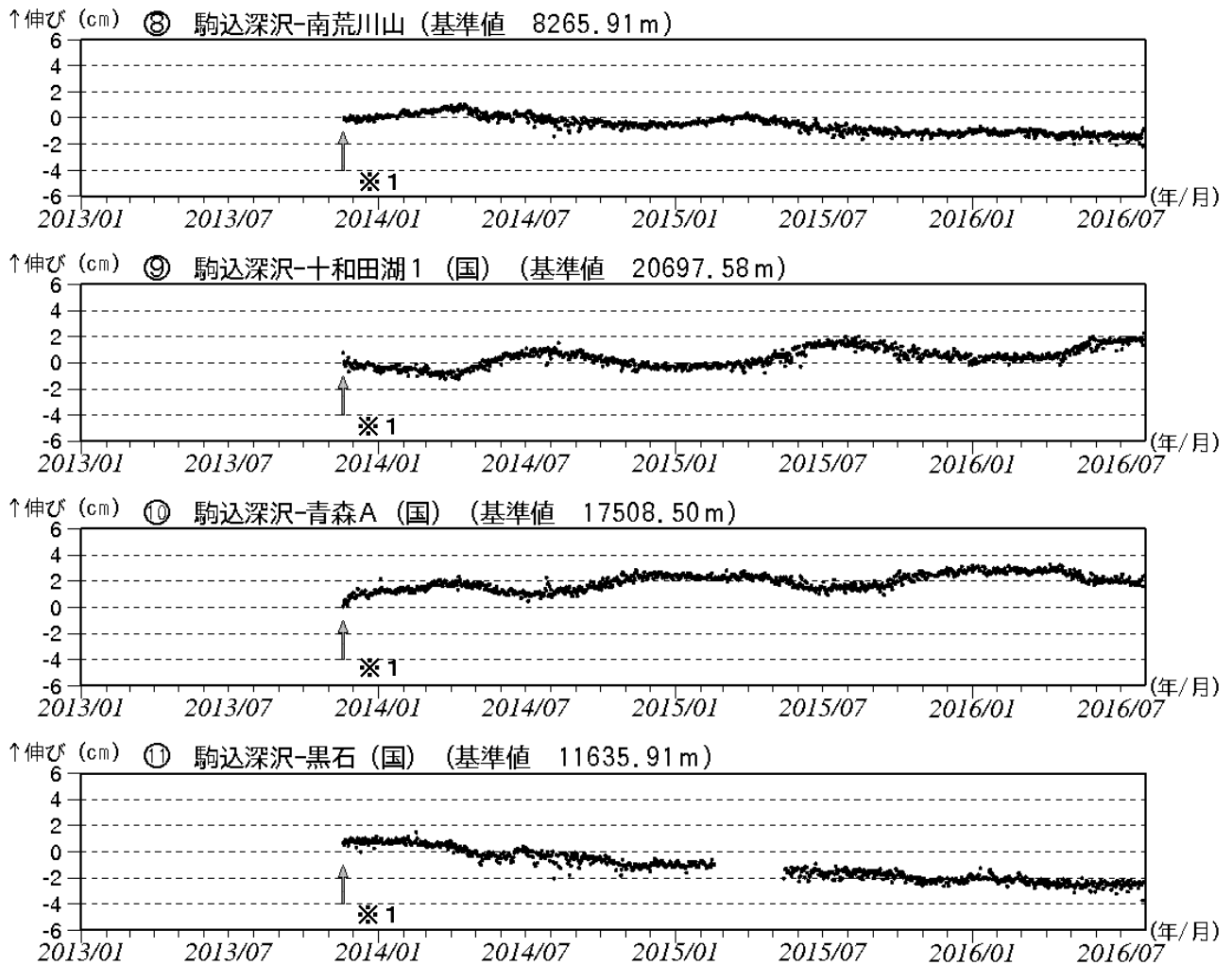
図 2-2 八甲田山 GNSS 基線長変化図 (2013 年 1 月～2016 年 7 月)
