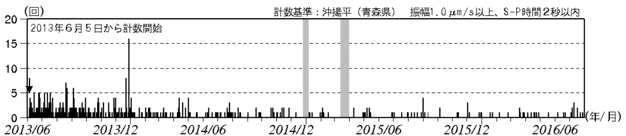
図 1 八甲田山 日別地震回数（2013 年 6 月～2016 年 7 月）
