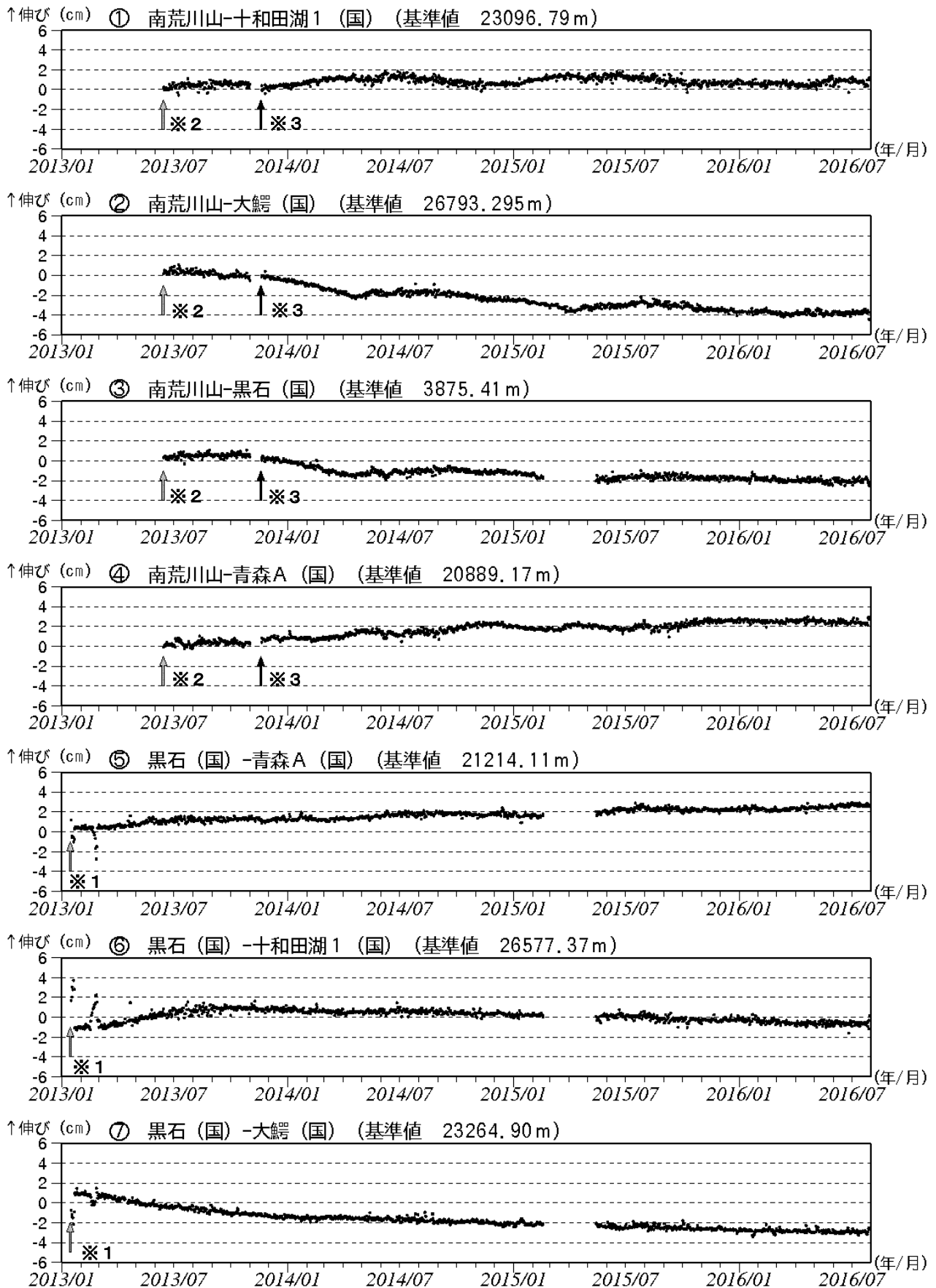
図 2-1 八甲田山 GNSS 1) 基線長変化図 (2013 年 1 月～2016 年 7 月)
