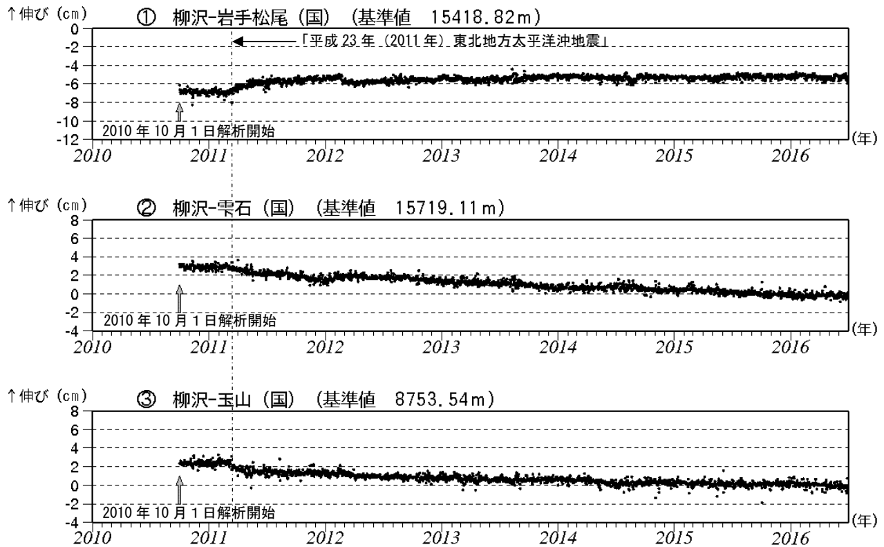
図 5 岩手山 GNSS 1) 基線長変化図 (2010 年 10 月～2016 年 6 月)
