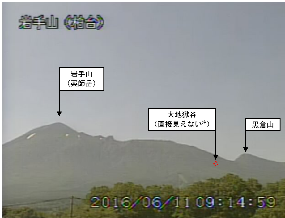
図1 岩手山 黒倉山の噴気の状態（6月11日）
