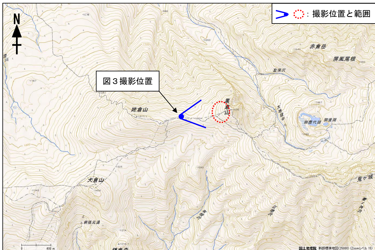
図2 岩手山 黒倉山の写真と地表面温度分布 1) 撮影位置
