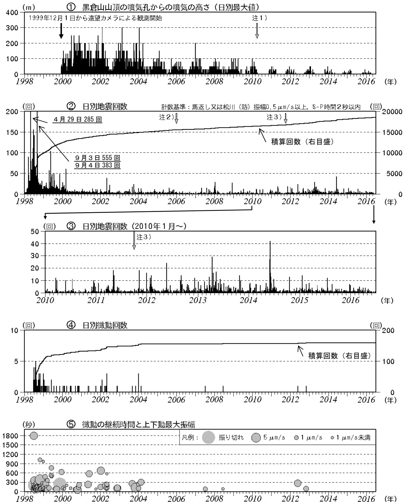
図4 岩手山 火山活動経過図（1998年1月～2016年6月）
