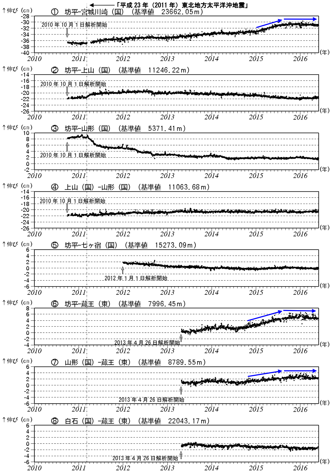
図 5-1 蔵王山 GNSS 基線長変化図 (2010 年 10 月～2016 年 5 月)
