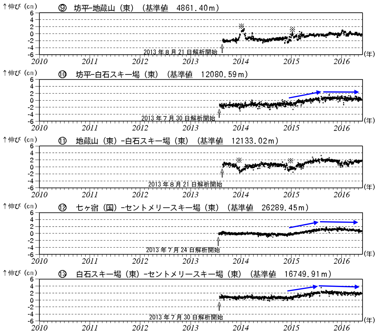
図 5-2 蔵王山 GNSS 基線長変化図 (2010 年 10 月～2016 年 5 月)
