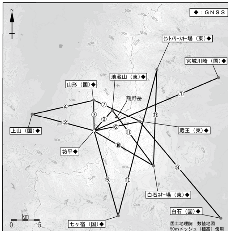
图7 藏王山 GNSS 観測点配置図
