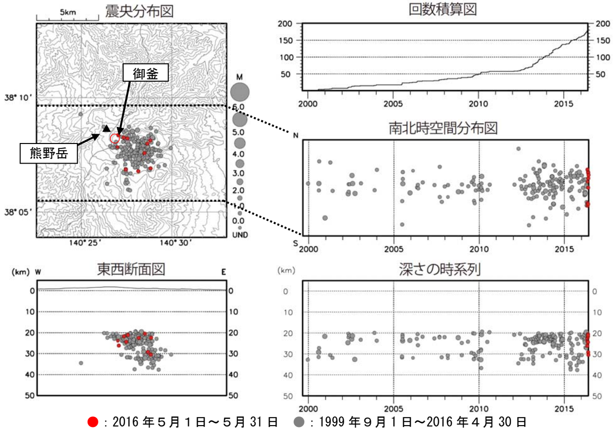
図 3 蔵王山 広域地震観測網による深部低周波地震活動（1999 年 9 月～2016 年 5 月）
