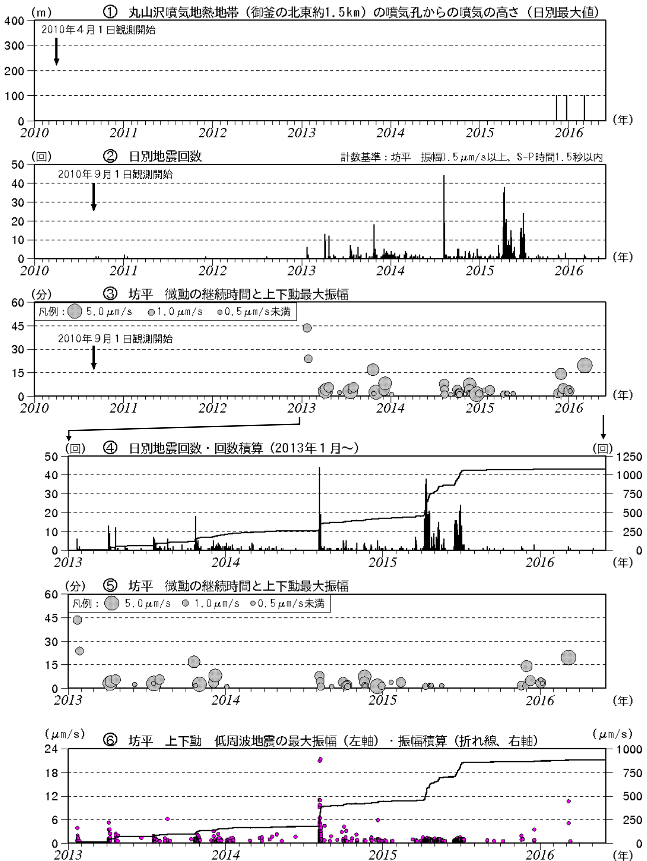
図2 蔵王山 火山活動経過図（2010年4月～2016年5月）
