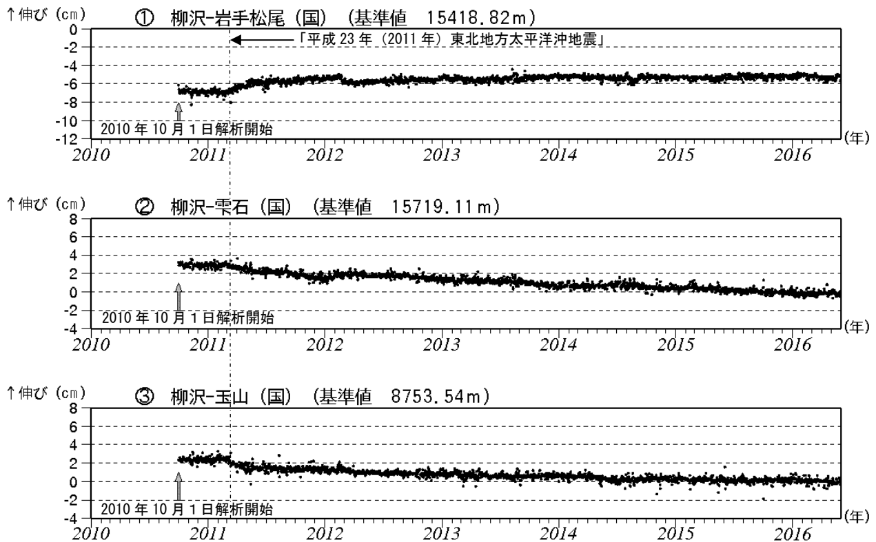
図3 岩手山 GNSS 1) 基線長変化図 (2010 年 10 月～2016 年 5 月)
