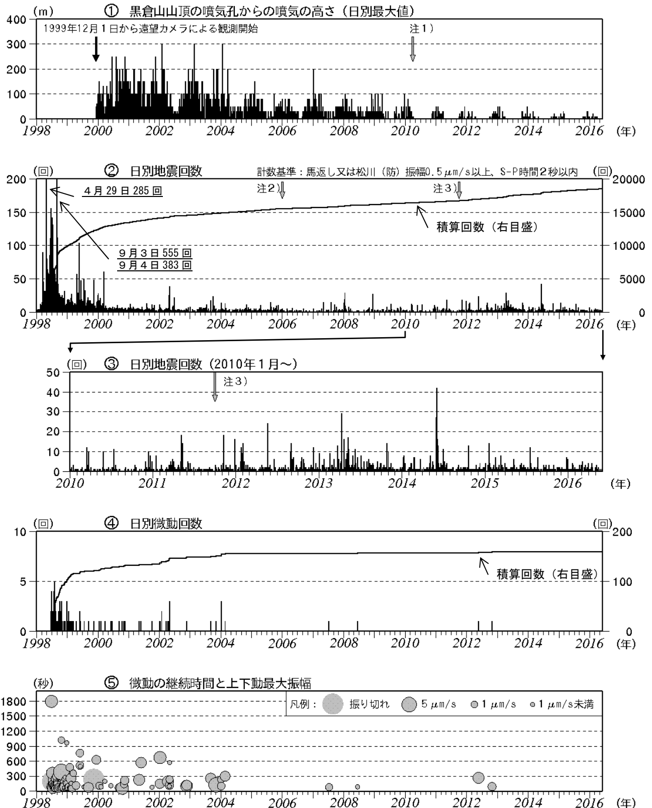
図2 岩手山 火山活動経過図（1998年1月～2016年5月）
