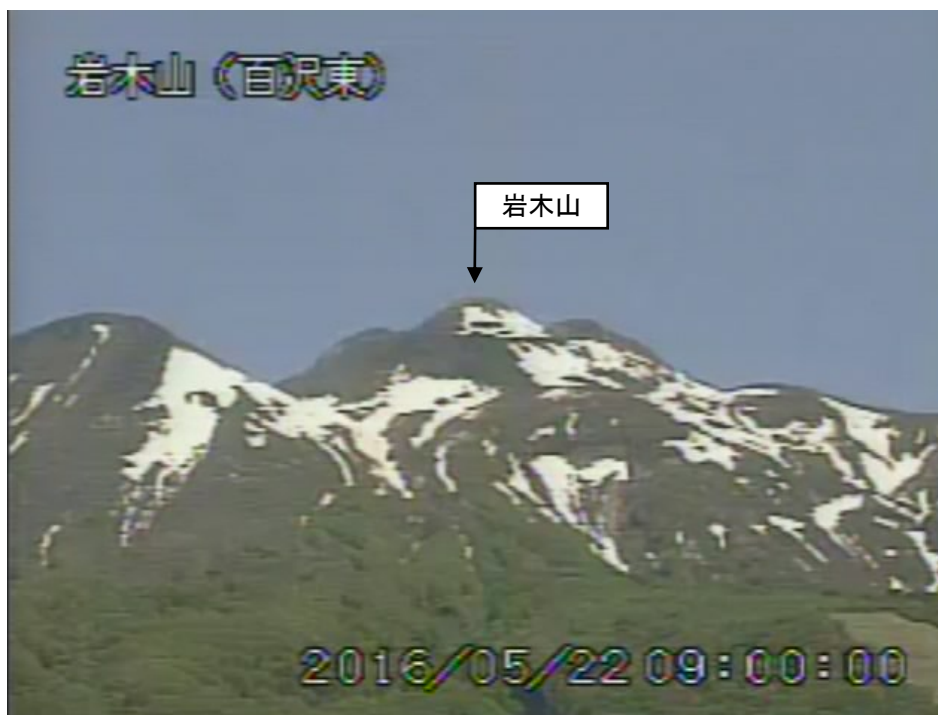
図 1 岩木山 山頂部の状況（5 月 22 日）
