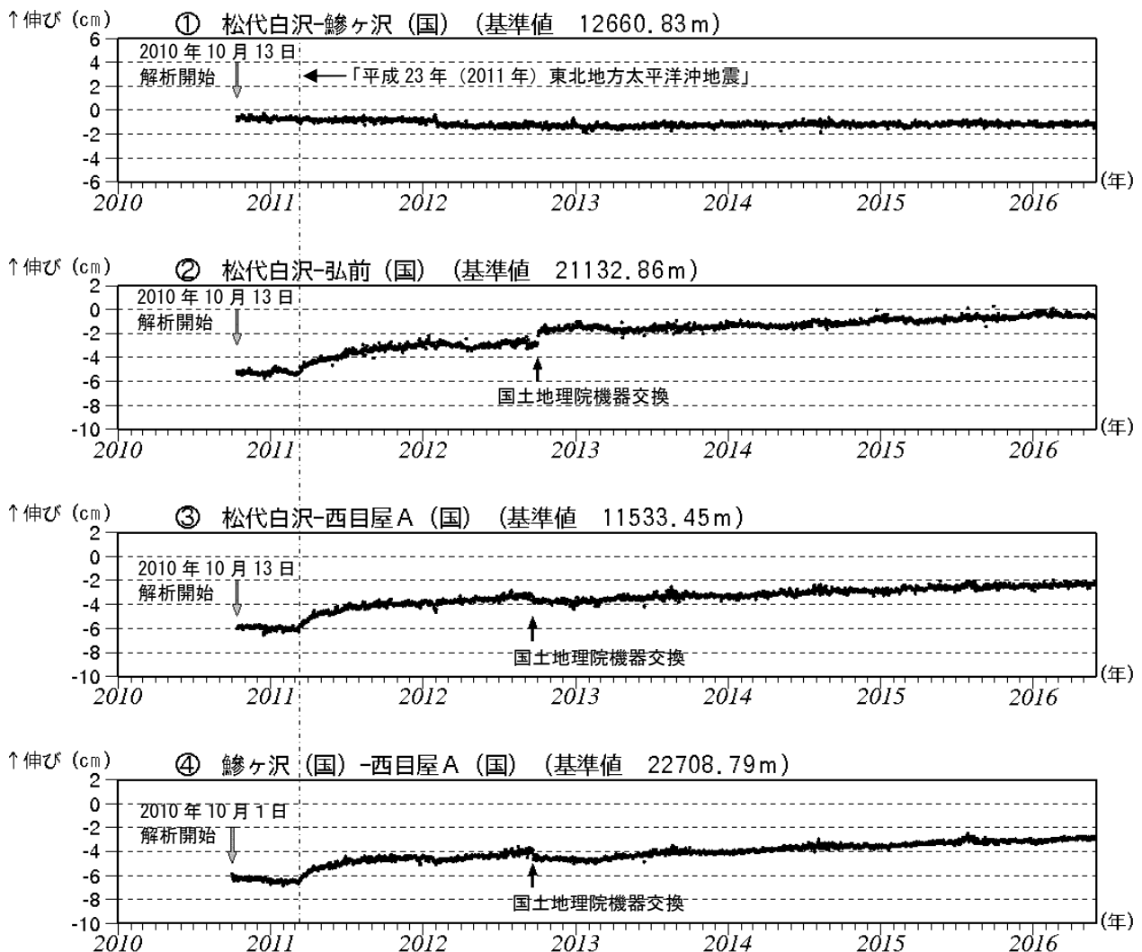
図3 岩木山 GNSS 1) 基線長変化図（2010年10月～2016年5月）
