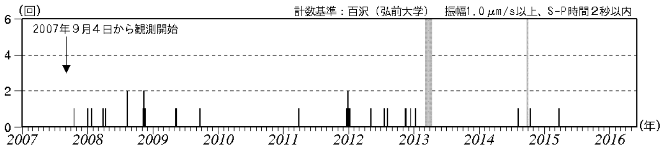
図2 岩木山 日別地震回数（2007年9月～2016年5月）
