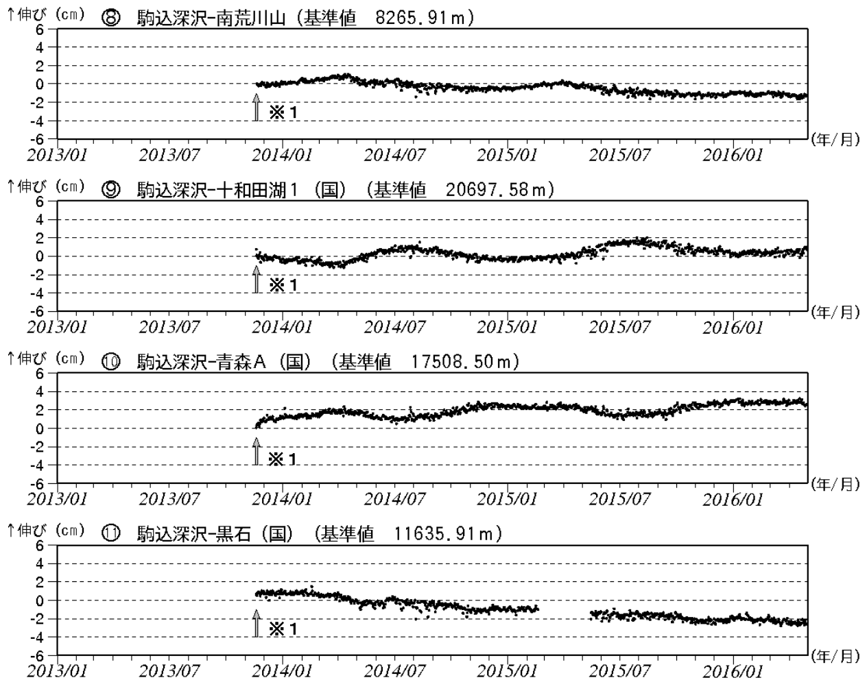
図 2-2 八甲田山 GNSS 基線長変化図 (2013 年 1 月～2016 年 4 月)
