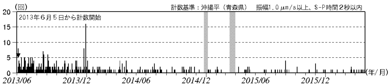
図 1 八甲田山 日別地震回数（2013 年 6 月～2016 年 4 月）
