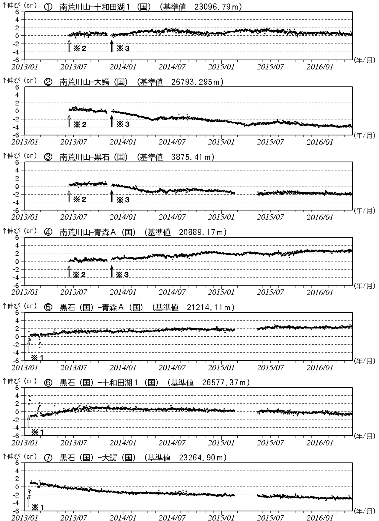
図 2-1 八甲田山 GNSS 1) 基線長変化図 (2013 年 1 月～2016 年 4 月)
