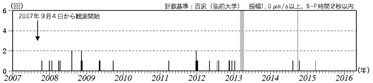
図2 岩木山 日別地震回数（2007年9月～2016年4月）
