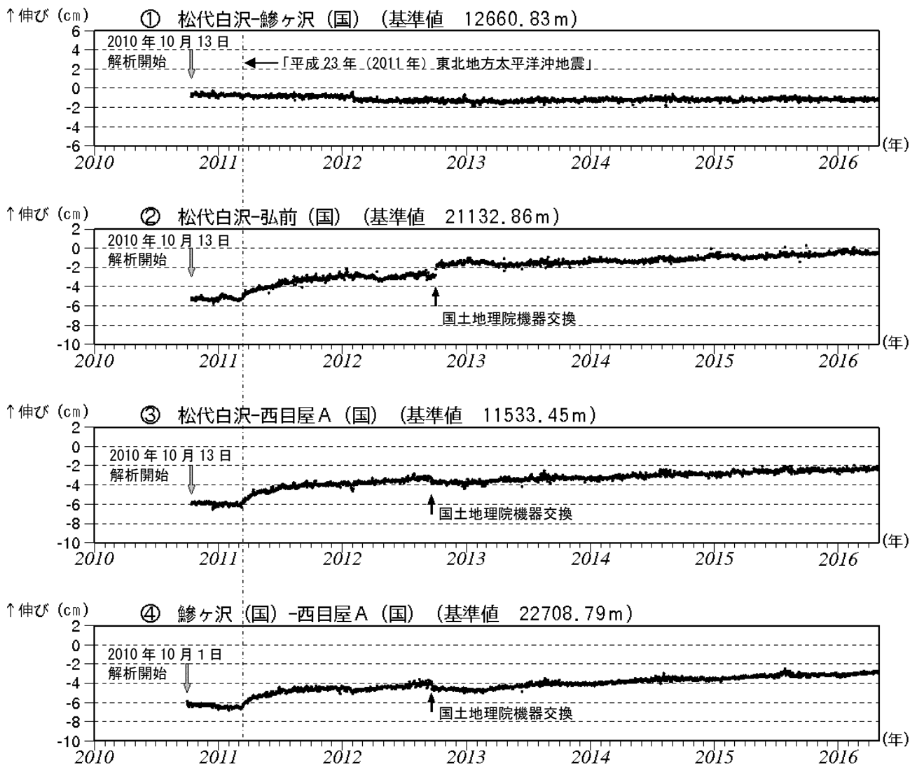
図3 岩木山 GNSS 1) 基線長変化図（2010年10月～2016年4月）
