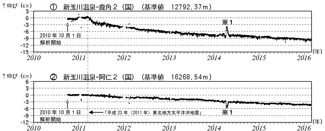
図 3 秋田焼山 GNSS 1) 基線長変化図（2010 年 10 月～2016 年 2 月）
