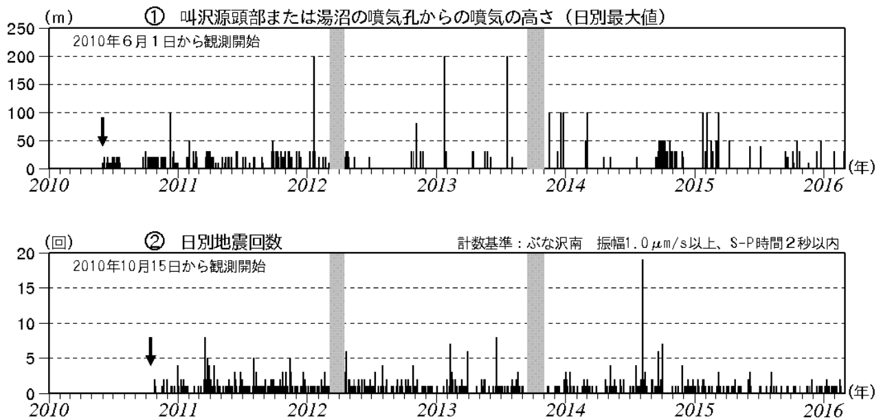
図 2 秋田焼山 火山活動経過図（2010 年 6 月～2016 年 2 月）
