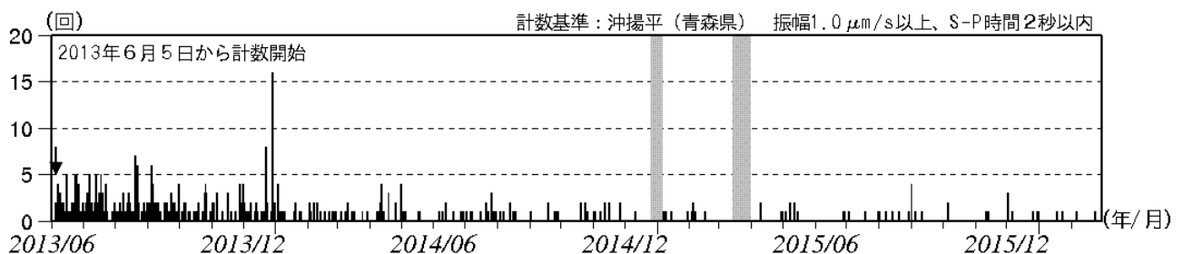
図 1 八甲田山 日別地震回数（2013 年 6 月～2016 年 2 月）
