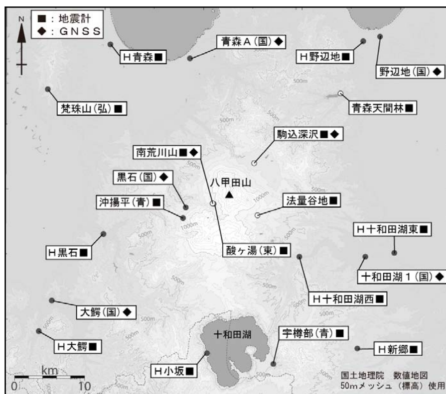
図4 八甲田山 GNSS観測点配置図
