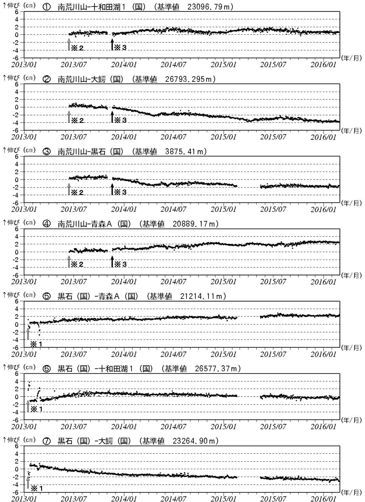
図2-① 八甲田山 GNSS 基線長変化図 (2013 年 1 月～2016 年 2 月)
