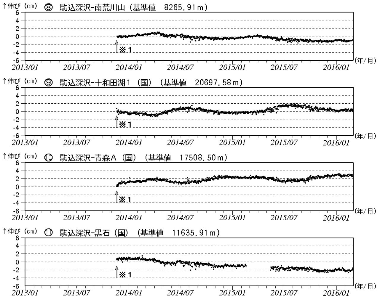
図2-② 八甲田山 GNSS 基線長変化図 (2013 年 1 月～2016 年 2 月)
