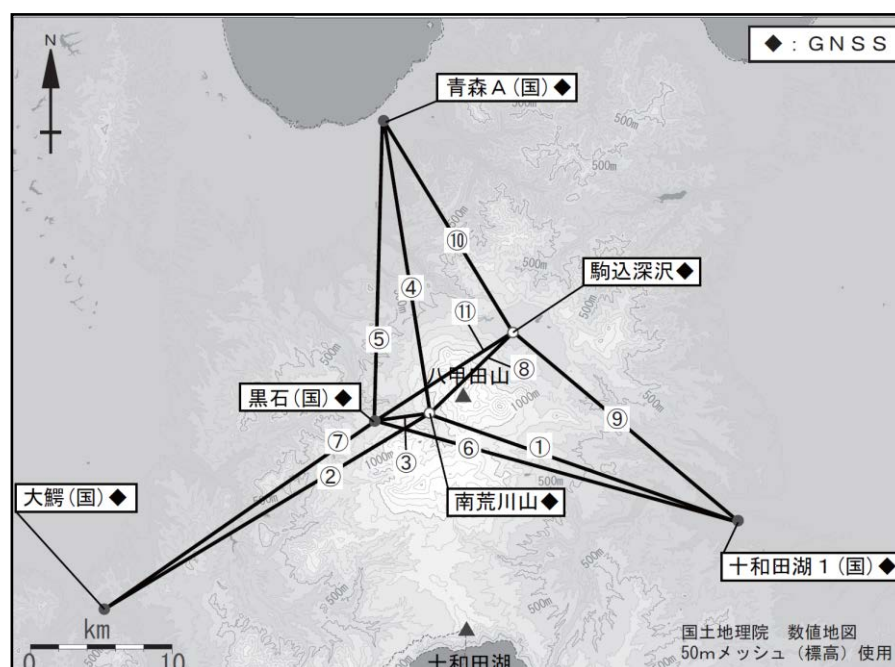
図3 八甲田山 観測点配置図
