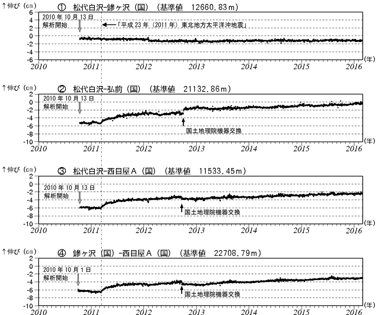
図3 岩木山 GNSS 1) 基線長変化図（2010年10月～2016年2月）
