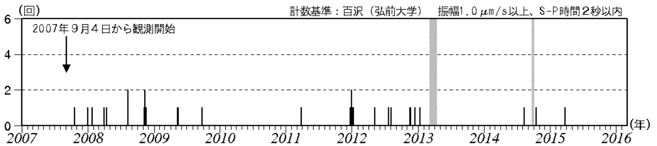
図2 岩木山 日別地震回数（2007年9月～2016年2月）
