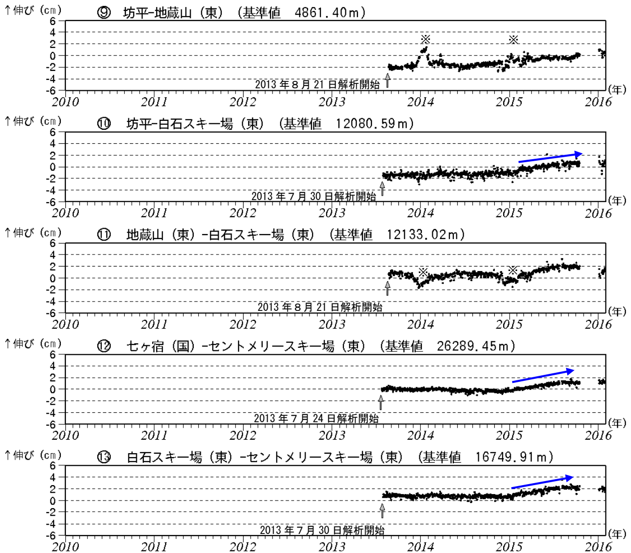
図 6-② 蔵王山 GNSS 基線長変化図 (2010 年 10 月～2016 年 1 月)
