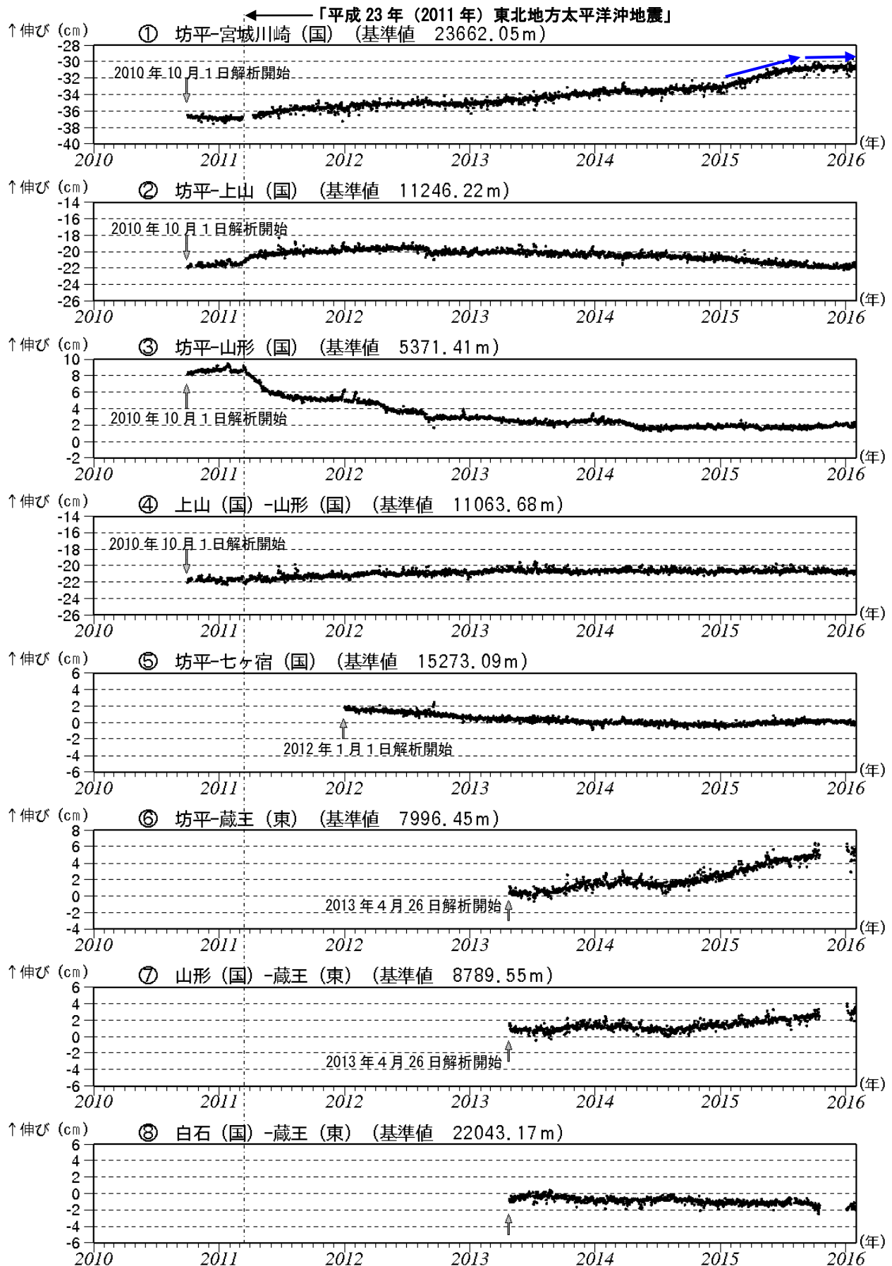
図 6-① 蔵王山 GNSS 基線長変化図 (2010 年 10 月～2016 年 1 月)
