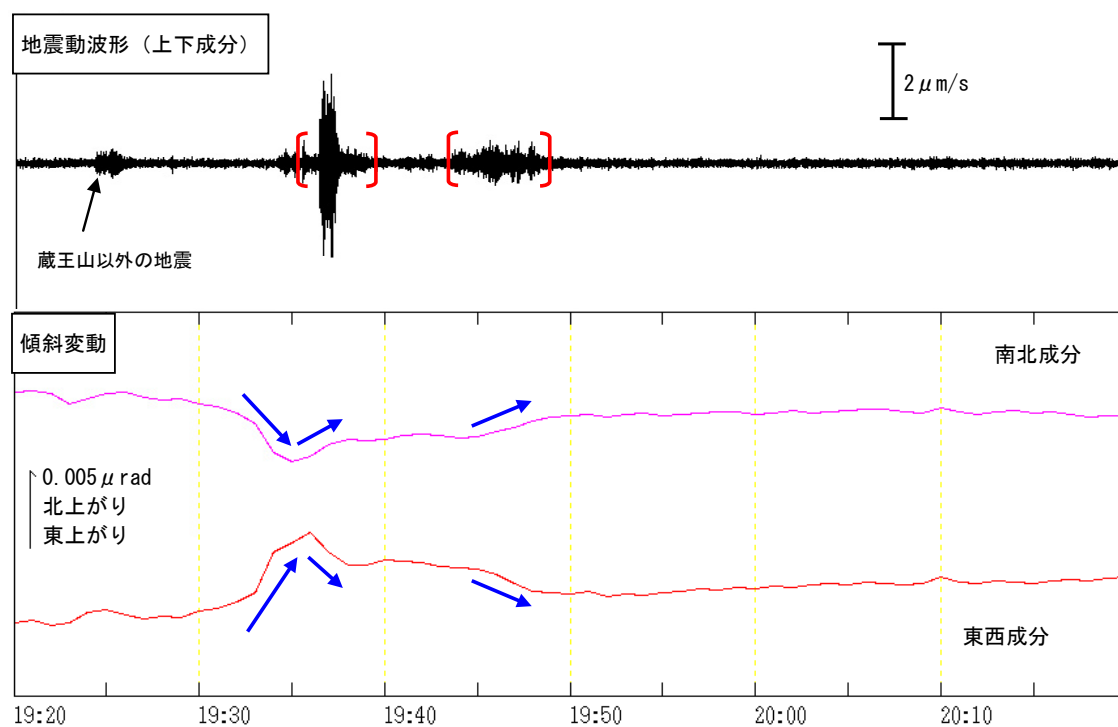
図5 蔵王山 坊平観測点での火山性微動波形及び傾斜変動 (2016年1月1日19時20分～20時20分)
