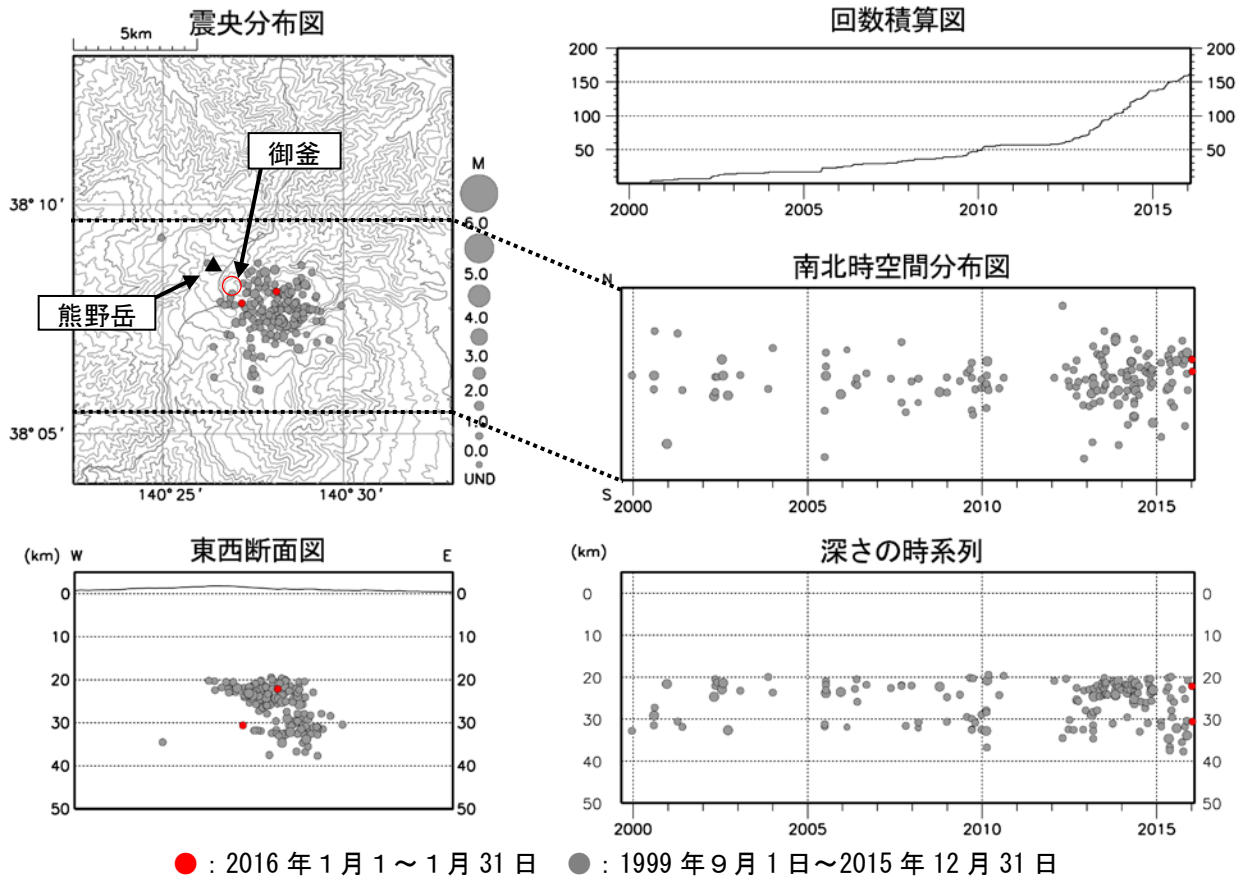
図3 蔵王山 広域地震観測網による深部低周波地震活動（1999 年 9 月～2016 年 1 月）
