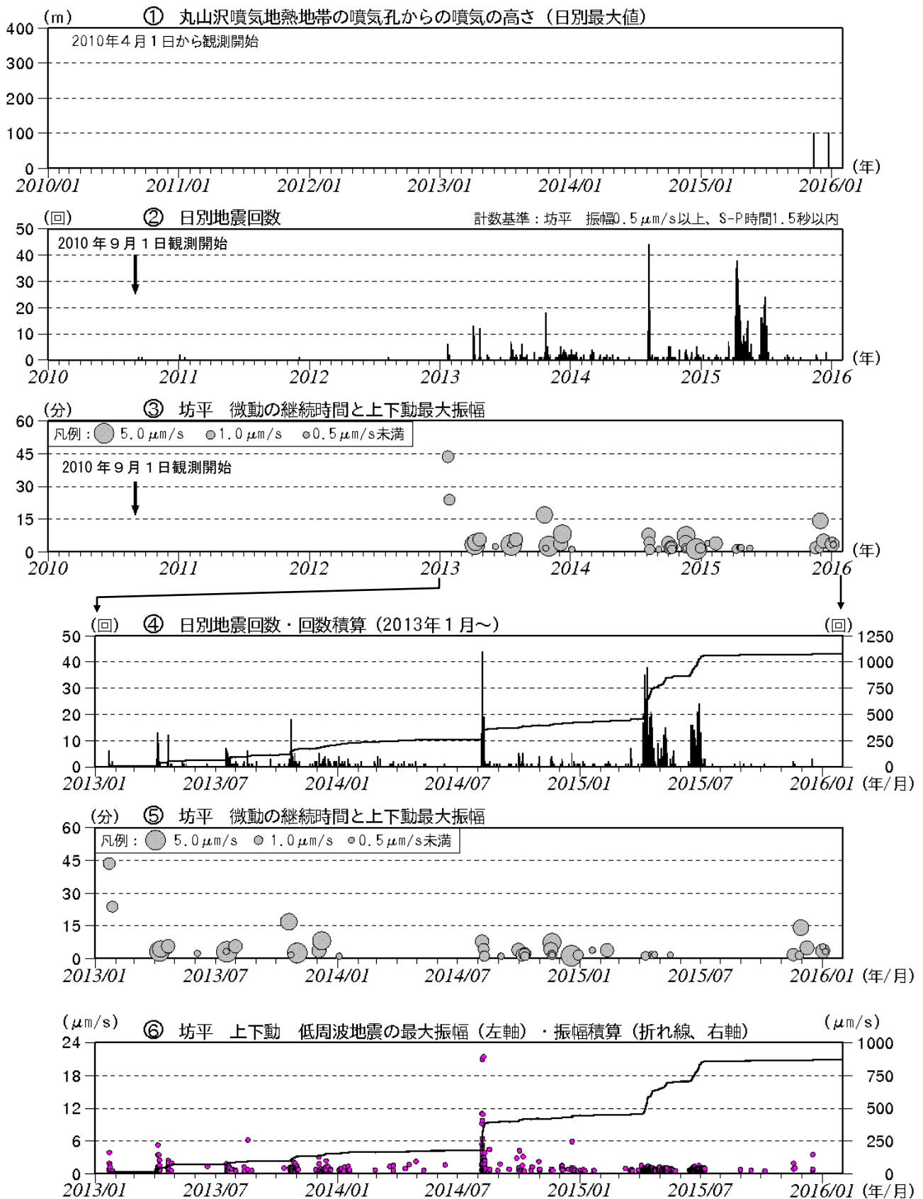
図2 蔵王山 火山活動経過図（2010年9月～2016年1月）
