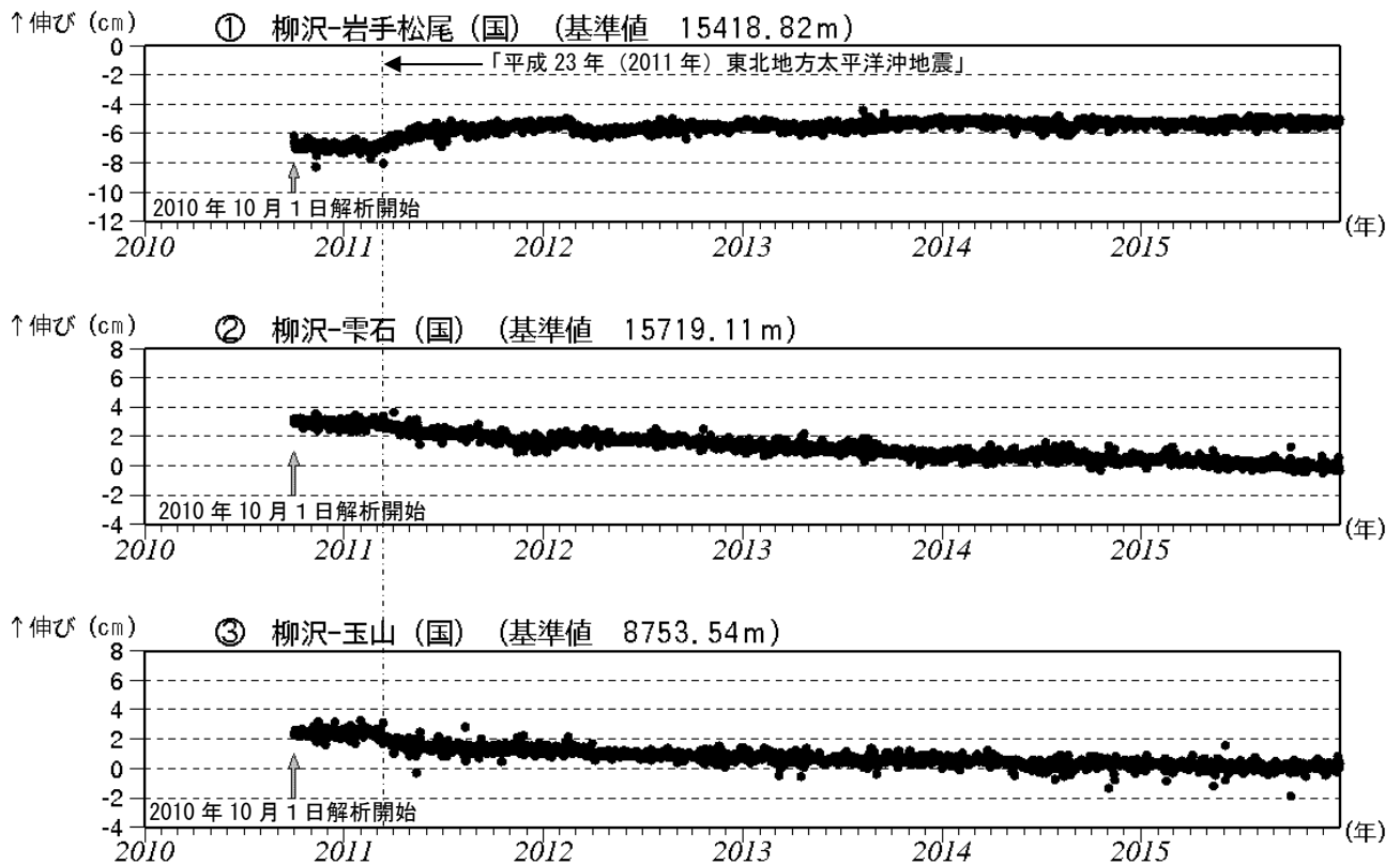
図3 岩手山 GNSS 1) 基線長変化図 (2010 年 10 月～2015 年 12 月)
