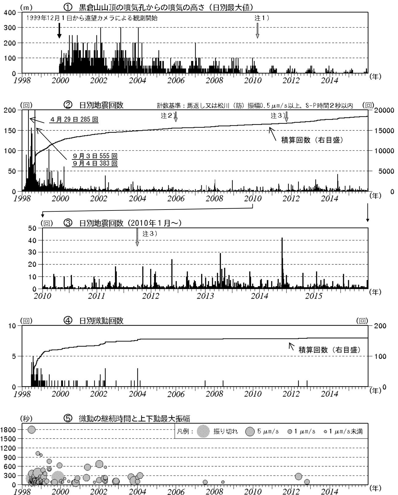
図2 岩手山 火山活動経過図（1998年1月～2015年12月）
