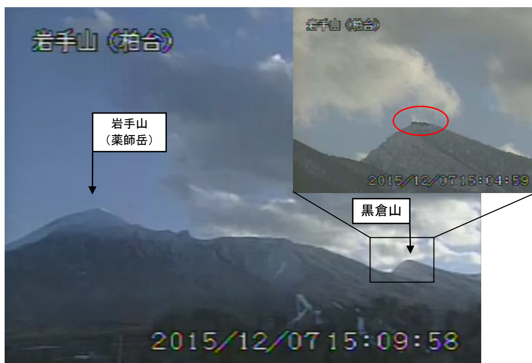
図 1 岩手山 黒倉山の噴気の状況（12 月 7 日）
