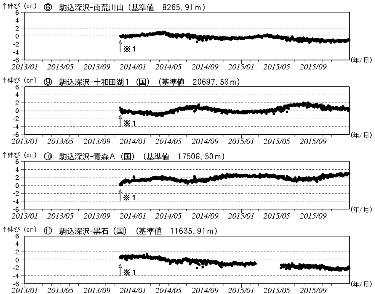
図2-② 八甲田山 GNSS 基線長変化図 (2013 年 1 月～2015 年 12 月)
