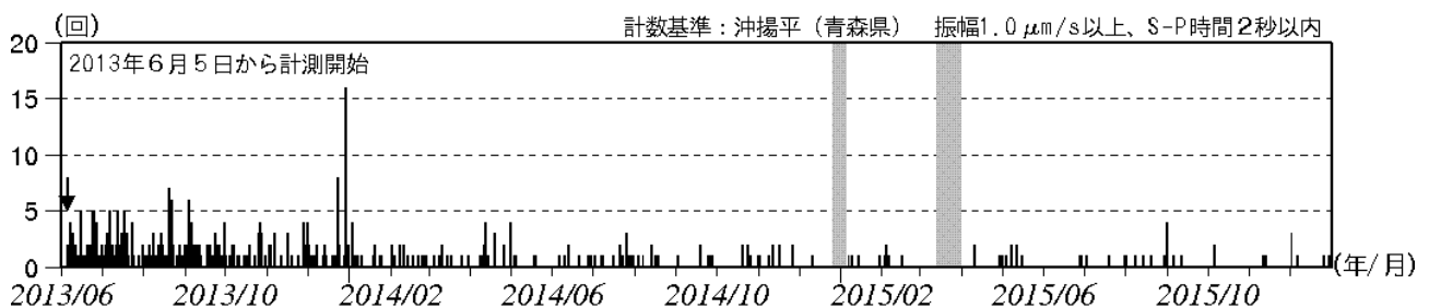
図 1 八甲田山 日別地震回数（2013 年 6 月～2015 年 12 月）
