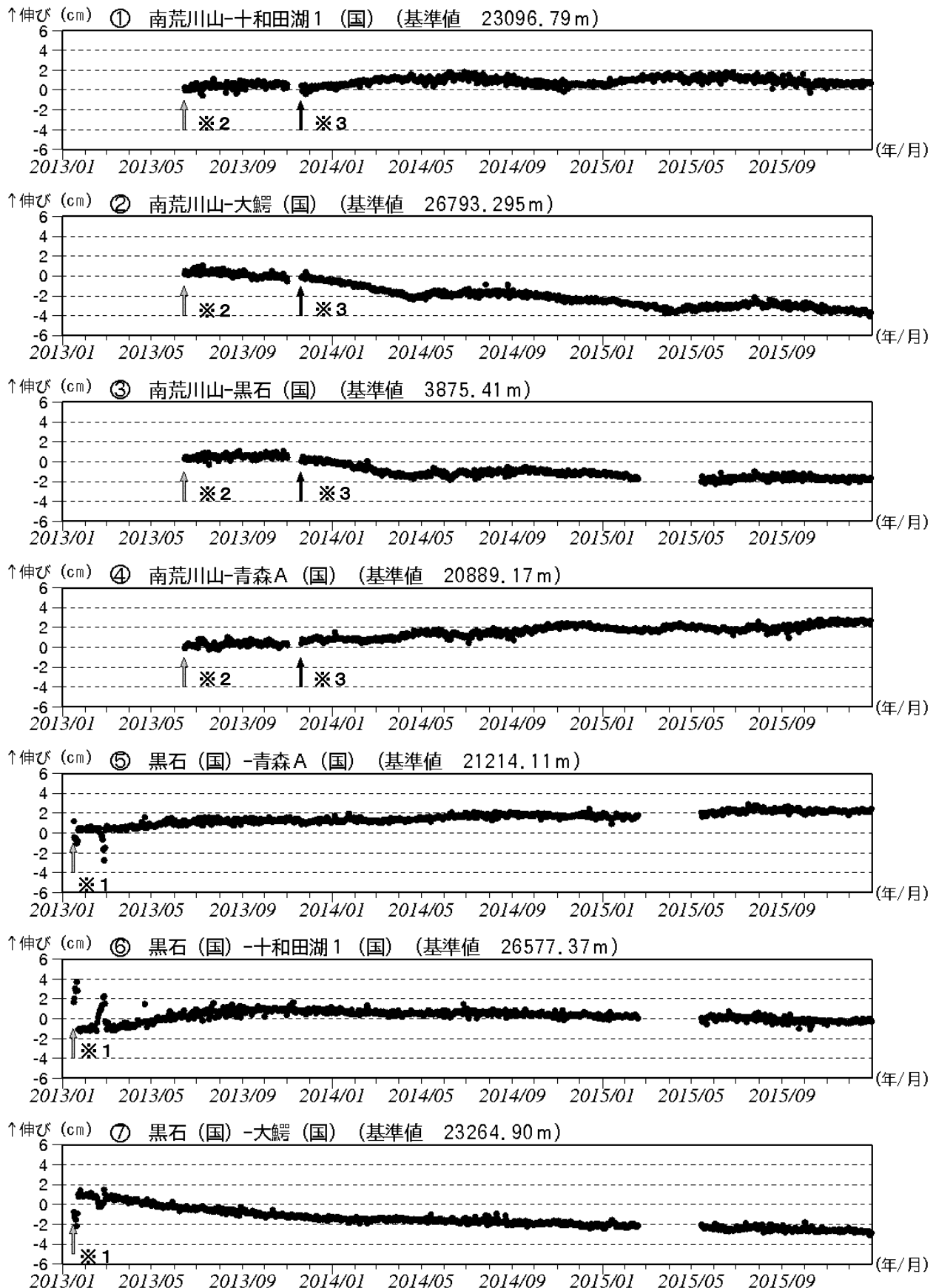
図 2-① 八甲田山 GNSS 基線長変化図 (2013 年 1 月～2015 年 12 月)
