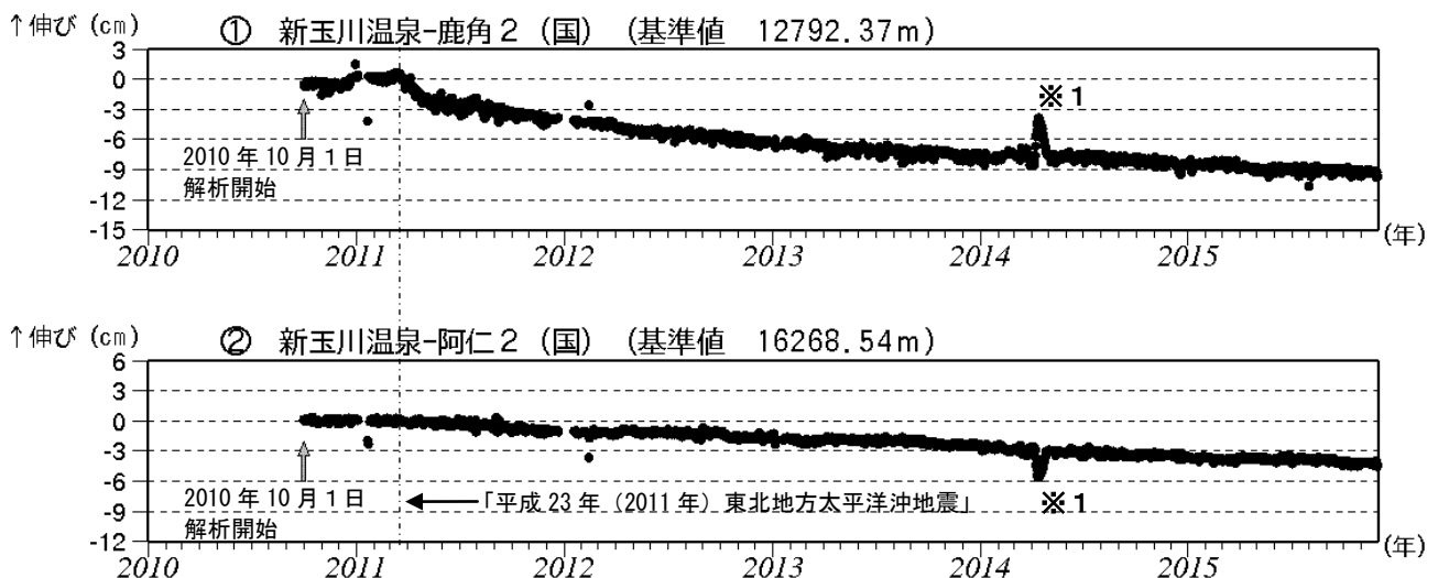
図 3 秋田焼山 GNSS 1) 基線長変化図（2010 年 10 月～2015 年 11 月）
