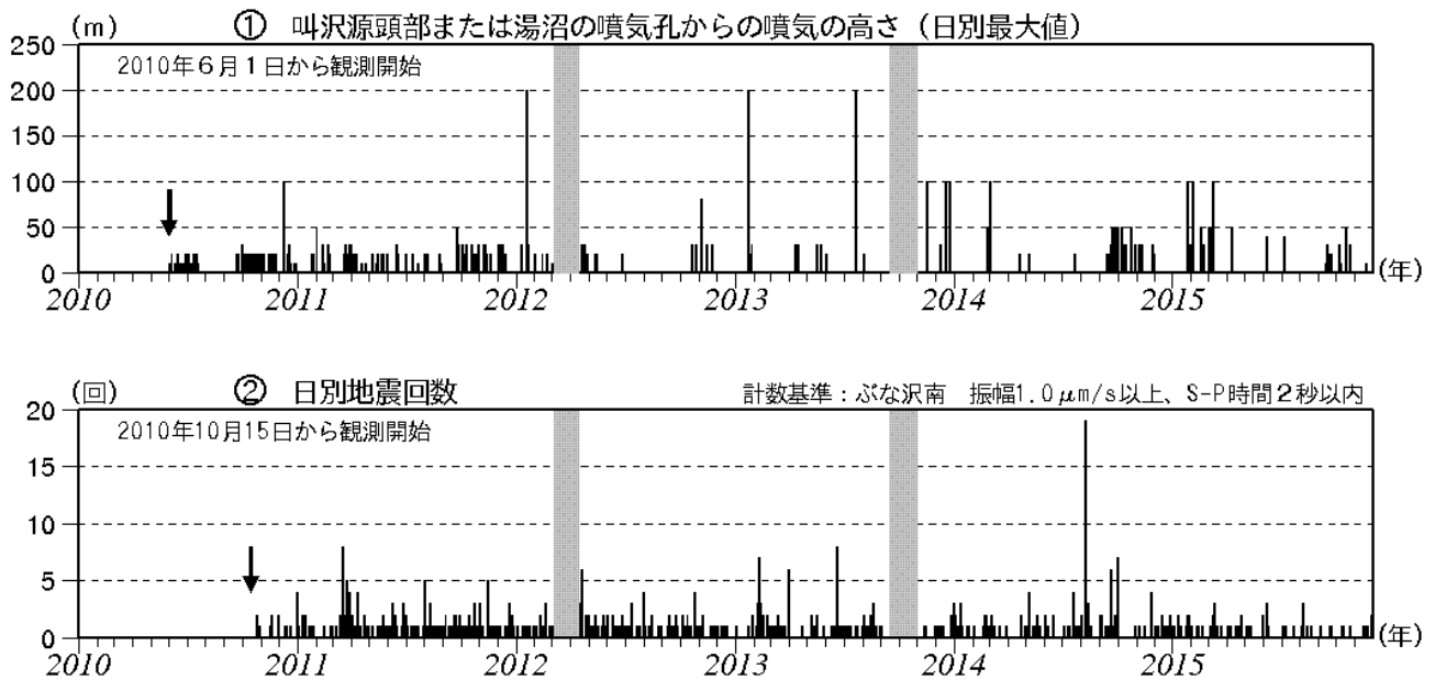
図 2 秋田焼山 火山活動経過図（2010 年 6 月～2015 年 11 月）
