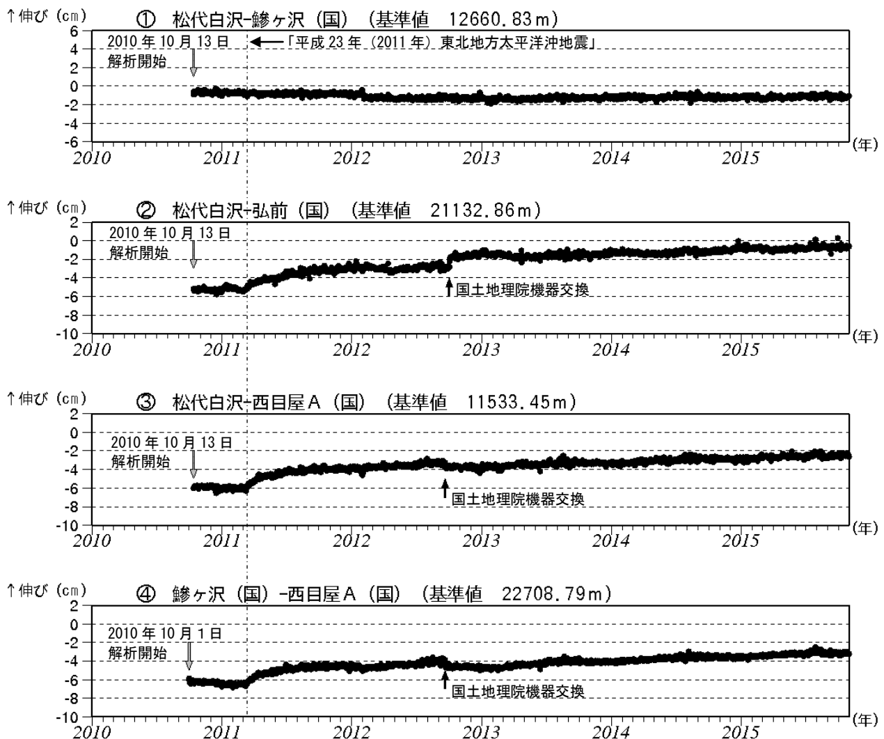
図3 岩木山 GNSS 1) 基線長変化図（2010年10月～2015年10月）
