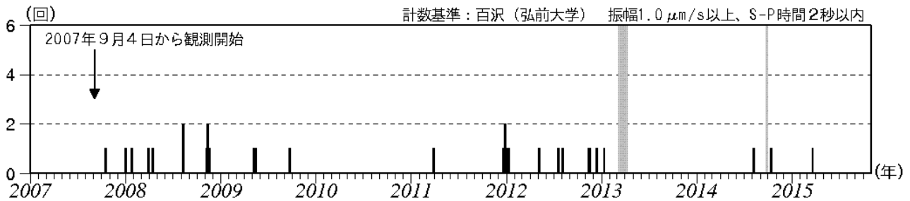
図2 岩木山 日別地震回数（2007年9月～2015年10月）
