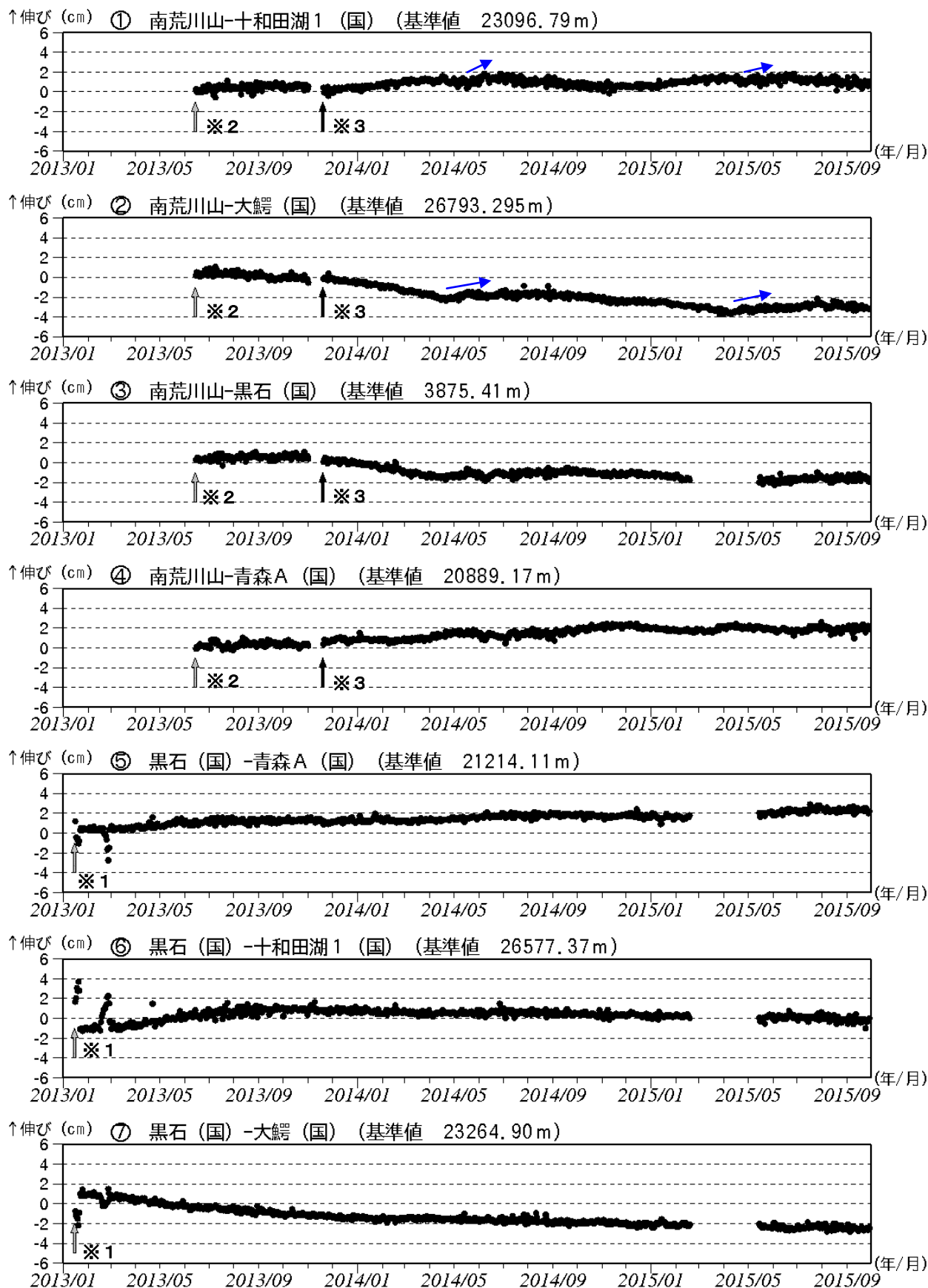
図3-① 八甲田山 GNSS 基線長変化図 (2013 年 1 月～2015 年 9 月)
