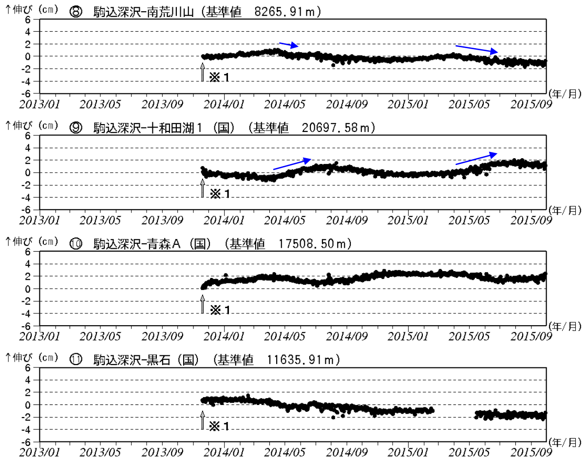
図3-② 八甲田山 GNSS 基線長変化図 (2013 年 1 月～2015 年 9 月)
