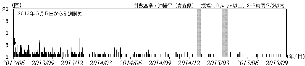
図2 八甲田山 日別地震回数 (2013年6月~2015年9月)
