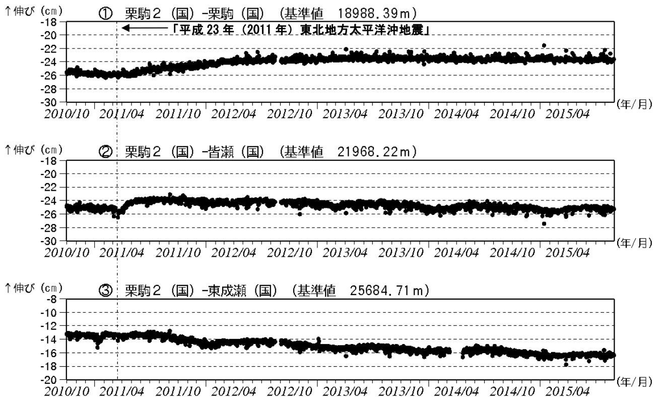
図5 栗駒山 GNSS 1) 基線長変化図（2010 年 10 月～2015 年 8 月）
