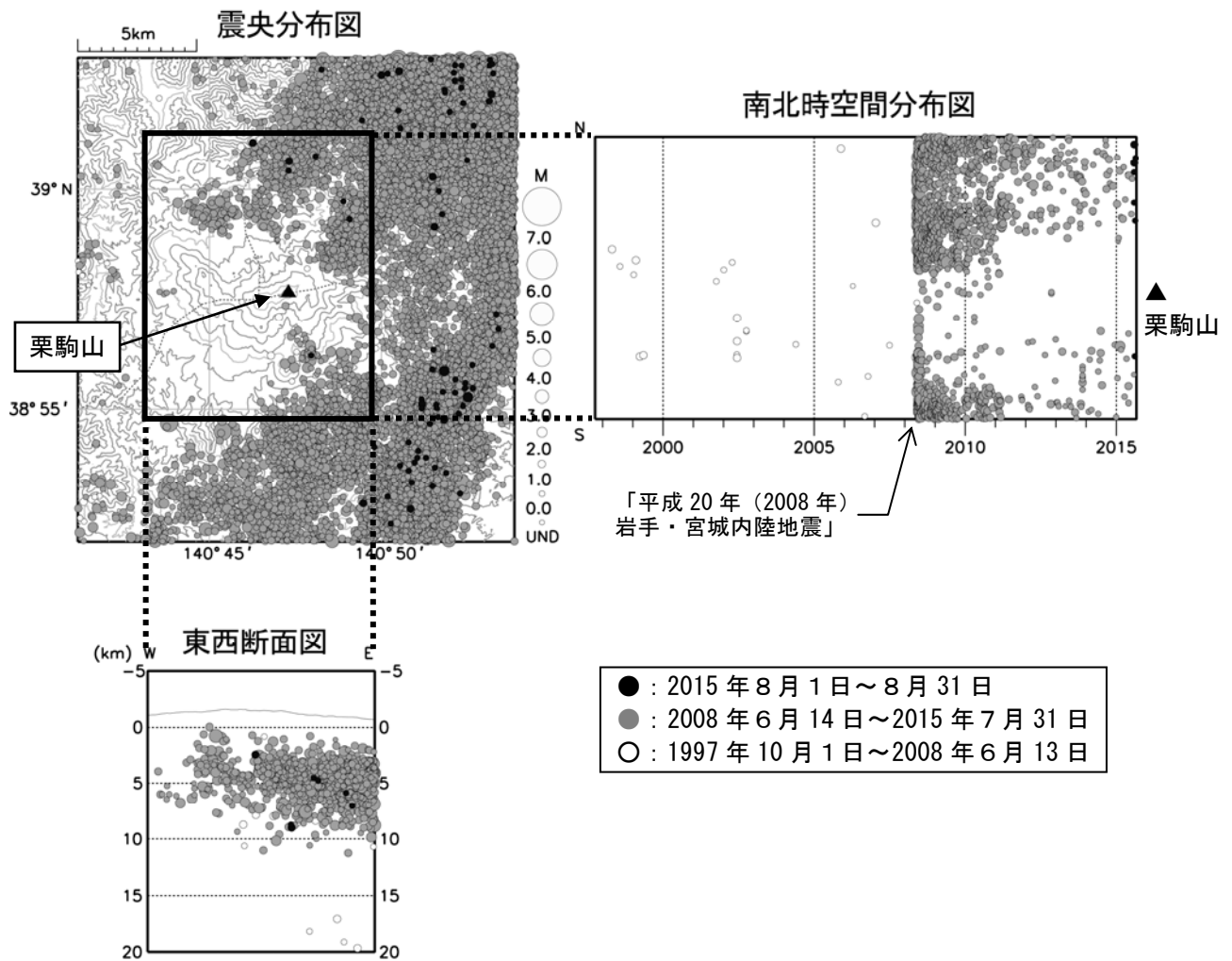
図 4 栗駒山 広域地震観測網による栗駒山周辺の地震活動（1997 年 10 月～2015 年 8 月）
