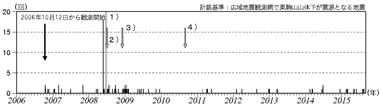
図3 栗駒山 日別地震回数（2006年10月～2015年8月）
