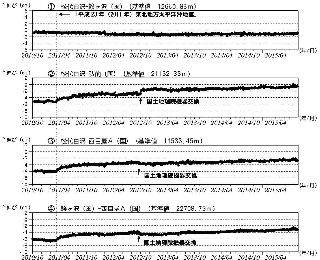
図3 岩木山 GNSS 1) 基線長変化図（2010年10月～2015年8月）
