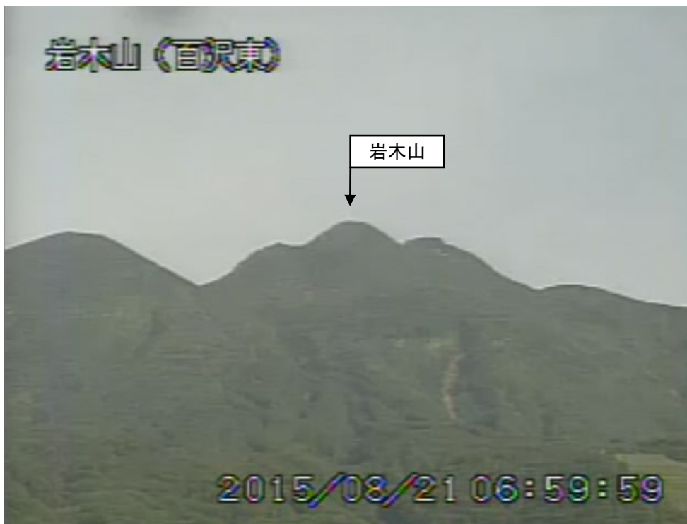
図 1 岩木山 山頂部の状況（8 月 21 日）
