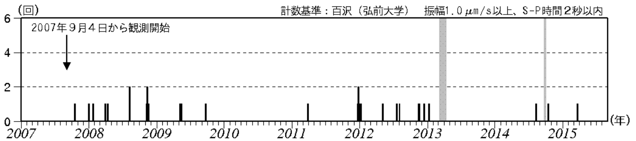
図2 岩木山 日別地震回数（2007年9月～2015年8月）
