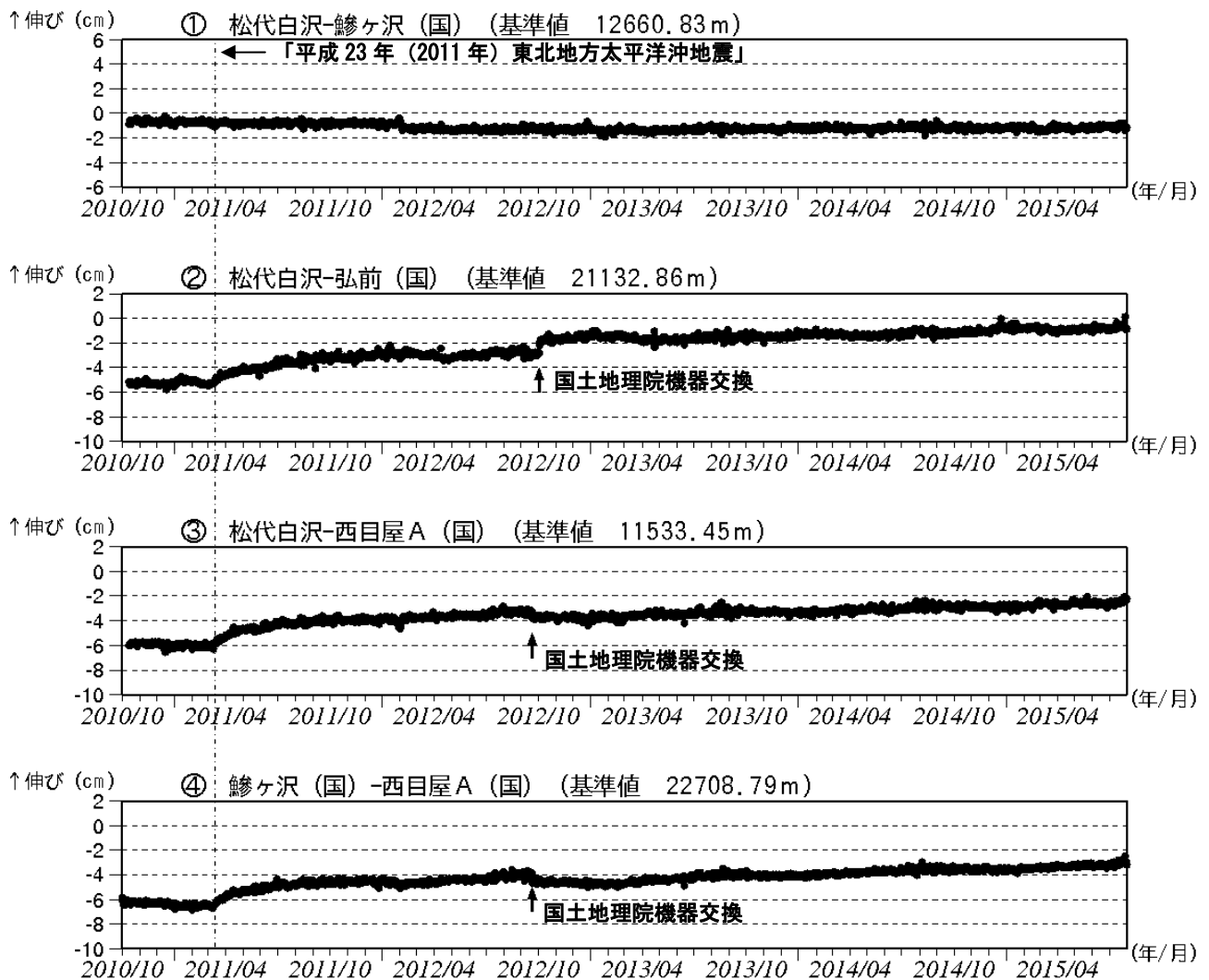
図3 岩木山 GNSS 1) 基線長変化図（2010年10月～2015年7月）
