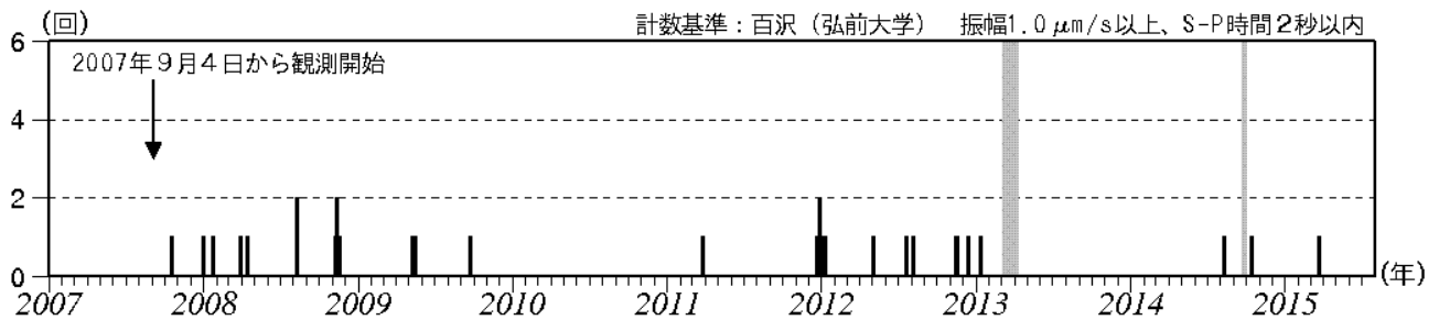
図2 岩木山 日別地震回数（2007年9月～2015年7月）
